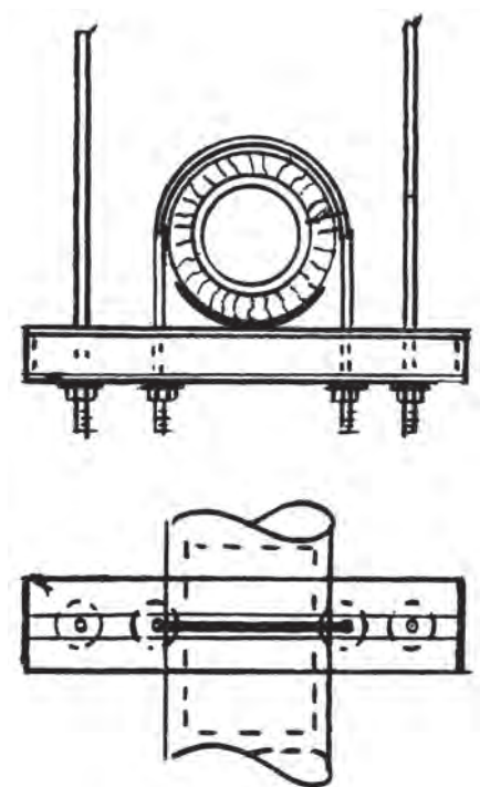
Σχήμα 1.7: Σχεδίαση λεπτομέρειας στήριξης σωλήνα με μόνωση.
