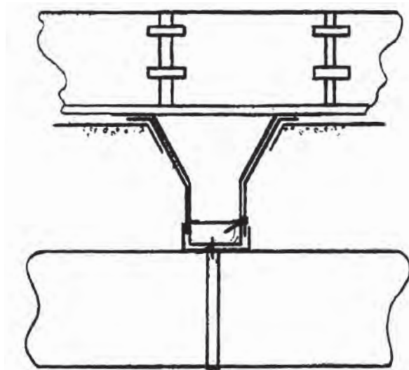
Σχήμα 3.19: Σχεδίαση υποστηρίγματος για αεραγωγό σε οροφή κτιρίου.
