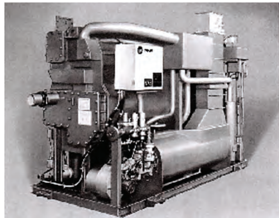
Σχήμα 5.12: Διβάθμιος ψύκτης νερού έμμεσης θέρμανσης (πηγή: Trane)
