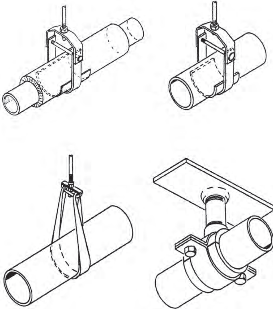
Σχήμα 1.13: Τριδιάστατη απεικόνιση διάφορων ειδών στήριξης σωληνώσεων από την οροφή.
