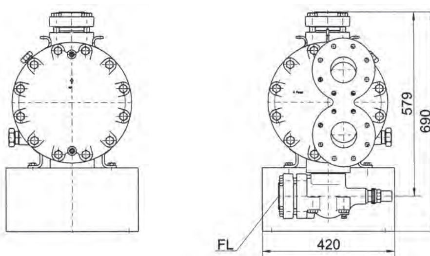
Σχήμα 4.8γ: Αριστερή και δεξιά πλάγια όψη συμπυκνωτή κελύφους-αυλών (πηγή: Bitzer)
