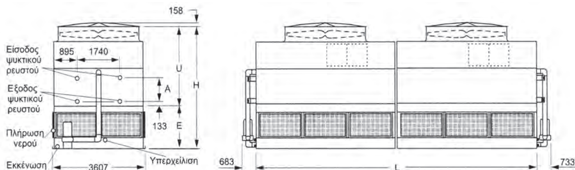
Σχήμα 4.15: Πρόσψη και πλάγια όψη αερόψυκτου συμπυκνωτή τύπου εξάτμισης (πηγή: Enarco)
