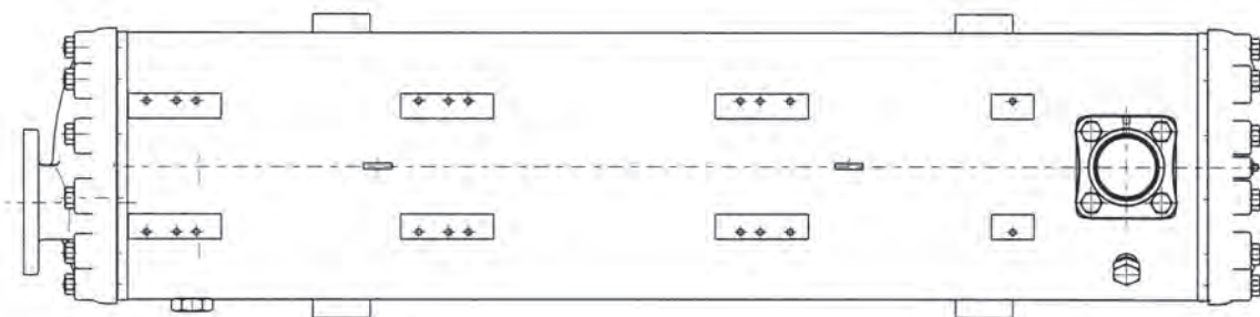
Σχήμα 4.8β: Κάτοψη συμπυκνωτή κελύφους-αυλών (πηγή:Bitzer)
