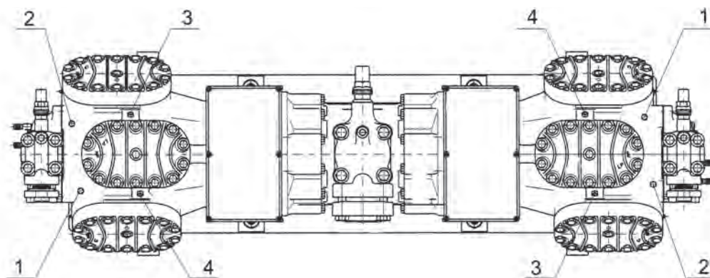
Σχήμα 4.4γ: Κάτοψη διάταξης ημερημτικών παλινδρομικών συμπιεστών συνδεδεμένων μεταξύ τους (πηγή:Bitzer)
