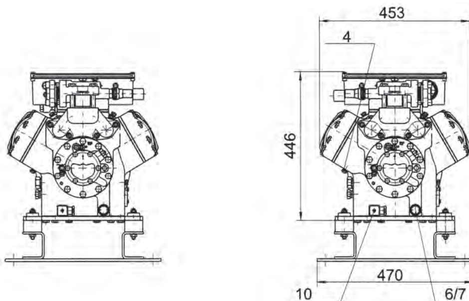
Σχήμα 4.4β: Αριστερή και δεξιά πλάγια όψη διάταξης ημερημνητικών παλινδρομικών συμπιεστών συνδεδεμένων μεταξύ τους (πηγή:Bitzer)
