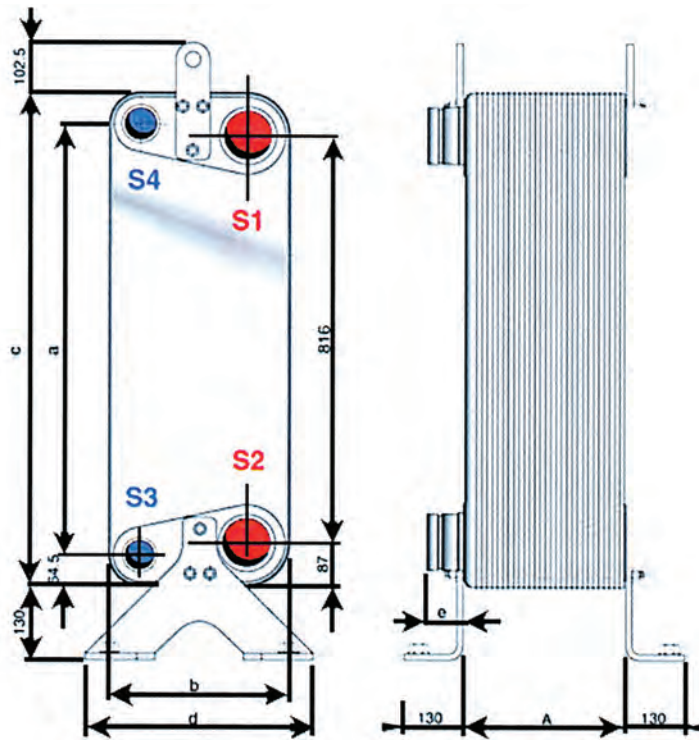
Σχήμα 4.19: Πρόοψη και δεξιά όψη του εξατμιστή με κασιτεροκολλημένες πλάκες (πηγή: Alfa Laval)
