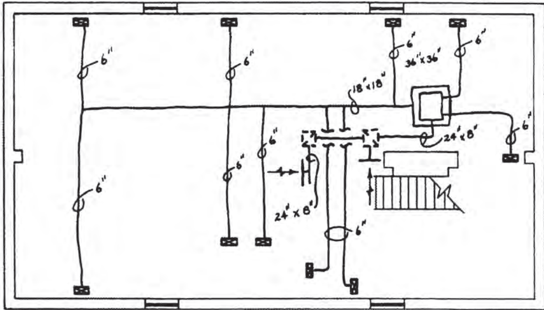
Σχήμα 3.40: Σχέδιο άσκησης 3.9.1
