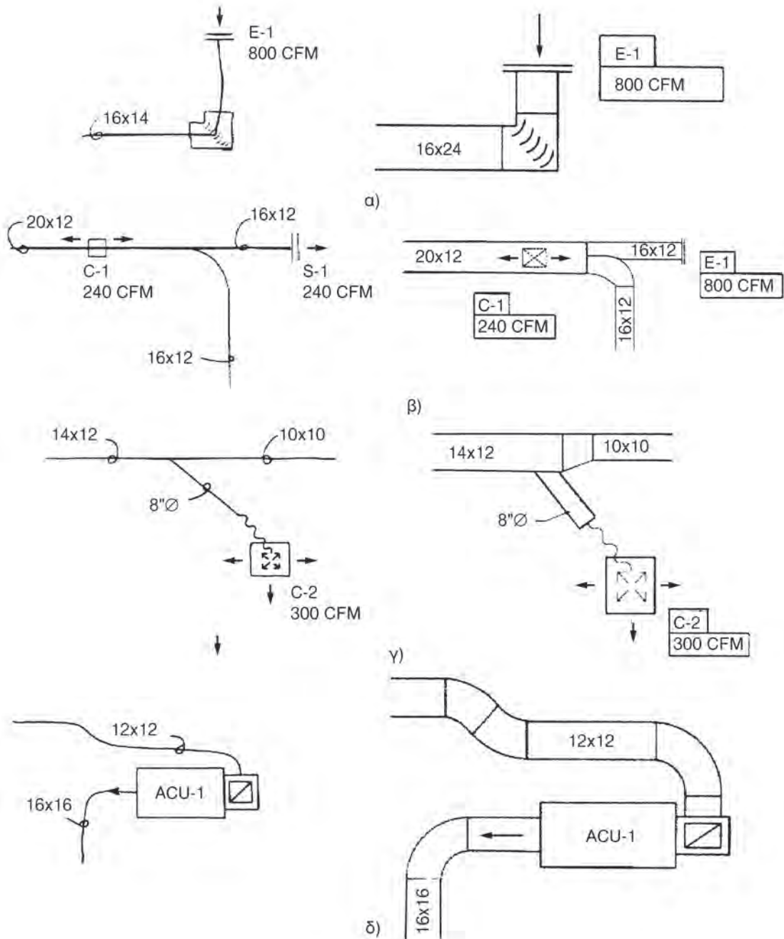
Σχήμα 3.2: Παραδείγματα μετατροπής σχηματικής σχεδίασης σε παραστατική σχεδίαση.
