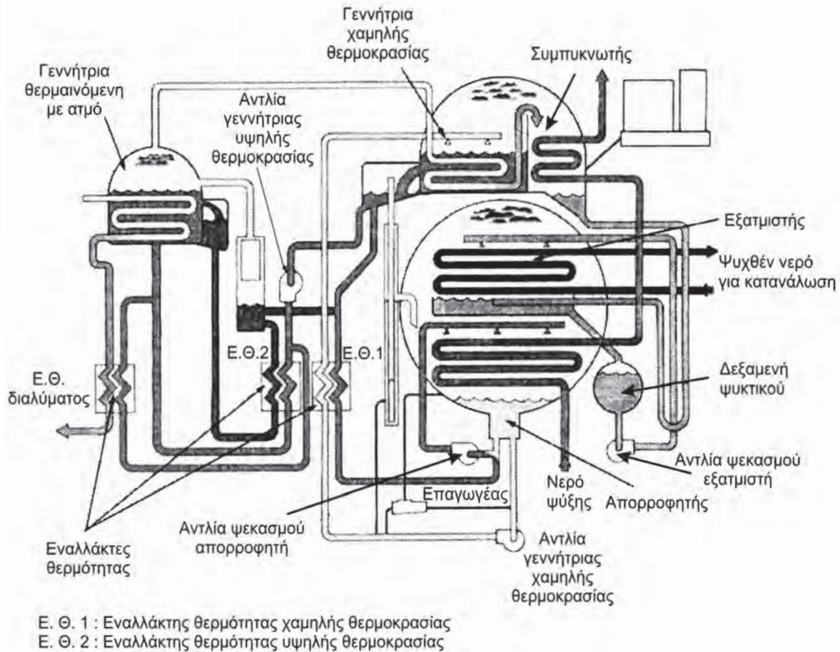
Σχήμα 5.8: Διβάθμιο ψύκτης νερού έμμεσης θέρμανσης (πηγή: Trane)
