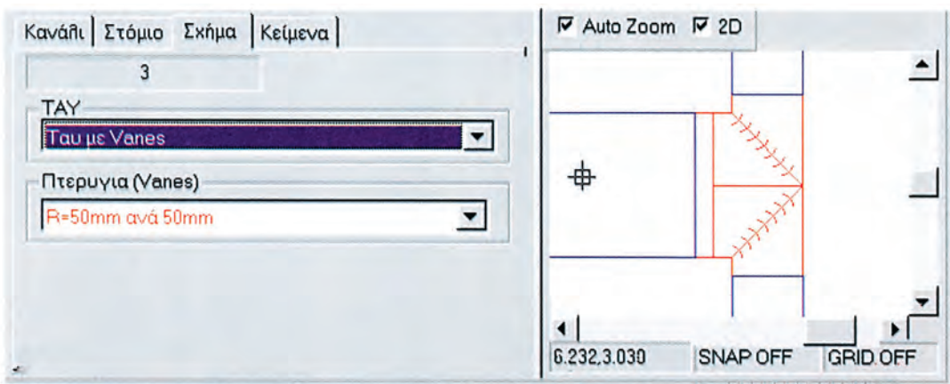
Σχήμα 8.31: Ταυ με πτερύγιο αλλαγής διεύθυνσης
