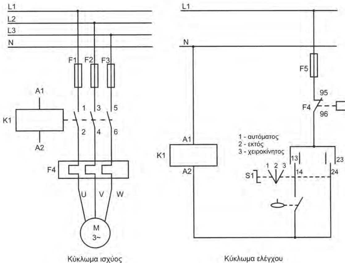
Σχήμα 7.19: Κύκλωμα εκκίνησης - στάσης τριφασικού κινητήρα με δυνατότητα επιλογής αυτόματης ή χειροκίνητης λειτουργίας
