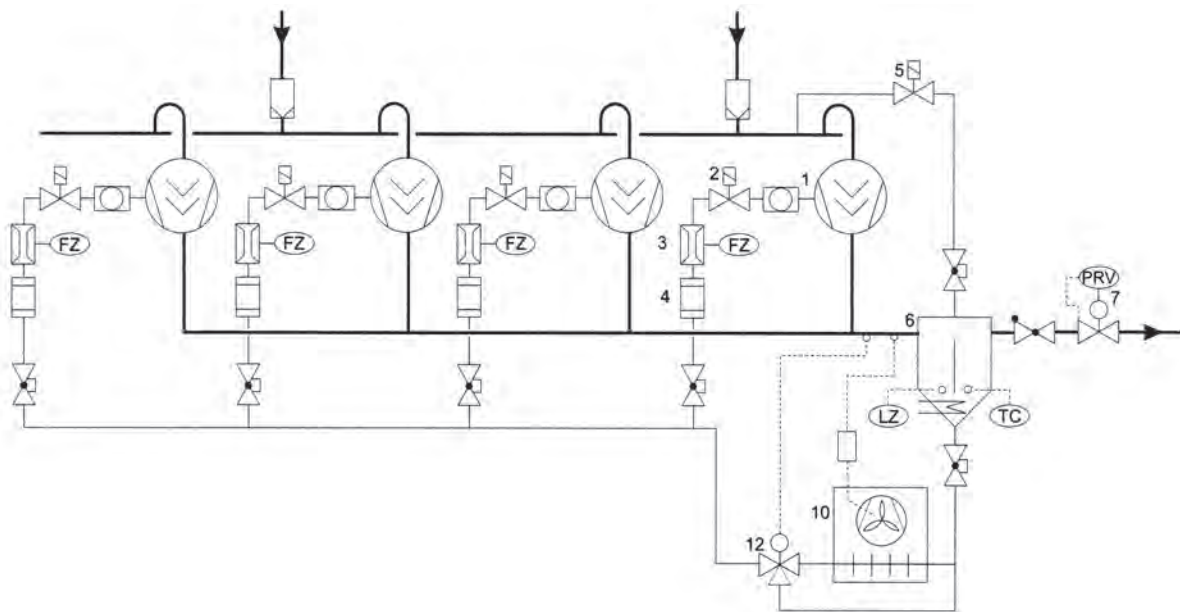
Σχήμα 4.31: Διάγραμμα ψυκτικής εγκατάστασης (πηγή: Bitzer)
