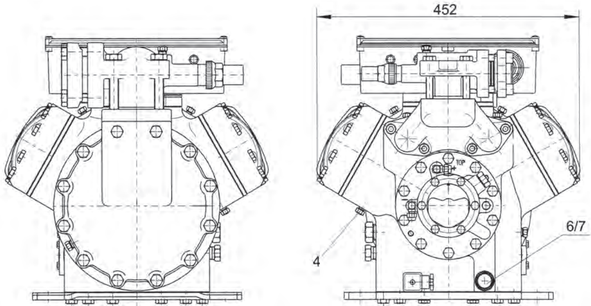
Σχήμα 4.3β: Δεξιά και αριστερή πλάγια όψη ημερημτικού παλινδρομικού συμπιεστή (πηγή:Bitzer)
