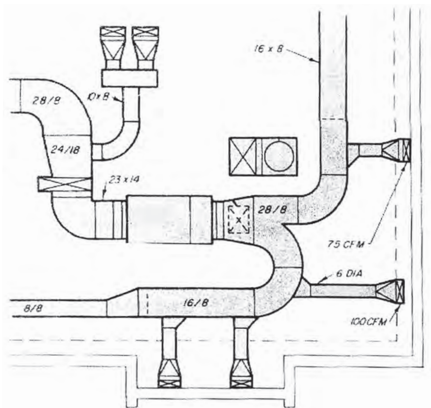
Σχήμα 3.31: Σχεδίαση συστήματος αεραγωγών.
