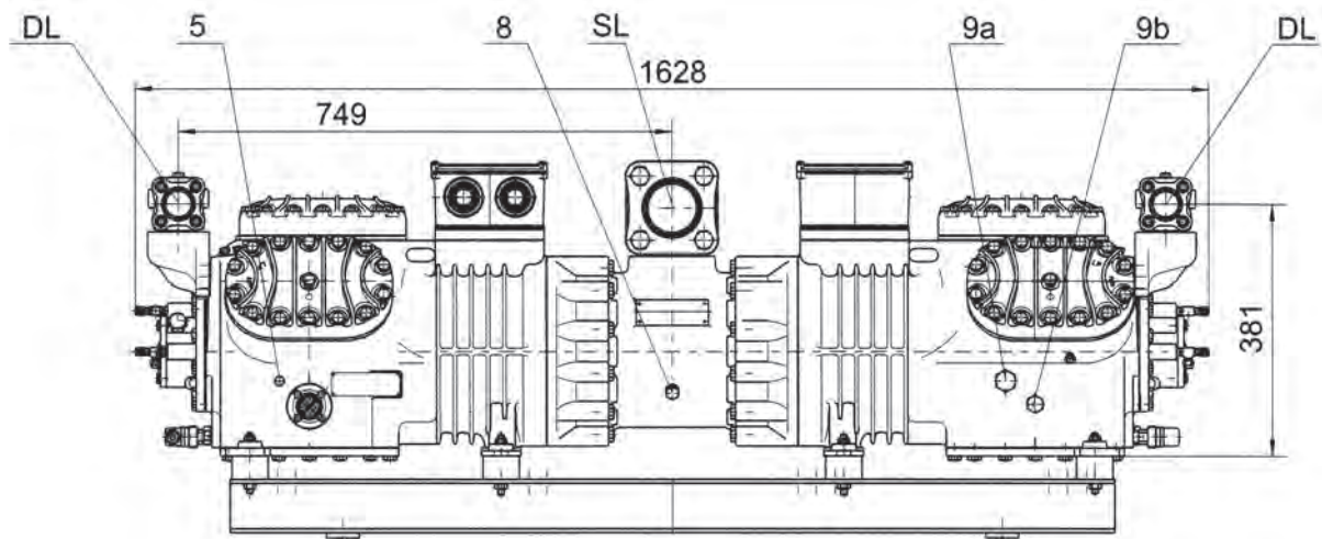
Σχήμα 4.4α: Πρόοψη διάταξης ημερημνητικών παλινδρομικών συμπιεστών συνδεδεμένων μεταξύ τους (πηγή:Bitzer)
