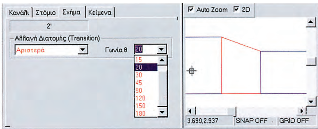
Σχήμα 8.34: Συστολή αριστερή με γωνία 20°
