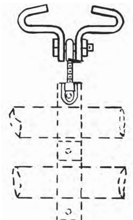
Σχήμα 1.8: Σχεδίαση λεπτομέρειας στήριξης σωλήνα με “τανιστήρα”.
