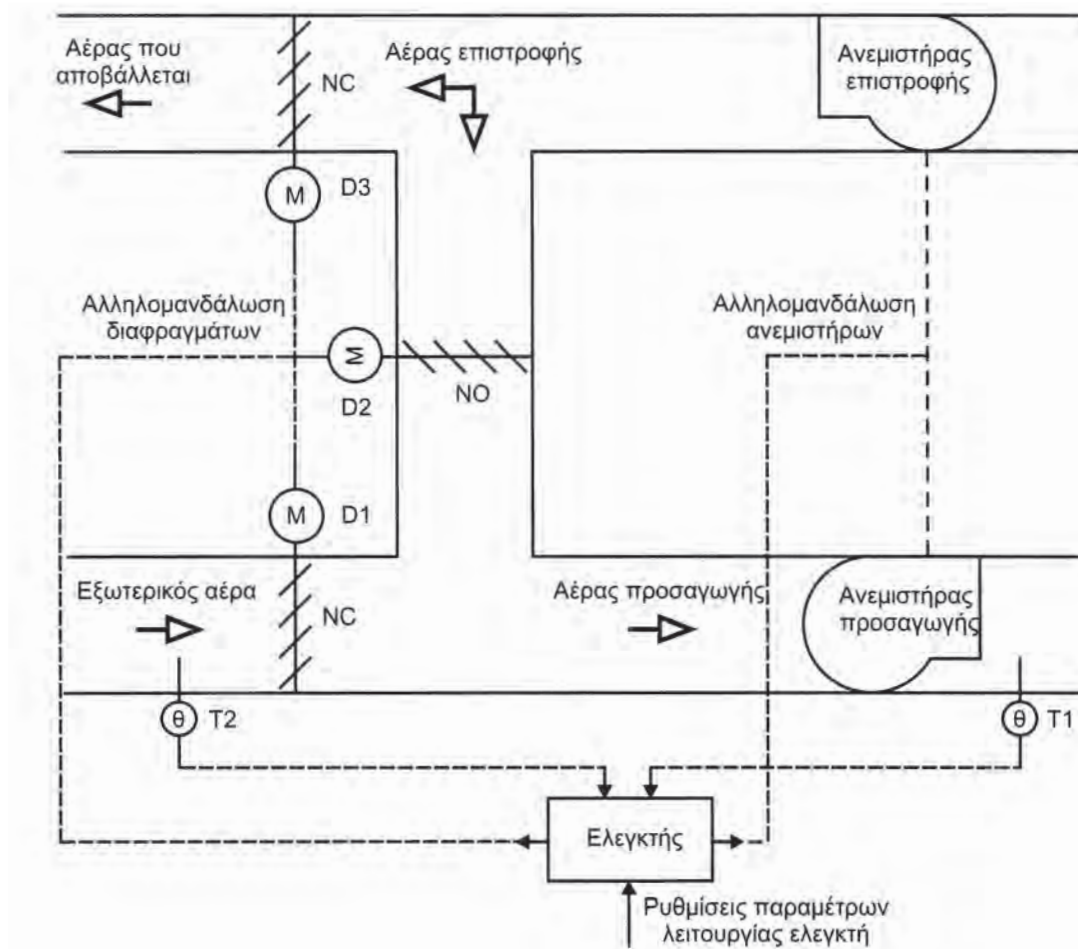
Σχήμα 7.13: Διάγραμμα συστήματος αυτόματου ελέγχου της θερμοκρασίας του αέρα προσαγωγής αεραγωγού
