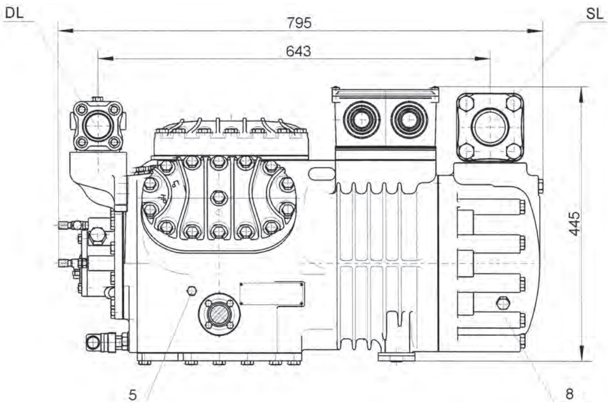
Σχήμα 4.3α: Πρόοψη ημερημνητικού παλινδρομικού συμπιεστή (πηγή: Bitzer)
