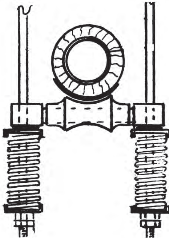
Σχήμα 1.6: Σχεδίαση λεπτομέρειας στήριξης σωλήνα με ελατήρια.
