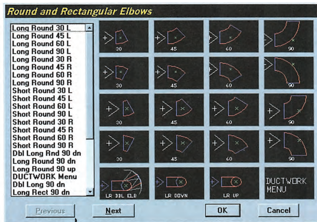
Σχήμα 8.12: Βιβλιοθήκη εξαρτημάτων
