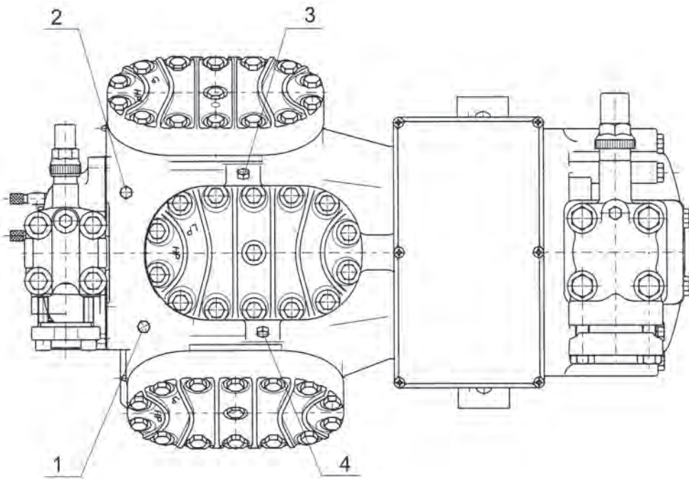
Σχήμα 4.3γ: Κάτοψη ημερημτικού παλινδρομικού συμπιεστή (πηγή:Bitzer)
