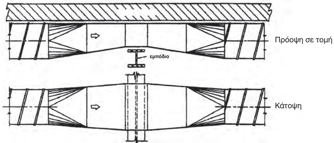
Σχήμα 2.9: Σχεδίαση αλλαγής διατομής αεραγωγού από ορθογωνική σε κυκλική, για την αποφυγή εμπόδιου.
