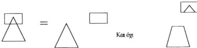
Σχηματική αναπαράσταση της αρχής της απλότητας
