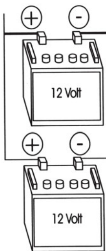
Σχήμα 3στ. Μπαταρίες σε παράλληλη σύνδεση
