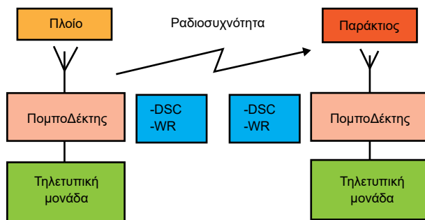
Σχήμα 7γ. Ραδιοτηλετυπικός εξοπλισμός με κλήσεις DSC.
