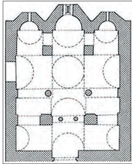
Κάτοψη με κόγχες προθέσεως, ιερού και διακονικού.
