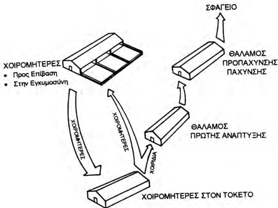
Εικόνα 3-20. Δομή κτιρίων χοιροστασίου αναπαραγωγής και πάχυνσης.
