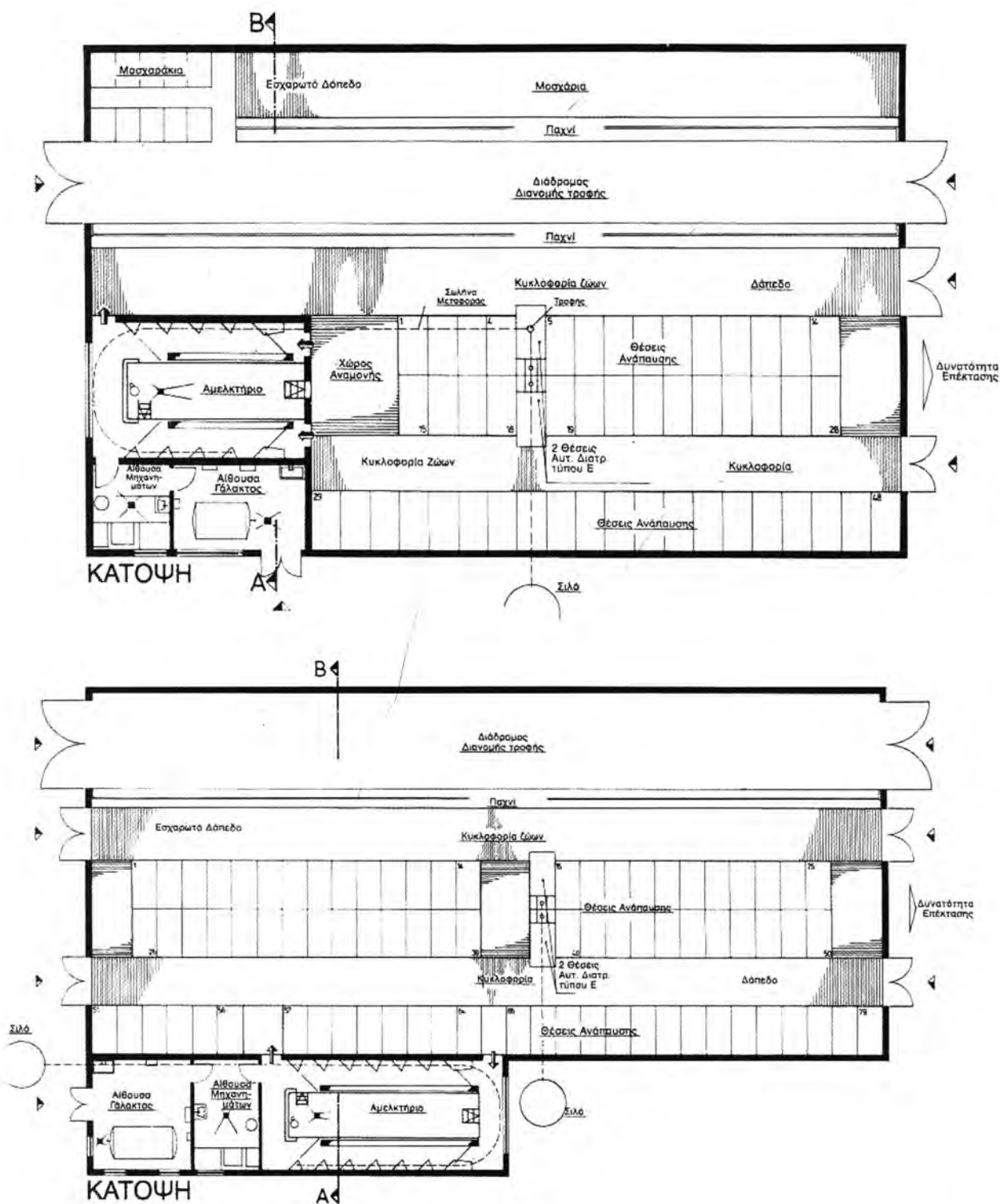
Εικόνα 1-37. Σχέδια σταύλων με ελεύθερο σταβλισμό, θέσεις ανάπαυσης για 50 ή 80 αγελάδες και αρμεκτήριο ψαροκόκκαλο.
