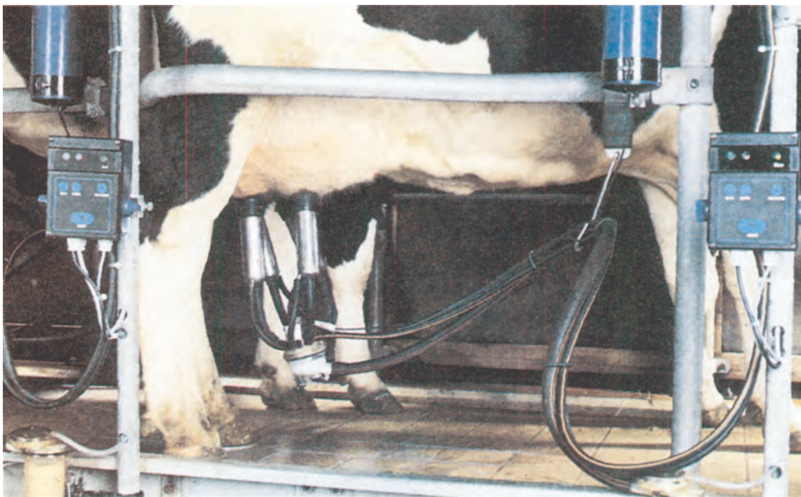
Εικόνα 1-20. Άρμεγμα με μηχανή
