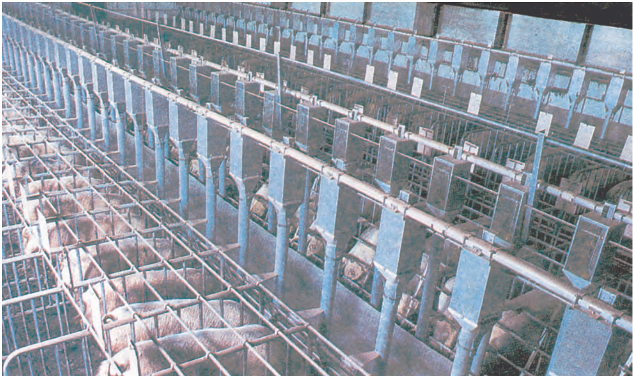
Εικόνα 3-15. Σύστημα αυτόματης, ατομικής διατροφής χοίρων.
