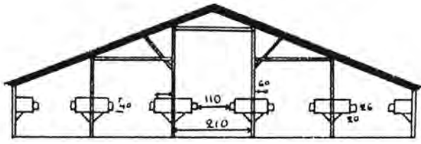
Εικόνα 7-7. Τομή υποστέγου με 10 σειρές κλωβών για μινκ.
