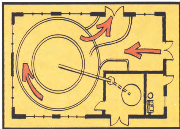
Εικόνα 2-35. Κάτοψη αρμεκτηρίου όπου φαίνεται η κίνηση των ζώων (είσοδος-έξοδος)
