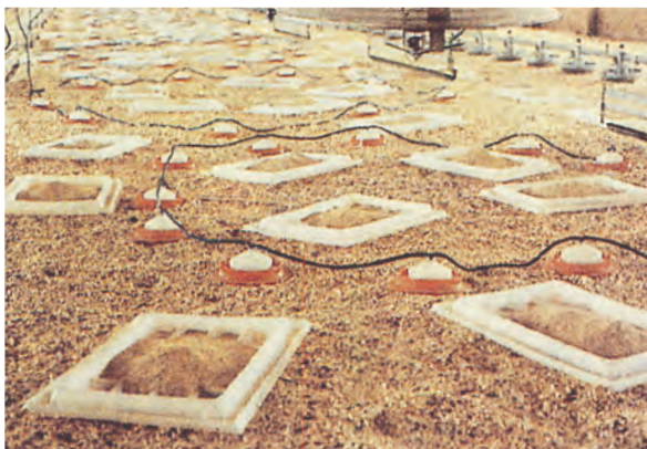
Εικόνα 5-49. Θάλαμος έτοιμος να δεχθεί νεοσσούς. Έχει ετοιμασθεί η στρωμνή, έχουν τοποθετηθεί οι ειδικές ποτίστρες-ταΐστρες. Διακρίνεται θερμομητέρα. Αλώνια δεν έχουν σχηματισθεί, γιατί προφανώς χρησιμοποιείται κεντρική θέρμανση.
