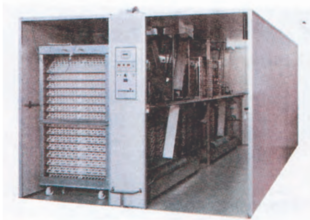
Εικόνα 5-22. α. Επωαστική μηχανή β. Εκκολαπτική μηχανή
