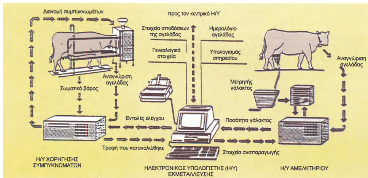
Εικόνα 6-13. Πλήρως αυτοματοποιημένο σύστημα συλλογής και επεξεργασίας στοιχείων σε σταύλο αγελάδων γαλακτοπαραγωγής
