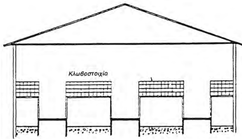
Εικόνα 6-7. Εγκάρσια τομή θαλάμου εκτροφής κουνελιών με 4 σειρές κλουβιών.
