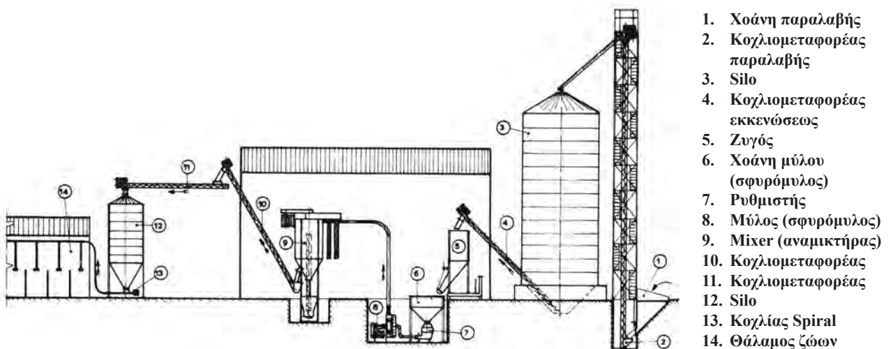
Εικόνα 10-31: Σχεδιάγραμμα μιας πλήρους αυτοματοποιημένης βιομηχανίας ζωοτροφών με τα επιμέρους μηχανήματα.
