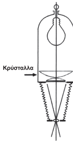
Εικόνα 5.3.2: Μεγεθυντήρας συγκεντρωτικός
