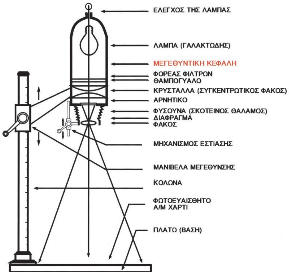
Εικόνα 5.1: Σχέδιο μεγεθυντήρα
