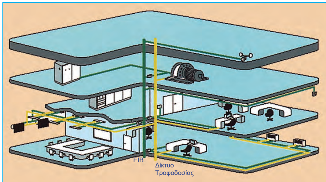
Σχήμα 1.4: Εγκατάσταση κτιρίου
