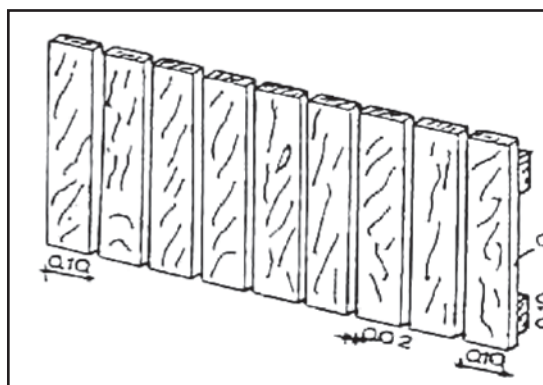
Εικόνα 13.48: Κουρτίνα και ανεμοφράκτης για περιορισμό της ταχύτητας του αέρα και λεπτομέρεια κατασκευής του
