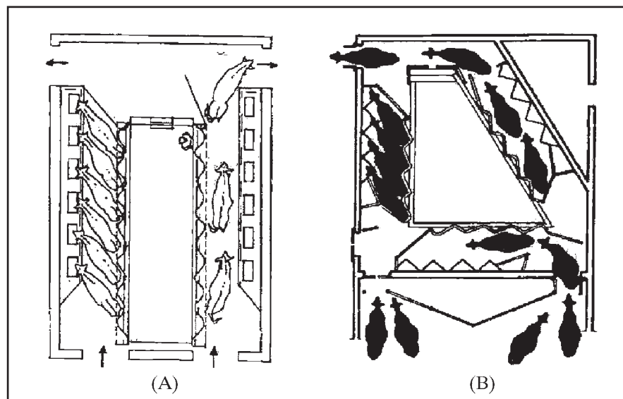
Εικόνα 6.73: Α: Διάγραμμα αρμεκτηρίου τύπου ψαροκόκαλου 2X6 και Β: Διάγραμμα τριγωνικού αρμεκτηρίου τύπου 3X4
