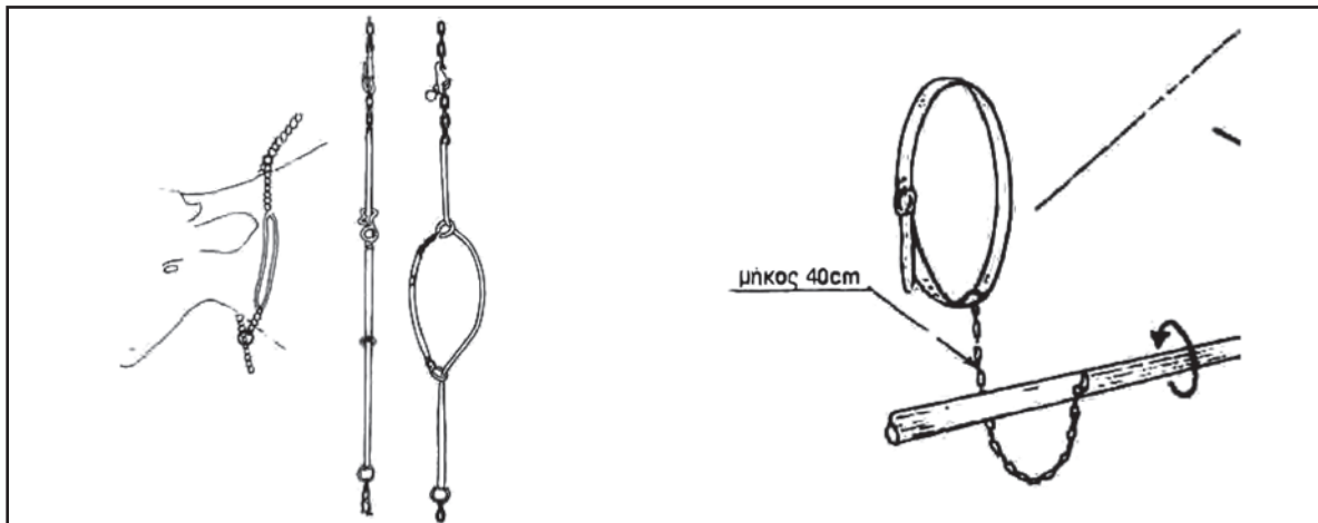
Εικόνα 6.59: Ολλανδικός (αριστερά) και Καναδικός (δεξιά) τύπος πρόσδεσης αγελάδων στα συστήματα περιορισμένου σταβλισμού
