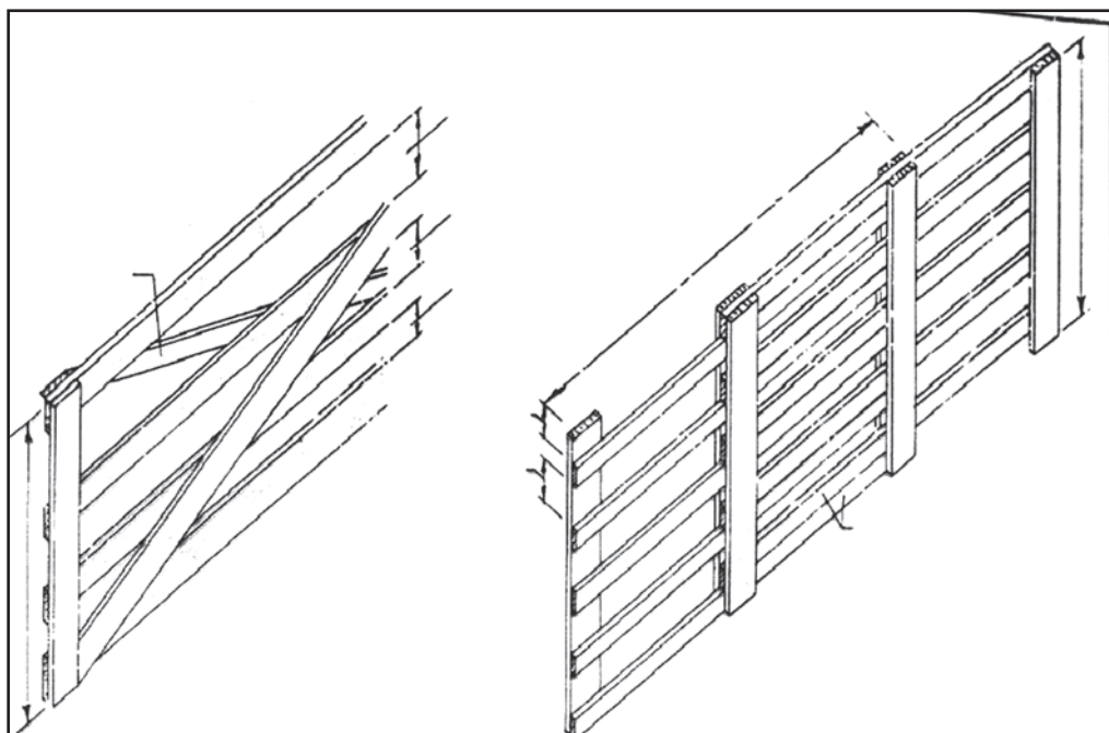
Εικόνα 13.50: Κινητά ξύλινα χωρίσματα από σανίδες (σταθερού και μεταβαλλόμενου μήκους) τον προσωρινό διαχωρισμό των διαφόρων κατηγοριών των ζώων ανάλογα με τις ανάγκες
