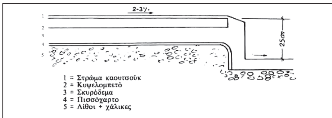
Εικόνα 6.56: Τομή ιδανικού δαπέδου της θέσης ανάπαυσης
