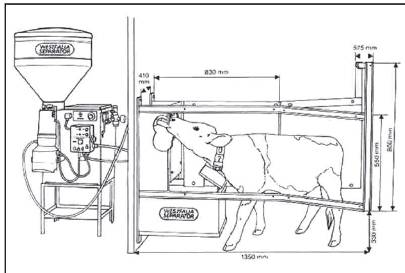
Εικόνα 7.6: Σχέδιο με κατασκευαστικά στοιχεία της θέσης τεχνητού θηλασμού που διαθέτουν οι θηλαστικές μονάδες ηλεκτρονικού τύπου
