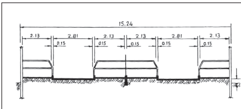
Εικόνα 6.64: Τομή χώρου ανάπαυσης ελεύθερου σταβλισμού με 4 σειρές θέσεων ανάπαυσης και δύο διαδρόμους κυκλοφορίας
