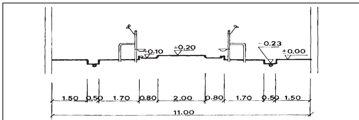
Εικόνα 6.57: Τομή στάβλου περιορισμένου σταβλισμού με 2 σειρές θέσεων στην οποία διακρίνονται με σειρά από αριστερά προς τα δεξιά: διάδρομος κυκλοφορίας, κανάλι συλλογής αποβλήτων, θέση ανάπαυσης, ταϊστρα, διάδρομος τροφοδοσίας, ταϊστρα, θέση ανάπαυσης, κανάλι συλλογής αποβλήτων, διάδρομος κυκλοφορίας
