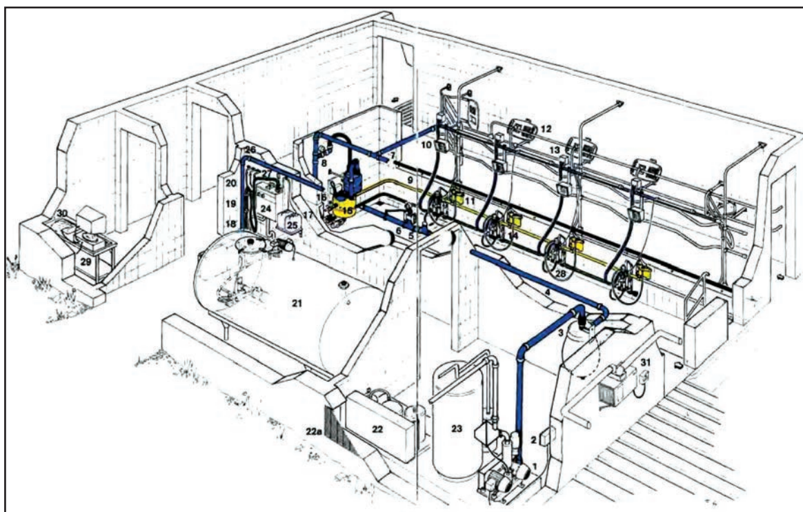
Εικόνα 6.49: Αρμεκτήριο τύπου ψαροκόκαλου
