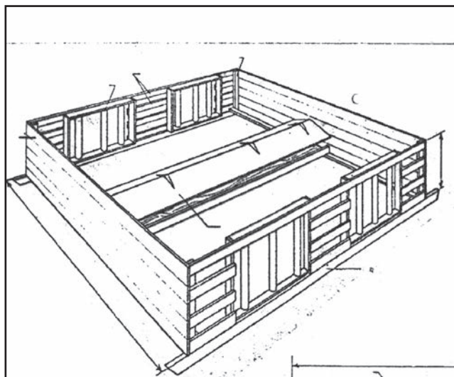
Εικόνα 13.52: Κινητά χωρίσματα σχηματίζοντα ιδιαίτερους χώρους για την περιοδική απομόνωση των θηλαζόντων αρνιών και εριφίων με αυτόματη ταΐστρα
