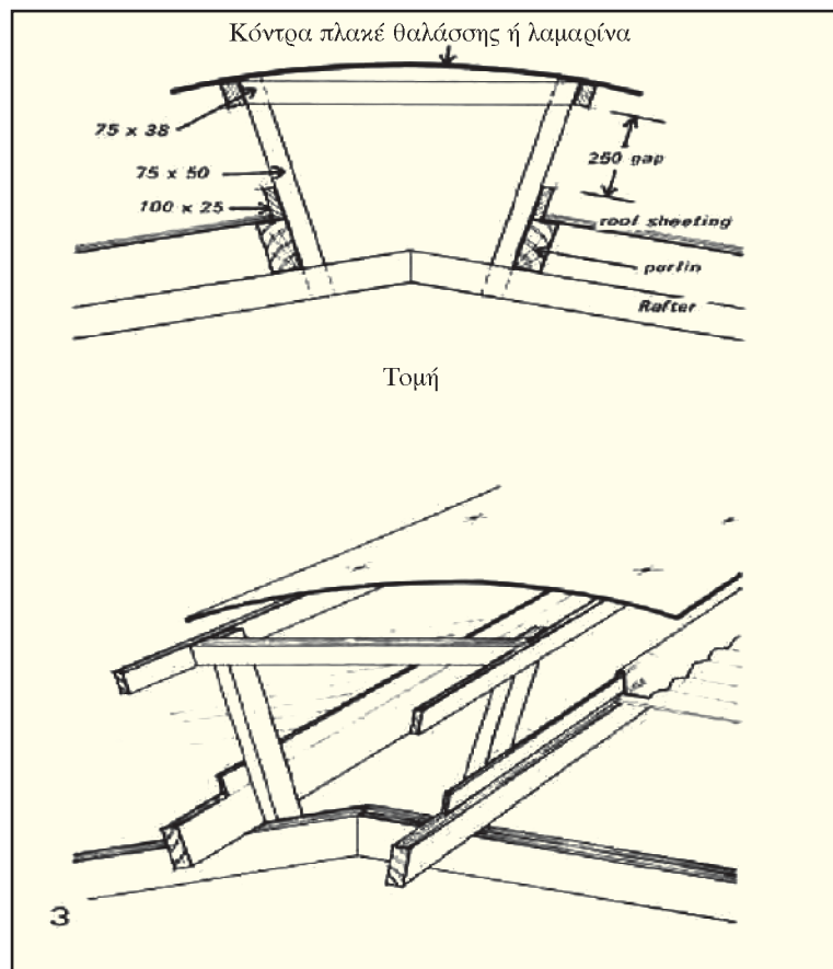
Εικόνα 13.49: Λεπτομέρεια κατασκευής κεντρικού συνεχούς ανοίγματος δίρικτης στέγης απαραίτητου για την απομάκρυνση του συγκεντρωμένου θερμού αέρα και των υδρατμών
