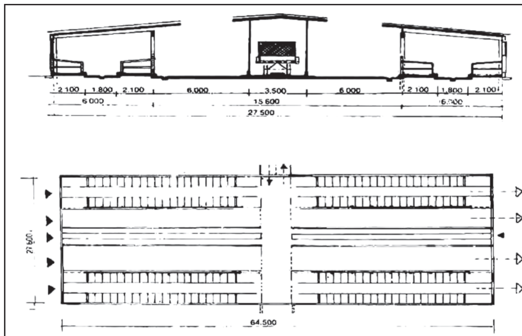
Εικόνα 6.69: Βουστάσιο ελεύθερου σταβλισμού 160 αγελάδων με 4 χώρους ανάπαυσης των 2 σειρών ο καθένας και χώρο διατροφής στο χώρο άσκησης (προαύλια)
