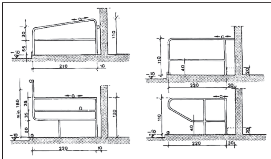
Εικόνα 6.62: Τύποι χωρισμάτων των ατομικών θέσεων ανάπαυσης στο σύστημα ελεύθερου σταβλισμού
