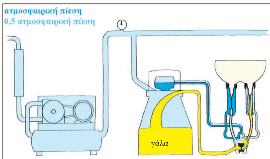
Εικόνα 6.47: Άρμεκτικό συγκρότημα με κάδους
