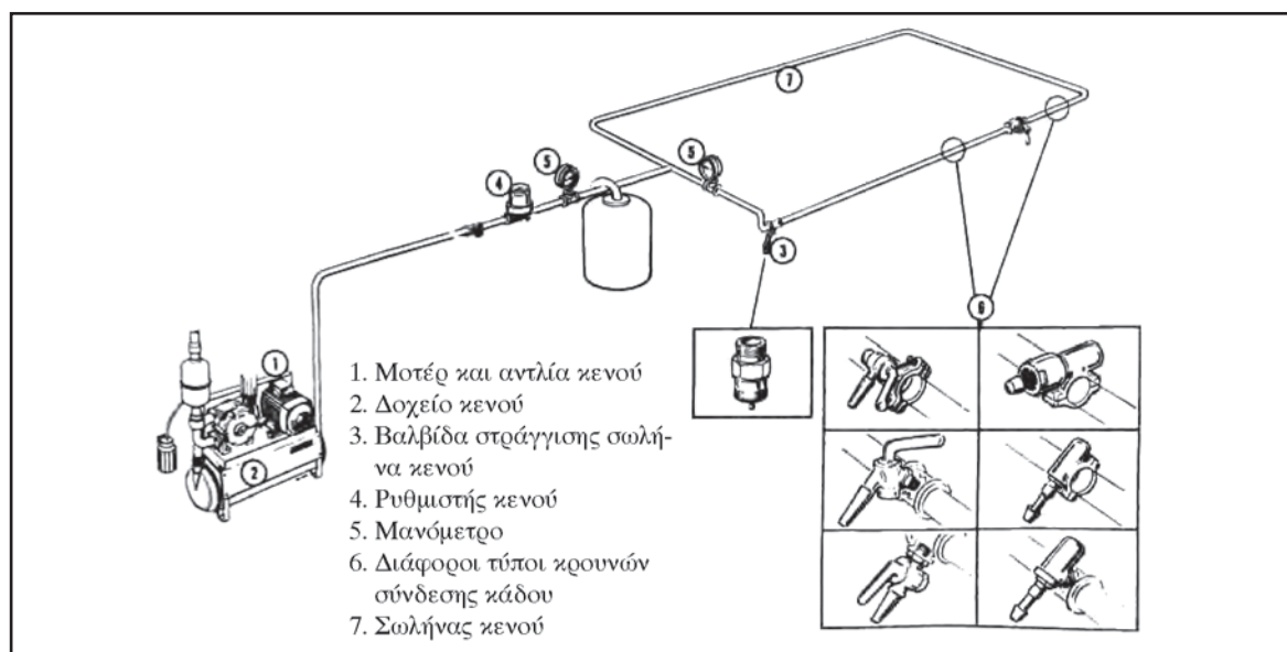
Εικόνα 6.42: Σχηματική παρουσίαση του συστήματος κενού αρμεκτικού συγκροτήματος
