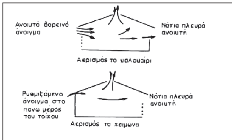
Εικόνα 13.47: Σχηματική τομή προβατοστασίου για επίδειξη του τρόπου φυσικού αερισμού το καλοκαίρι και το χειμώνα
