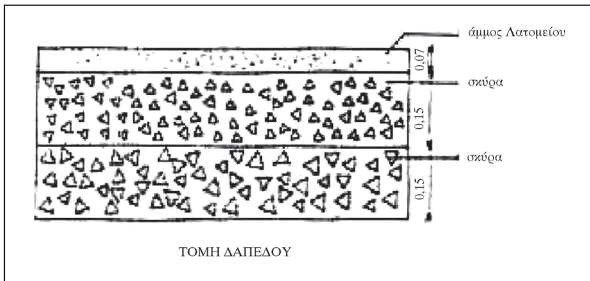
Εικόνα 13.43: Λεπτομέρεια κατασκευής τεχνητού εδάφους με τρεις στρώσεις (από πάνω προς τα κάτω: άμμος 5cm πάχος, χαλίκια διαμέτρου 2-3cm και πάχος 15cm, χαλίκια διαμέτρου 3-5cm και πάχος 15cm)
