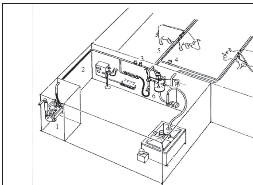
Εικόνα 6.48: Συγκρότημα με σωλήνα μεταφοράς γάλακτος
