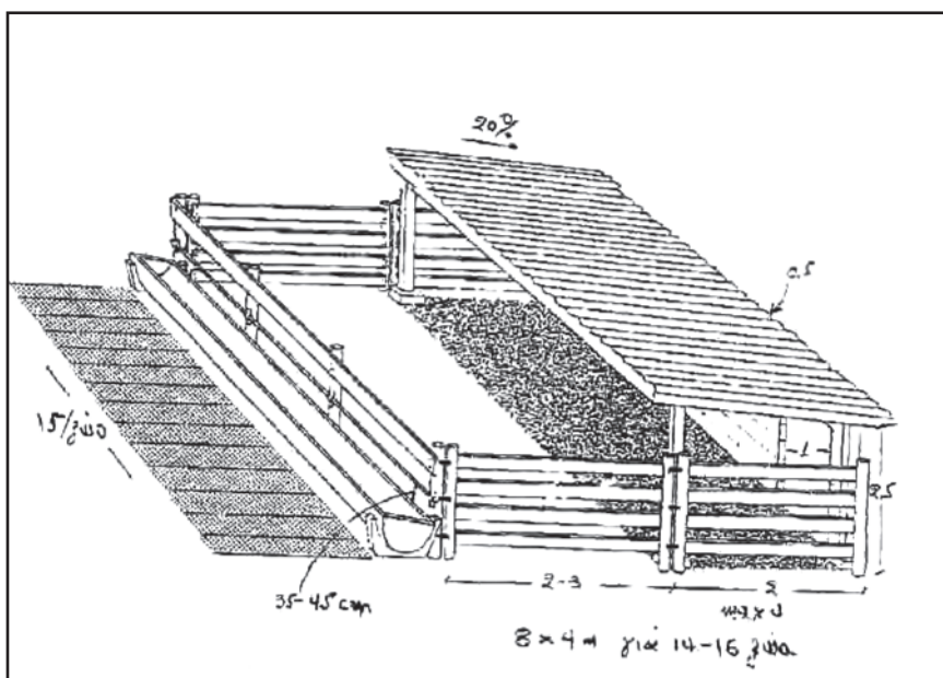
Εικόνα 7.17: Σχέδιο με κατασκευαστικά στοιχεία ανοικτού στάβλου παχυνόμενων μοσχαριών ελεύθερου σταβλισμού
