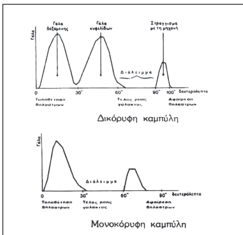
Εικόνα 13.30: Δικόρυφη και μονοκόρυφη καμπύλη απεικόνισης της ροής του γάλακτος ακολουθούμενη από την καμπύλη στράγγισης του γάλακτος
