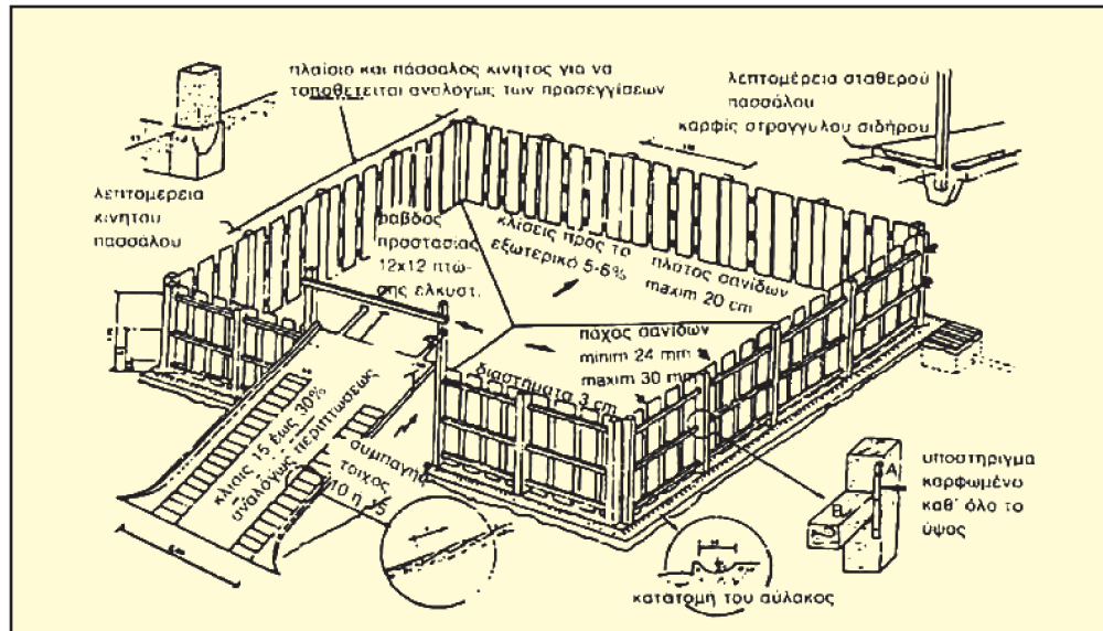
Εικόνα 6.78: Σχεδιάγραμμα κατασκευαστικών λεπτομερειών κοπροσωρού
