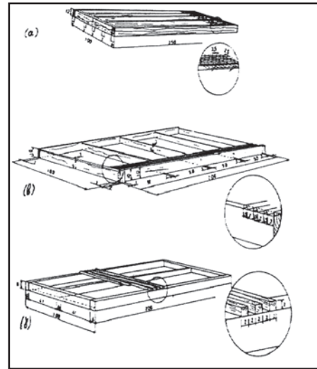
Εικόνα 13.46: Ξύλινο σχαρωτό δάπεδο και λεπτομέρεια κατασκευής του
