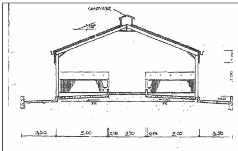
Εικόνα 7.15: Σχέδιο με κατασκευαστικά στοιχεία κλειστού στάβλου ελεύθερου σταβλισμού
