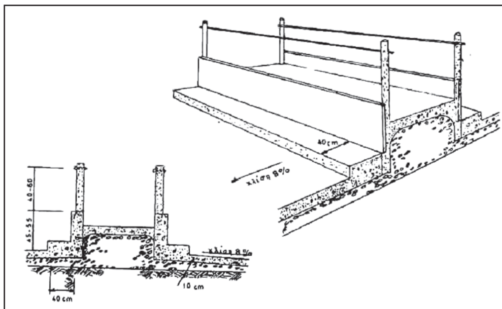
Εικόνα 6.68: Λεπτομέρεια κατασκευής ταΐστρας αγελάδων ελεύθερου σταβλισμού
