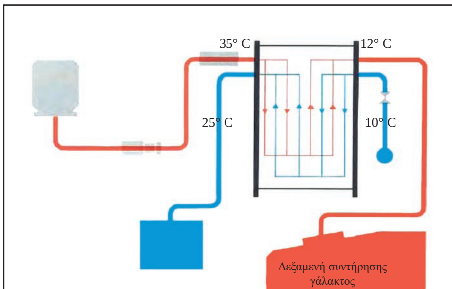
Εικόνα 6.54: Διάγραμμα λειτουργίας πλακοειδή ψύκτη συνεχούς λειτουργίας για άμεση ψύξη του γάλακτος, με αντίθετη ροή νερού αρχικής θερμοκρασίας 10°C και γάλακτος αρχικής θερμοκρασίας 35 °C
