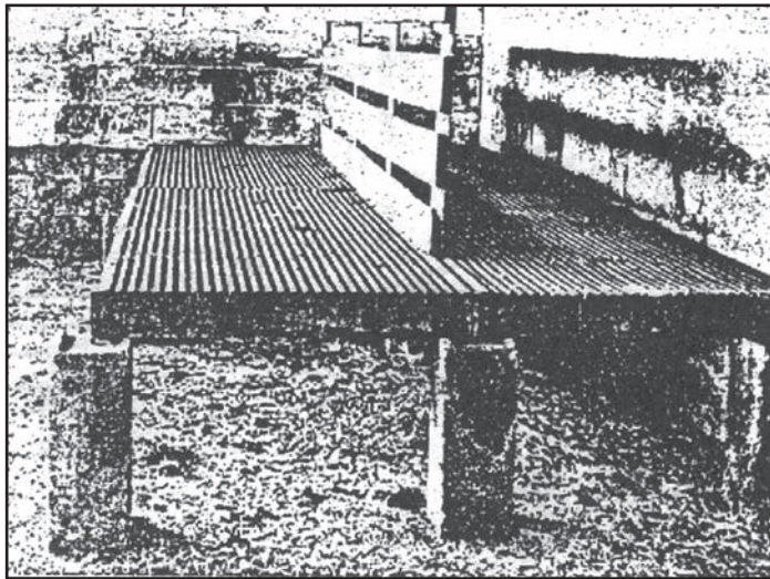
Εικόνα 13.46: Ξύλινο σχαρωτό δάπεδο και λεπτομέρεια κατασκευής του
