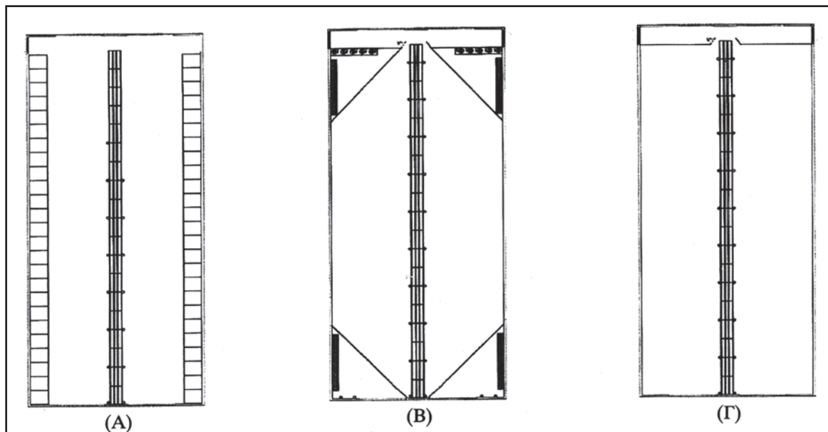
Εικόνα 13.56: Σχηματική λειτουργική κάτοψη αιγοπροβατοστασίου σε τρεις διαφορετικές περιόδους, με ταινία τροφοδοσίας στη μέση (Α: κατά την περίοδο των τοκετών εξοπλισμένο, με κελιά τοκετού Β: κατά την περίοδο του θηλασμού εξοπλισμένο με χώρους αρνιών ή εριφίων Γ: κατά την περίοδο της εγκυμοσύνης)
