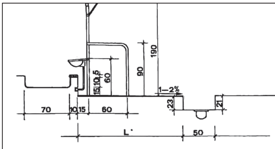
Εικόνα 6.61: Σχηματική τομή θέσης περιορισμένου σταβλισμού με 1 σειρά θέσεων, στην οποία διακρίνονται με σειρά από αριστερά προς τα δεξιά: διάδρομος τροφοδοσίας, ταΐστρα, θέση ανάπαυσης, κανάλι συλλογής αποβλήτων, διάδρομος κυκλοφορίας
