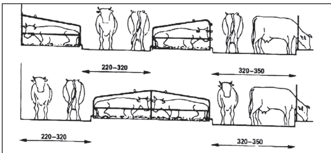
Εικόνα 6.63: Διάταξη διαδρόμων κυκλοφορίας και ατομικών θέσεων ανάπαυσης
