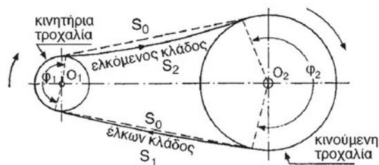
Σχήμα 14.6.2.δ Απλή περίπτωση ιμαντοκίνησης (πραγματική εικόνα, κατά την κίνηση)
