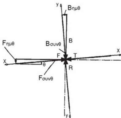
Σχήμα 14.6.3.γ Η ανάλυση των δυνάμεων που ενεργούν στο σπείρωμα κοχλίας, σε ορθογώνιο σύστημα x, x' - y, y' .
