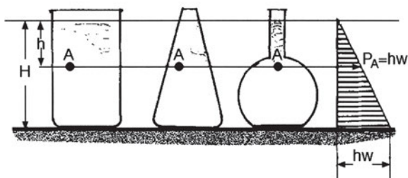
Σχήμα 15.4.δ Η υδροστατική πίεση είναι ανεξάρτητη από το σχήμα του δοχείου
