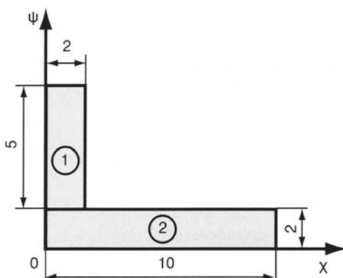
Σχήμα 4.α Σύνθετη επιφάνεια
