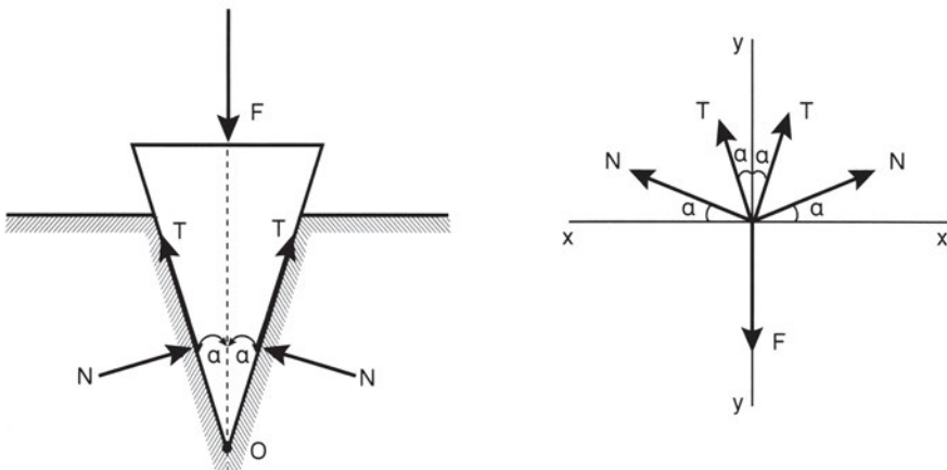
Σχήμα 13.5δ Ισοσκελής σφήνα
