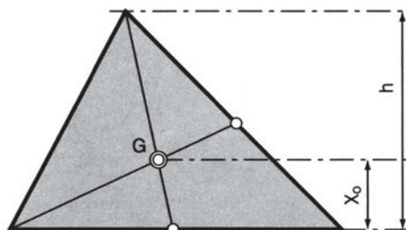
Σχήμα 4.3δ Κεντροειδές επιφάνειας τριγώνου
