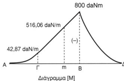
Σχήμα 8.6θ Μονοπροέχουσα δοκός
