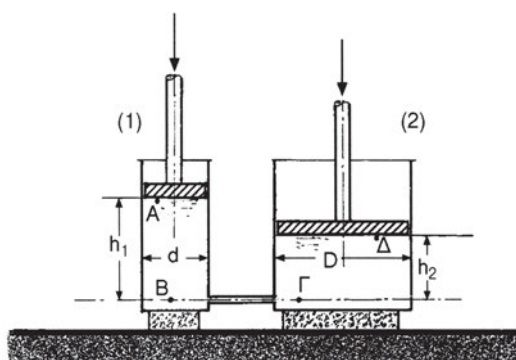
Σχήμα 15.9.1.α Η αρχή του υδραυλικού πιεστήριου - ανυψωτήρα
