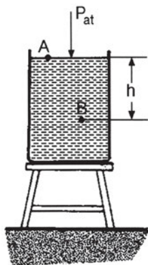
Σχήμα 15.4.γ Η πίεση υγρού σε ορισμένο βάθος
