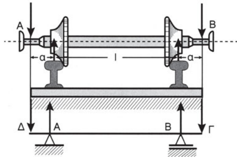
Σχήμα 8.2η Άρθρωση - Κύλιση
