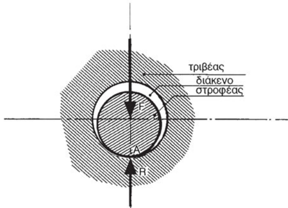
Σχήμα 14.6.1.γ Κατάσταση ηρεμίας
