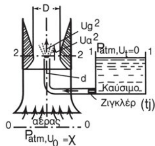
Σχήμα 16.8.β Εξαερωτής
