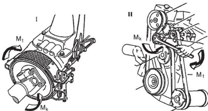
Σχήμα 11.1.α Περιπτώσεις εμφάνισης στρεπτικής καταπόνησης
