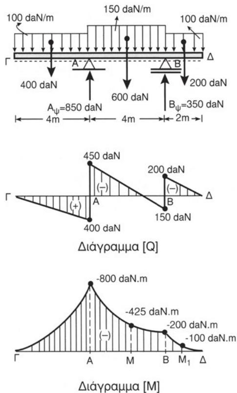
Σχήμα 8.6i Αμφιπροέχουσα δοκός
