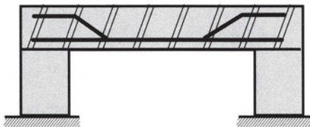
Σχήμα 10.45 Τοποθέτηση χάλυβα σε καμπτόμενη δοκό
