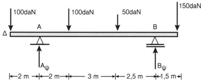
Σχήμα 8.3γ Αμφιπρόεχουσα δοκός
