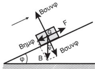
Σχήμα 13.2ε Το φορτίο ανέρχεται
