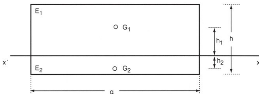
Σχήμα 7.3β Στατική ροπή ορθογωνικής διατομής
