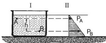
Σχήμα 15.4.α Η μεταβολή της υδροστατικής πίεσης μετά του βάθους
