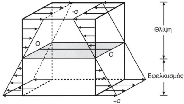
Σχήμα 8.50 Κάμψη της διατομής της δοκού
