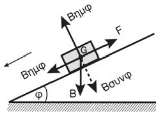
Σχήμα 13.25 Το φορτίο κατέρχεται
