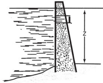
Σχήμα 16.4.α Δυναμική ενέργεια υγρού
