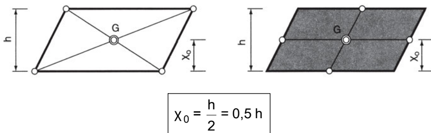
Σχήμα 4.3β Το κεντροειδές παραλληλογράμμου
