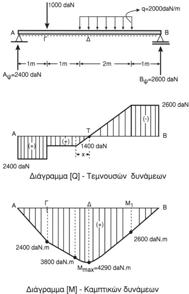
Σχήμα 10.4γ Καταπόνηση της δοκού σε κάμψη
