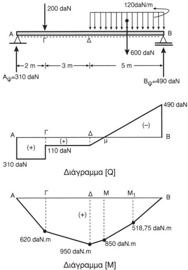
Σχήμα 8.6κ Αμφιέρεστη δοκός
