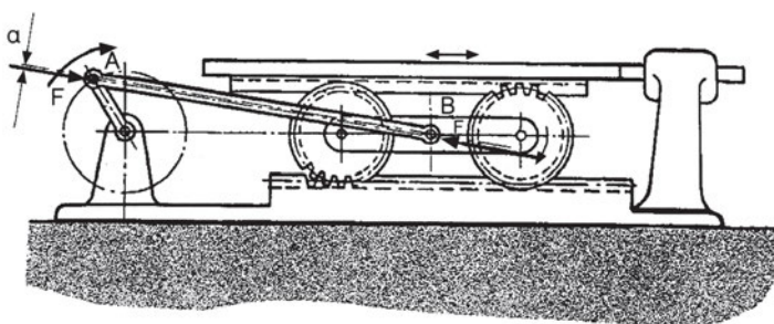
Σχήμα 12.3.3.α Στον μηχανισμό διωστήρα στροφάλου, το βάκτρο AB υπόκειται σε θλίψη και εφελκυσμό εναλλάξ
