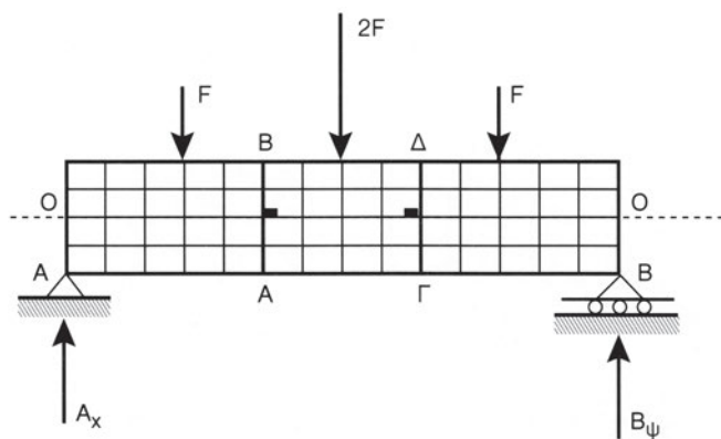
Σχήμα 8.5ζ Κάμψη της δοκού. Ουδέτερος άξονας 0 - 0
