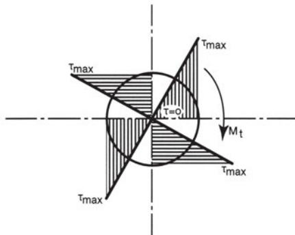
Σχήμα 11.2.β Η διανομή των τάσεων σε κυκλική διατομή
