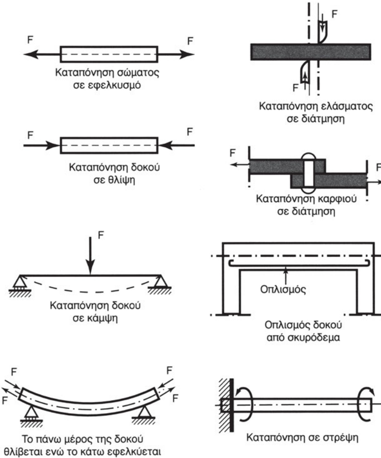
Σχήμα 5.4α Οι σπουδαιότερες καταπονήσεις
