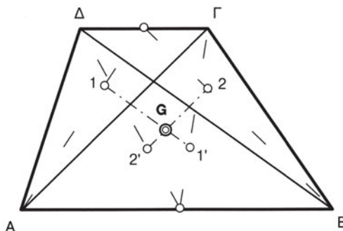
Σχήμα 4.3θ Το κεντροειδές τραπεζίου (2ος τρόπος)
