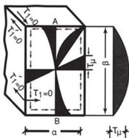
Σχήμα 11.5.δ Ορθογωνική διατομή. Η διανομή των τάσεων λόγω στρεπτικής ροπής
