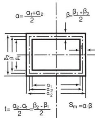
Σχήμα 11.5.γ Ορθογωνική σωληνωτή διατομή (στραντζαριστό)
