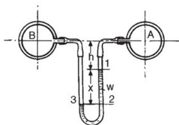
Σχήμα 15.8.δ Μέτρηση διαφοράς πίεσης μεταξύ δυο σωλήνων με διαφορικό μανόμετρο
