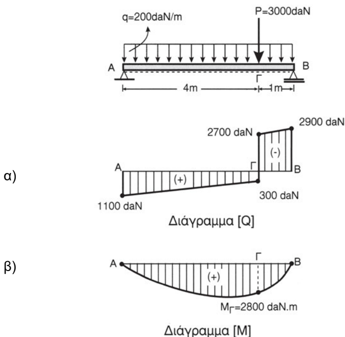
Σχήμα 10.4η Αμφιέρειστη δοκός καταπονούμενη σε κάμψη
