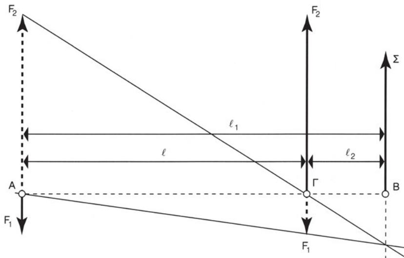
Σχήμα 3.4α Η συνισταμένη γραφικά δύο παραλλήλων και αντιπρόπων δυνάμεων.
