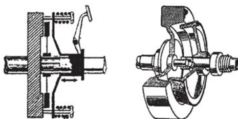
Σχήμα 14.6.6.β Είδη συμπλεκτών
