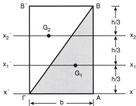
Σχήμα 7.6β Ροπή αδράνειας τριγωνικής διατομής
