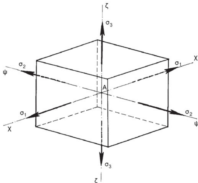
Σχήμα 12.4.3.1.α Στοιχειώδης κύβος, εντατικής κατάστασης, περί σημείο A καταπονούμενου σώματος.
