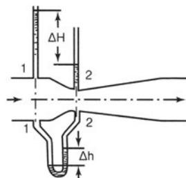
σχ. 16.8.α Μετρητής Βεντούρι
