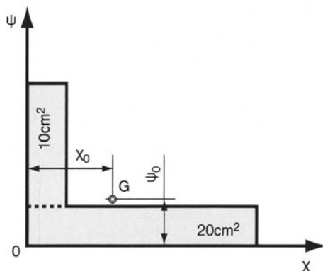
Σχήμα 4.β Η θέση του κέντρου επιφάνειας
