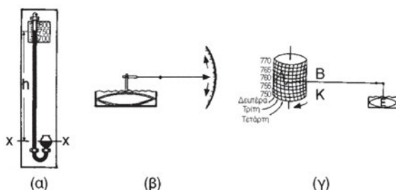
Σχήμα 15.8. α) Εργαστηριακό βαρόμετρο, β) Μεταλλικό βαρόμετρο Vidi (αρχή), γ) Αυτογραφικό όργανο (αρχή)
