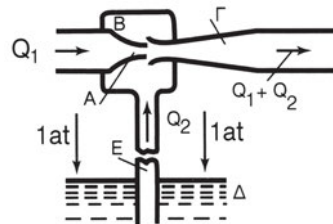
Σχήμα 16.8.γ Ψεκαστήρας
