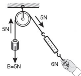
Σχήμα 13.4.2β Τροχαλία
