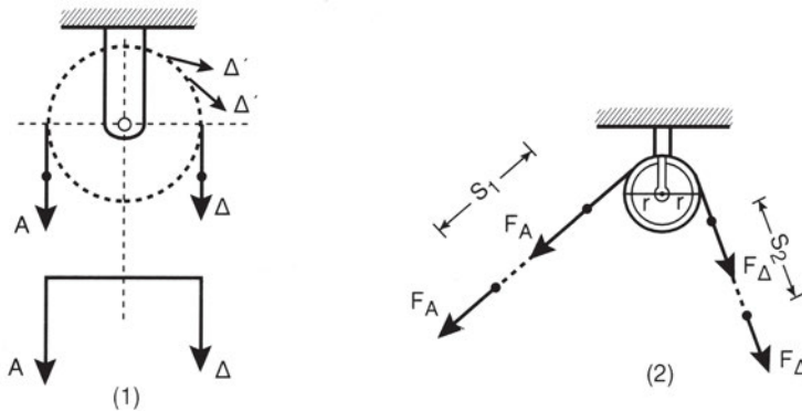
Σχήμα 13.4.2γ Τροχαλία
