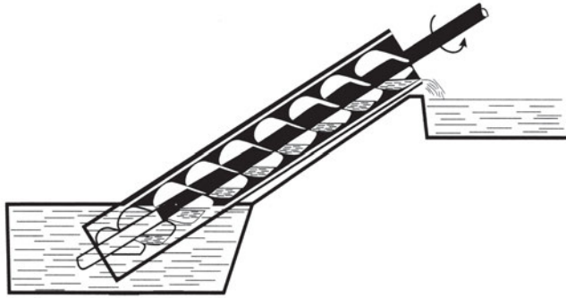
Σχήμα 13.6β Κοχλίας
