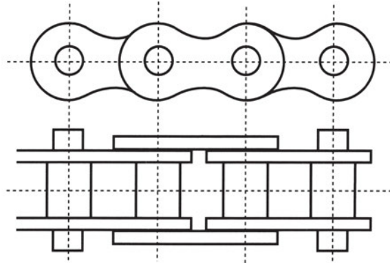
Σχήμα 13.7ζ Αλυσοκίνηση
