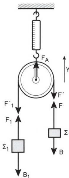
Σχήμα 13.4.2α Τροχαλία
