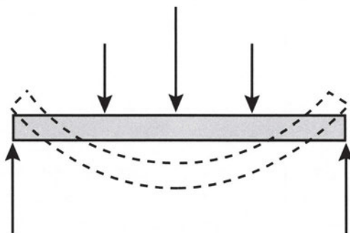
Σχήμα 10.1γ Εγκάρσια κάμψη
