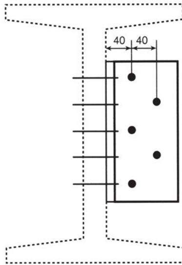
Καρφωτή σύνδεση
