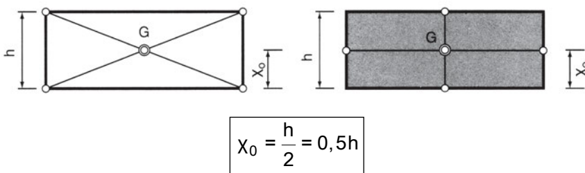
Σχήμα 4.3α Το κεντροειδές ορθογωνίου
