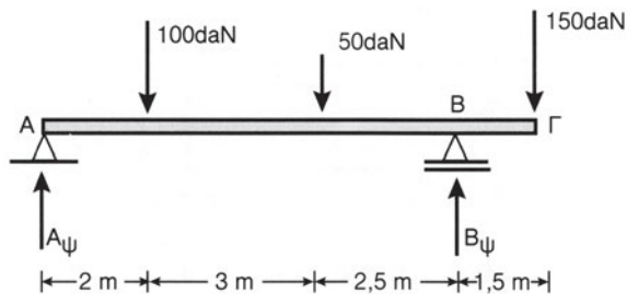
Σχήμα 8.3β Μονοπροέχουσα δοκός
