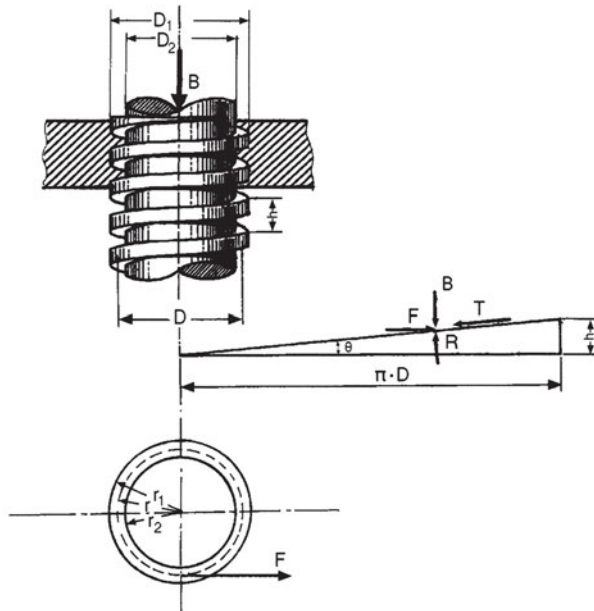
Σχήμα 14.6.3.β Κοχλίας κίνησης και το ανάπτυσμα της μέσης έλικας του σπειρώματός του.
