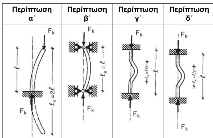
Σχήμα 12.3.5 Οι βασικές περιπτώσεις στερέωσης ράβδων, καταπανούμενων σε λυγισμό και το κατά περίπτωση ανηγμένο μήκος λυγισμού.
