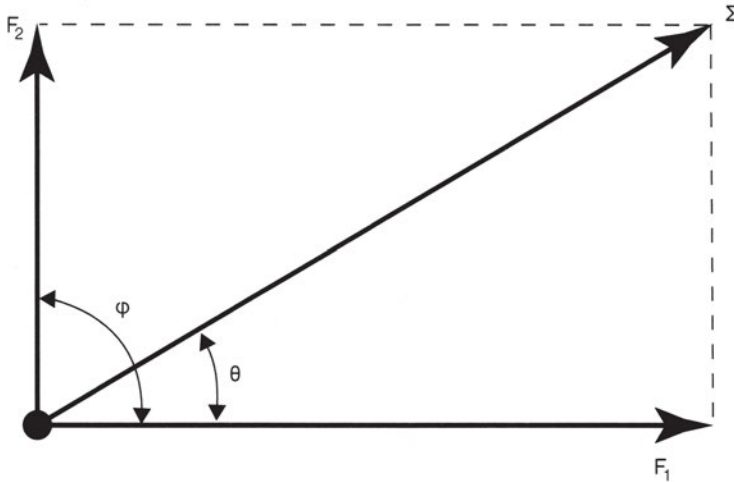
Σχήμα 3.1γ Συνισταμένη δύο δυνάμεων, υπό γωνία 90^\circ .
