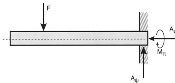
Σχήμα 8.2α Πάκτωση
