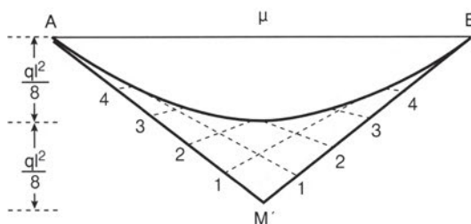
Σχήμα 8.60 Αμφιέριστη δοκός
