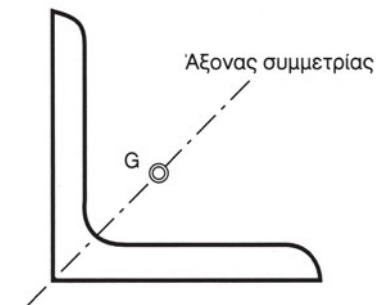
Σχήμα 4.2γ Κεντροειδές σχήματος με ένα άξονα συμμετρίας
