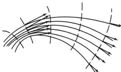
Σχήμα 16.2.β Ανομοιόμορφη μόνιμη ροή
