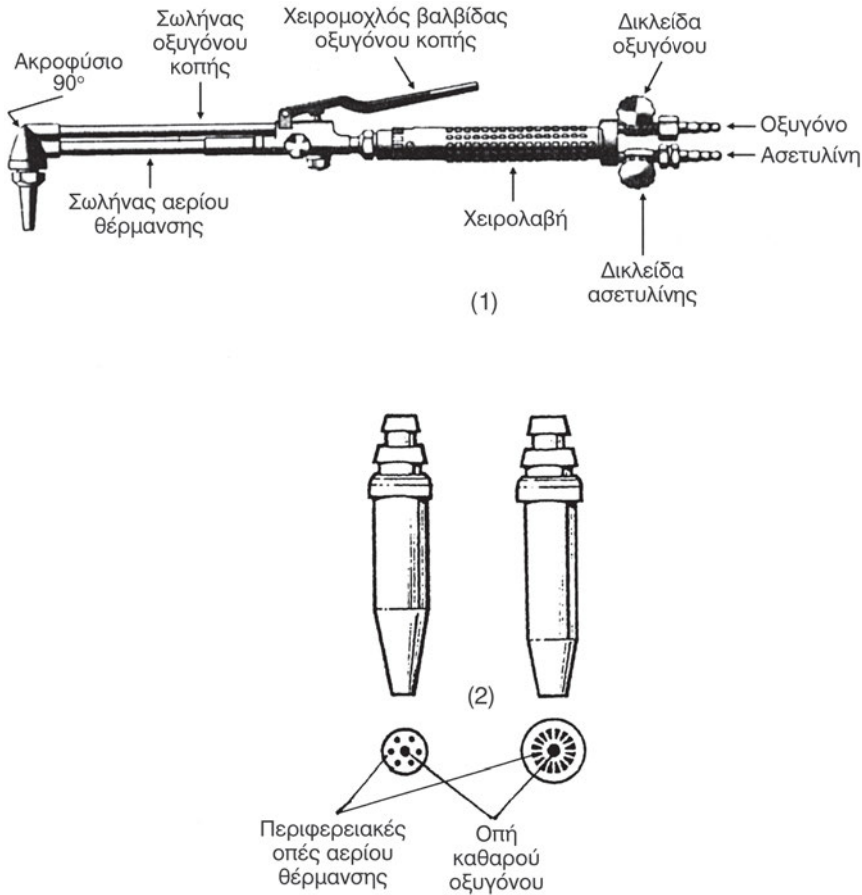
Σχήμα 8.3.12β 1) Οξυγονοκόφτης. 2) Ακροφύσια οξυγονοκόφτη.
