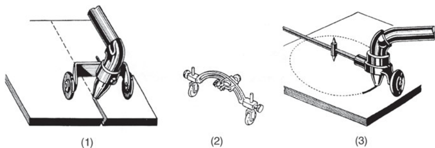
Σχήμα 8.3.12γ: 1) Ιδιοσυσσκευή με οδηγητήριους τροχούς για ευθεία οξυγονοκοπή. 2) Ιδιοσυσσκευή για οξυγονοκοπή υπό γωνία. 3) Ιδιοσυσσκευή για οξυγονοκοπή κύκλων (διαβήτη οξυγονοκοπής).
