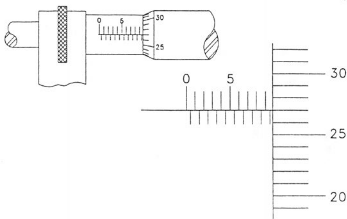
Σχήμα 3.2.5γ Ανάγνωση μικρομέτρου με βαθμό ακριβείας 0.01 mm
