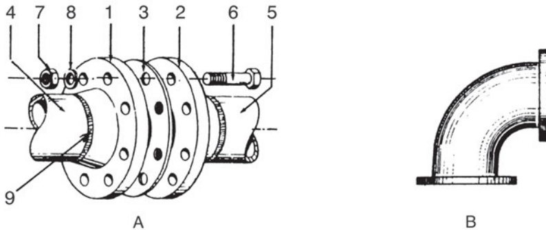
Σχήμα 9.2.1 α A) Σύνδεση σωλήνων με φλάντζες: 1,2-Φλάντζες, 3-Παρέμβυσμα, 4,5-Σωλήνες, 6-Κοχλίας, 7-Περιοκόχλιο, 8-Ροδέλλα ασφαλείας, 9-Ραφή συγκόλλησης B) Φλαντζωτό εξάρτημα (γωνία).
