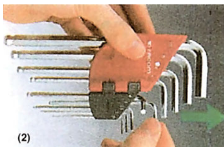
Σχήμα 4.4.2β -1. Καρυδάκι με τη μανέλλα του -2. Σειτ κλειδιών Άλλεν
