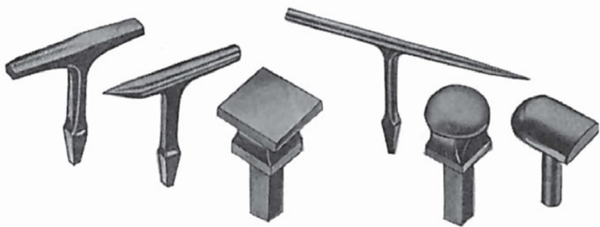
Σχήμα 4.3.2α Αμονάκια σε διάφορα σχήματα
