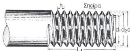
Σχήμα 4.16α Χαρακτηριστικά στοιχεία σπειρώματος
