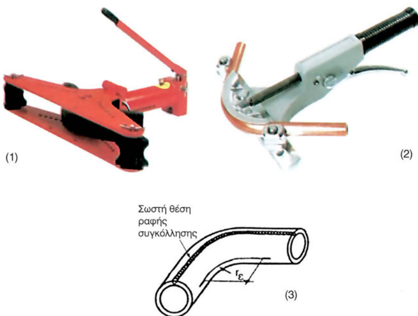
Σχήμα 9.3.4α 1) Υδραυλικός κουρμπαδόρος για κουρμπάρισμα σιδηροσωλήνων. 2) Κουρμπαδόρος κασάνιας για κουρμπάρισμα χαλκοσωλήνων. 3) Σωστή θέση της ραφής συγκόλλησης κατά την κάμψη του σωλήνα.
