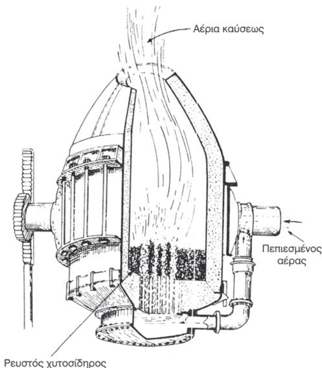
Σχήμα 2.6γ Άπιον του Μπέσσεμερ για παραγωγή χάλυβα από χυτοσίδηρο
