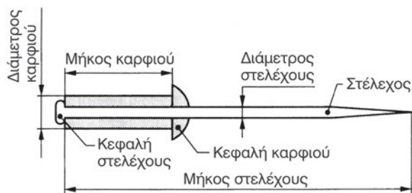
Σχήμα 7.1.2η Τα μέρη από τα οποία αποτελείται ένα τυφλοκαρφί (πριτσίνι) από αλουμίνιο
