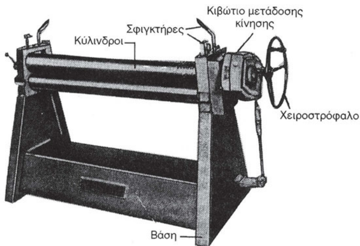
Σχήμα 6.3δ Χειροκίνητος κυλινδροπιεστής
