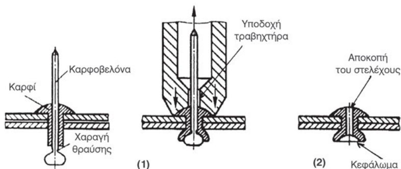
Σχήμα 7.1.2θ Καρφωτή σύνδεση με χρήση τυφλοκαρφιού και κάρφωμα με μηχανικό τραβηχτήρα (πριτσιναδόρο)
