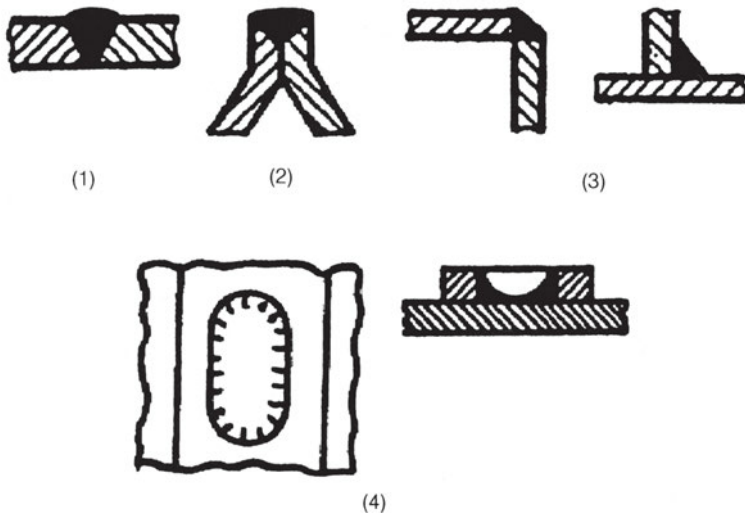
Σχήμα 8.4.8α: Είδη συγκολλητικών ραφών αναλόγως προς τη μορφή συνδέσεως των προς συγκόλληση ελασμάτων.
