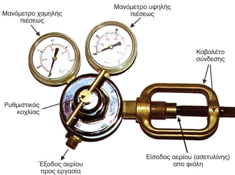
Σχήμα 8.3.4β: 1) Μανομετρικός εκτονωτής οξυγόνου. Σύνδεση στη φιάλη με τη βοήθεια μαστού. 2) Μανομετρικός εκτονωτής ασετυλίνης. Σύνδεση στη φιάλη με τη βοήθεια καβαλέτου.
