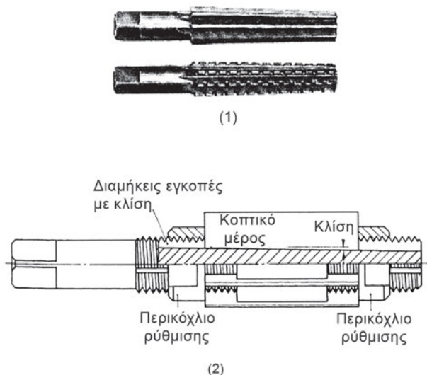
Σχήμα 4.15β -1. Κωνικά γλύφανα χειριού
