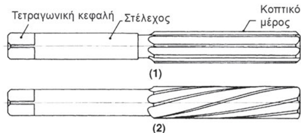
Σχήμα 4.15α -1. Παράλληλο γλύφano χεριού με ίσια δόντια -2. Παράλληλο γλύφano χεριού με ελικοειδή δόντια
