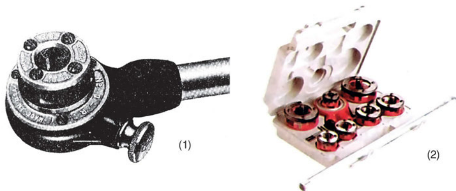
Σχήμα 9.3.5α 1) Χειροκίνητος βιδολόγος με καστάνια 2) Σετ κεφαλών (κουκουνάρες) βιδολόγου
