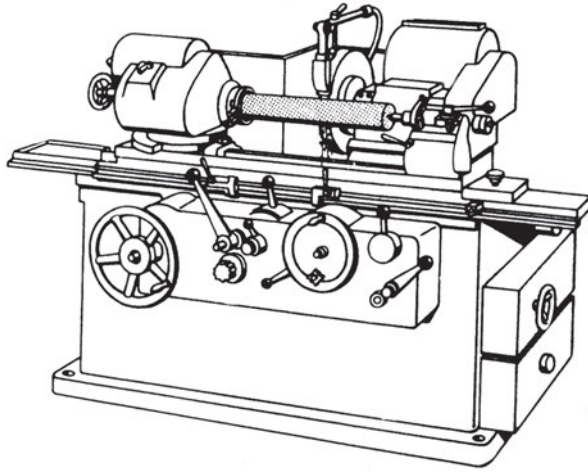
Σχήμα 13.5α Λειαντική μηχανή για εξωτερικές κυλινδρικές επιφάνειες
