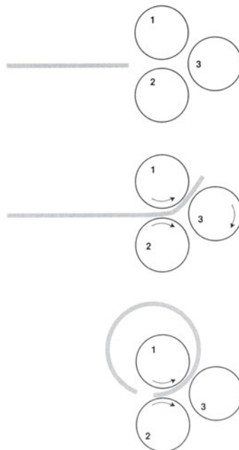
Σχήμα 6.3ε Φάσεις διαμόρφωσης σε κυλινδροπιεστή
