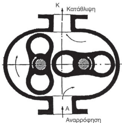
Σχήμα 16.1.1γ Αντλία με περιστρεφόμενα έμβολα (λοβούς)
