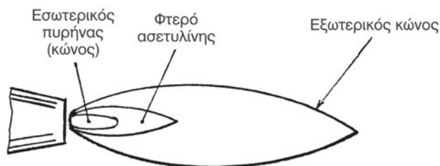
Σχήμα 8.3.9β: Αναγωγική ή ανθρακωτική φλόγα
