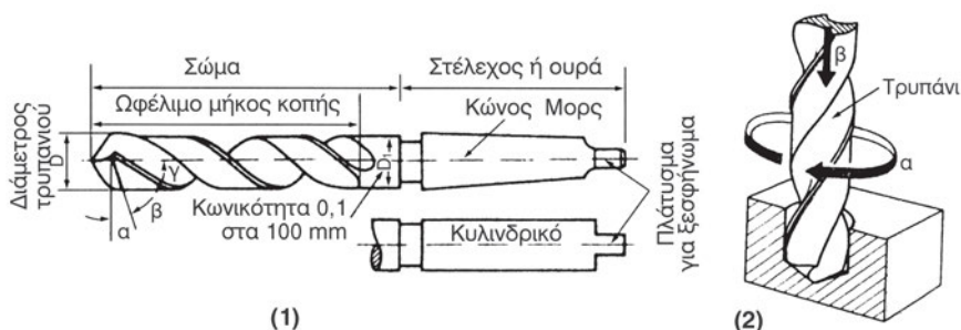
Σχήμα 4.14α -1. Τα κύρια μέρη του τρυπανιού -2. Οι κινήσεις του τρυπανιού
