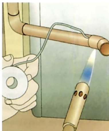
Σχήμα 8.2.2η: Κασσιτεροσυγκόλληση χαλκοσωλήνων
