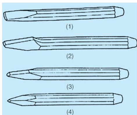
Σχήμα 4.8β -1. Πλατύ κοπίδι -2. Σταυρωτό κοπίδι -3. Μισοστρόγγυλο κοπίδι -4. Κοπίδι νύχια
