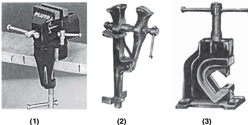
Σχήμα 4.2.2β -1. Μέγγενη εφαρμοστή -2. Μέγγενη σιδηρουργού, -3. Σωληνομέγγενη
