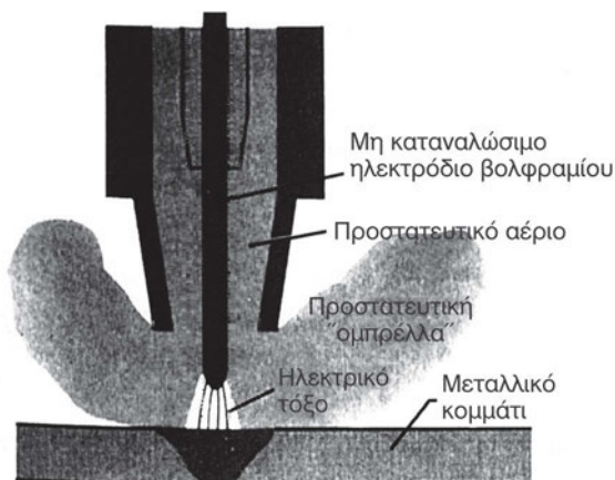
Σχήμα 8.4.10α: Ηλεκτροσυγκόλληση με μη καταναλώσιμο ηλεκτρόδιο βολφραμίου και προστατευτικό αέριο (TIG)
