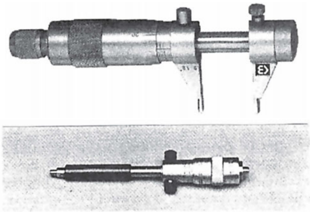
Σχήμα 3.2.5ε Μικρόμετρα μέτρησης εσωτερικών διαστάσεων
