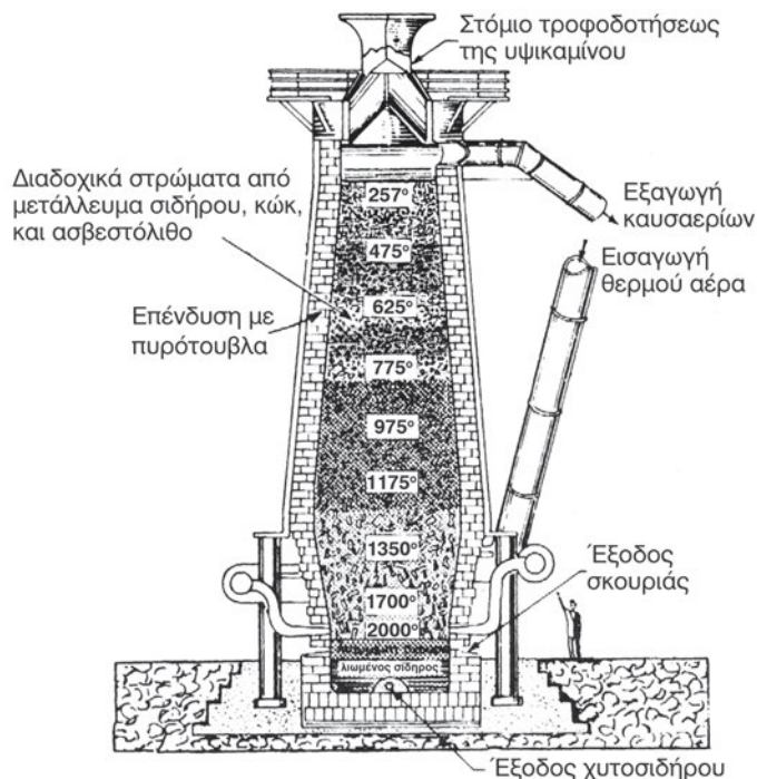
Σχήμα 2.6α Σχηματική παράσταση υψικαμίνου
