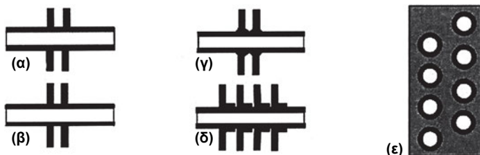
Σχήμα 2.16: Διάφοροι τρόποι στερέωσης των πτερυγίων στους σωλήνες του συμπυκνωτή (α,β,γ,δ), (ε) μεγάλο πολλαπλό πτερύγιο.
