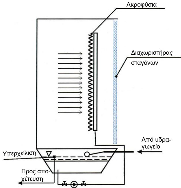
Σχήμα 2.46: Θάλαμος ακροφυσίων.
