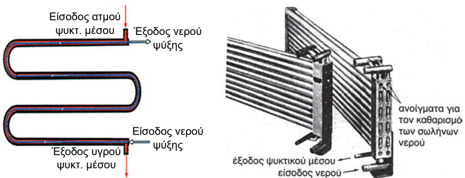
Σχήμα 2.20: Σπειροειδής ομοαξονικός σωλήνας (1) και στοιχείο υδρόψυκτου συμπτυκνωτή με παράλληλους ομοαξονικούς σωλήνες (2). Ο μηχανικός καθαρισμός των σωλήνων νερού γίνεται αφού πρώτα αφαιρεθεί το πλευρικό σχετικό κάλυμμα.
