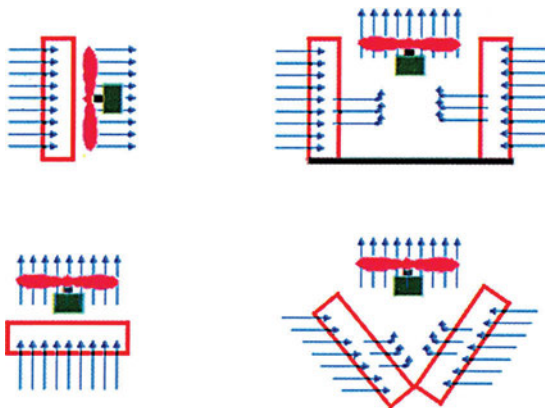
Σχήμα 2.17: Σχηματική παράσταση θέσεων εγκατάστασης πτερυγοφόρων στοιχείων εναλλαγής θερμότητας αερόψυκτου συμπυκνωτή.
