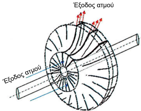
Σχήμα 2.11: Πτερυγιοφόρο στοιχείο φυγοκεντρικού συμπιεστή, ακτινικής απόκλισης.
