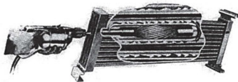
Εικόνα 2.6: Μηχανικός καθαρισμός εσωτερικού σωλήνων υδρόψυκτου συμπτυκνωτή παράλληλων ομοαξονικών σωλήνων.
