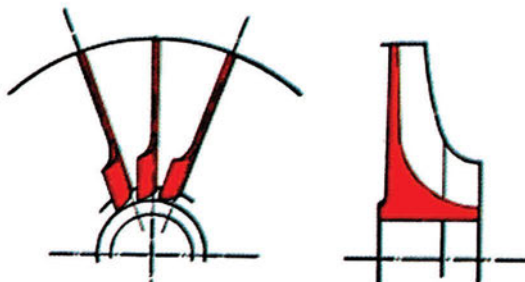
Σχήμα 2.13: Φτερωτή φυγοκεντρικού συμπιεστή με ακτινικά πτερύγια.
