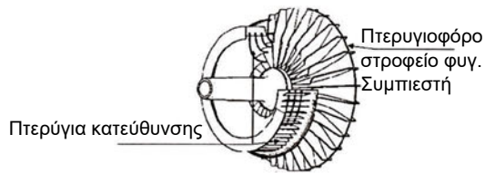
Σχήμα 2.10: Σχηματική παράσταση πτερυγιοφόρου στροφέιου φυγοκεντρικού, συμπιεστή αξονικής εισόδου, με πτερύγια κατεύθυνσης.
