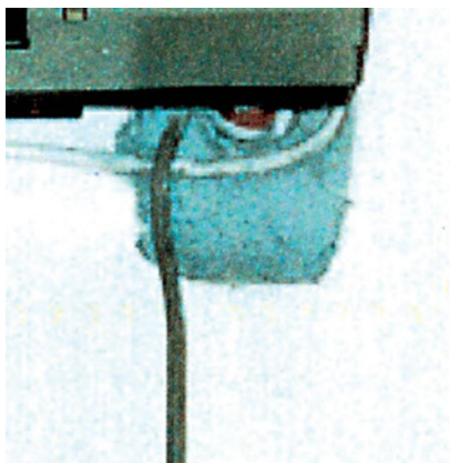
Εικόνα 3.18: Σφράγισμα της τρύπας, απ' όπου περνούν οι σωλήνες του ψυκτικού, με ελαφροτσιμέντο. (Το άσπρο καλώδιο είναι για την ηλεκτροδότηση της μονάδας, ενώ το σκουρόχρωμο είναι του ενσύρματου τηλεχειριστηρίου).
