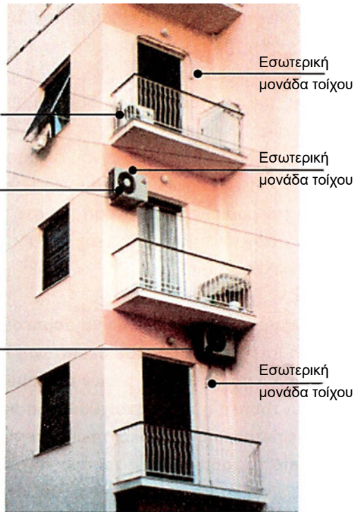
Εικόνα 3.10: Εξωτερικές μονάδες κλιματιστικών, διαιρούμενου τύπου, για μικρούς χώρους μιας κατοικίας με διάφορους τρόπους εγκατάστασής τους (ορθούς-λανθασμένους).
