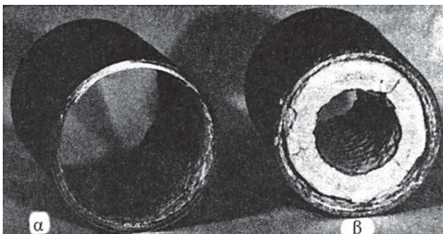
Εικόνα 2.5: Σχηματισμός κρούστας στους σωλήνες ενός υδρόψυκτου συμπυκνωτή. Επικαθήσεις όταν χρησιμοποιείται: α) αποσκληρυμένο νερό και β) με σκληρό νερό (δεν έχει γίνει αποσκλήρυνση).
