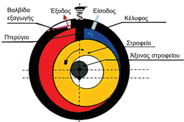
Σχήμα 2.5: Σχηματική παράσταση (σε τομή) βασικών δομικών στοιχείων περιστροφικού συμπιεστή με σταθερό σύρτη (πτερύγιο) και έκκεντρο στροφέιο.
