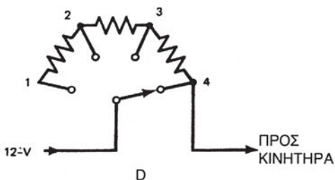
Σχήμα 6.26: Ροοστάτης που ρυθμίζει την ταχύτητα του κινητήρα.
