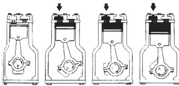
Σχήμα 6.6: Εισαγωγή ή χρόνος αναρρόφησης.
