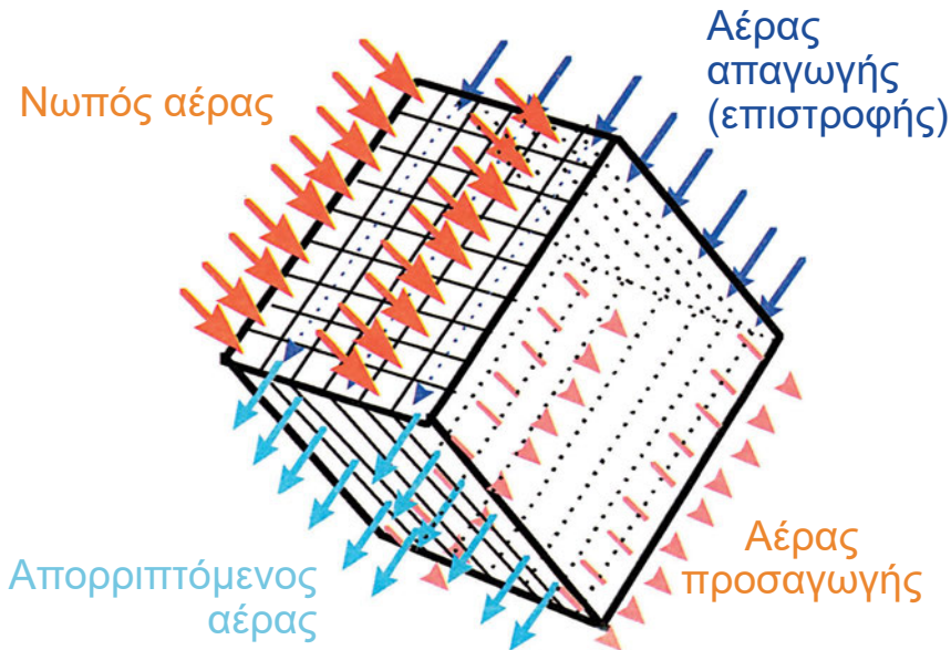
Σχήμα 3.9β: Πλακοειδής εναλλάκτης με διάταξη «σταυρορροής» των δύο ρευστών.
