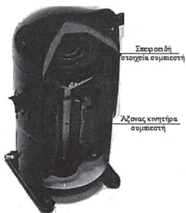
Εικόνα 2.2: Σπειροειδής συμπιεστής.
