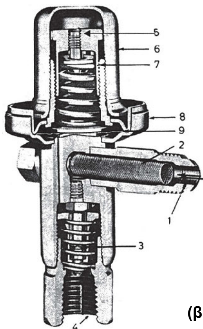
Σχήμα 2.30: (α) Σχηματική παράσταση δομής και αρχής λειτουργίας πιεζοστατικής εκτονωτικής βαλβίδας. 1. Είσοδος ψυκτικού υγρού. 2. βαλβίδα (βελονοειδής δισκοειδής κ.λπ.). 3. Έδρα βαλβίδας. 4. Στέλεχος βαλβίδας. 5. Μembrάνη. 6. Ελατήριο προέντασης. 7. Καπάκι χώρου-θαλάμου membrάνης. 8. Έξοδος ψυκτικού μέσου (υγρό + ατμός). 9. Ελατήριο ρύθμισης. 10. κοχλίας ρύθμισης. (β) Εικόνα πιεζοστατικής βαλβίδας εκτόνωσης με membrάνη. 1. Είσοδος ψυκτικού μέσου. 2. Μεταλλικό φίλτρο. 3. Βαλβίδα και έδρα βαλβίδας. 4. Έξοδος ψυκτικού μέσου. 5. Ρύθμιση ελατηρίου και πίεσης ατμοποίησης. 6. Καπάκι βαλβίδας. 7. Ελατήριο ρύθμισης. 8. Κέλυφος. 9. Μembrάνη.
