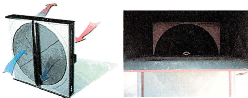
Σχήμα 3.10: Τροχός ανάκτησης θερμότητας/υγρασίας. Σχηματική διάταξή του (αριστερά) και εγκατάστασή του σε ΚΚΜ (δεξιά).
