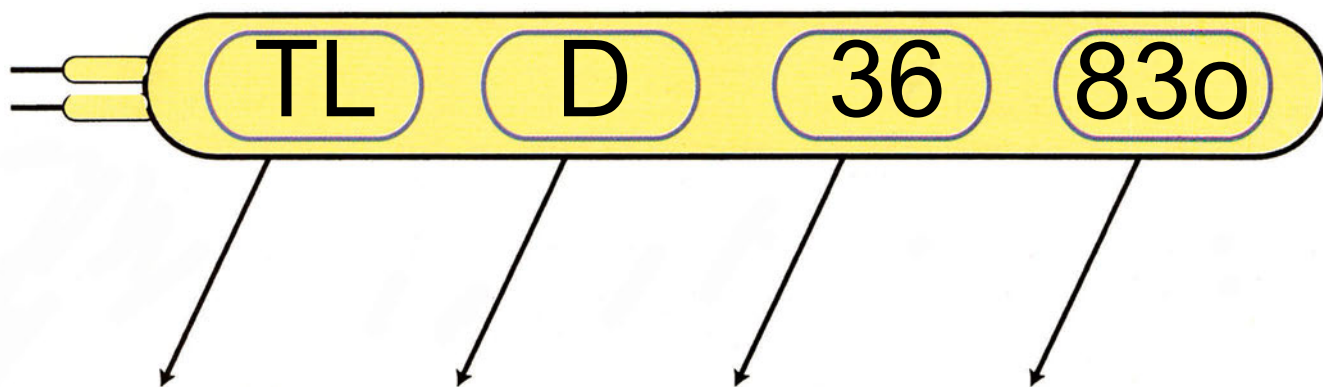
Σχήμα 3.32: Παράδειγμα αποκωδικοποίησης χαρακτηριστικών λαμπτήρα φθορισμού
