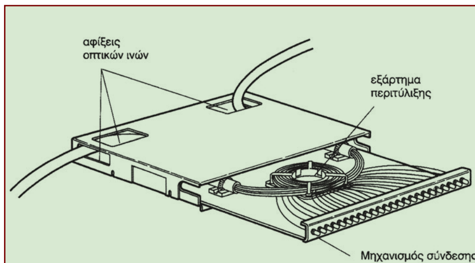
Σχήμα 3.15 : Συρτάρια οπτικών ινών.
