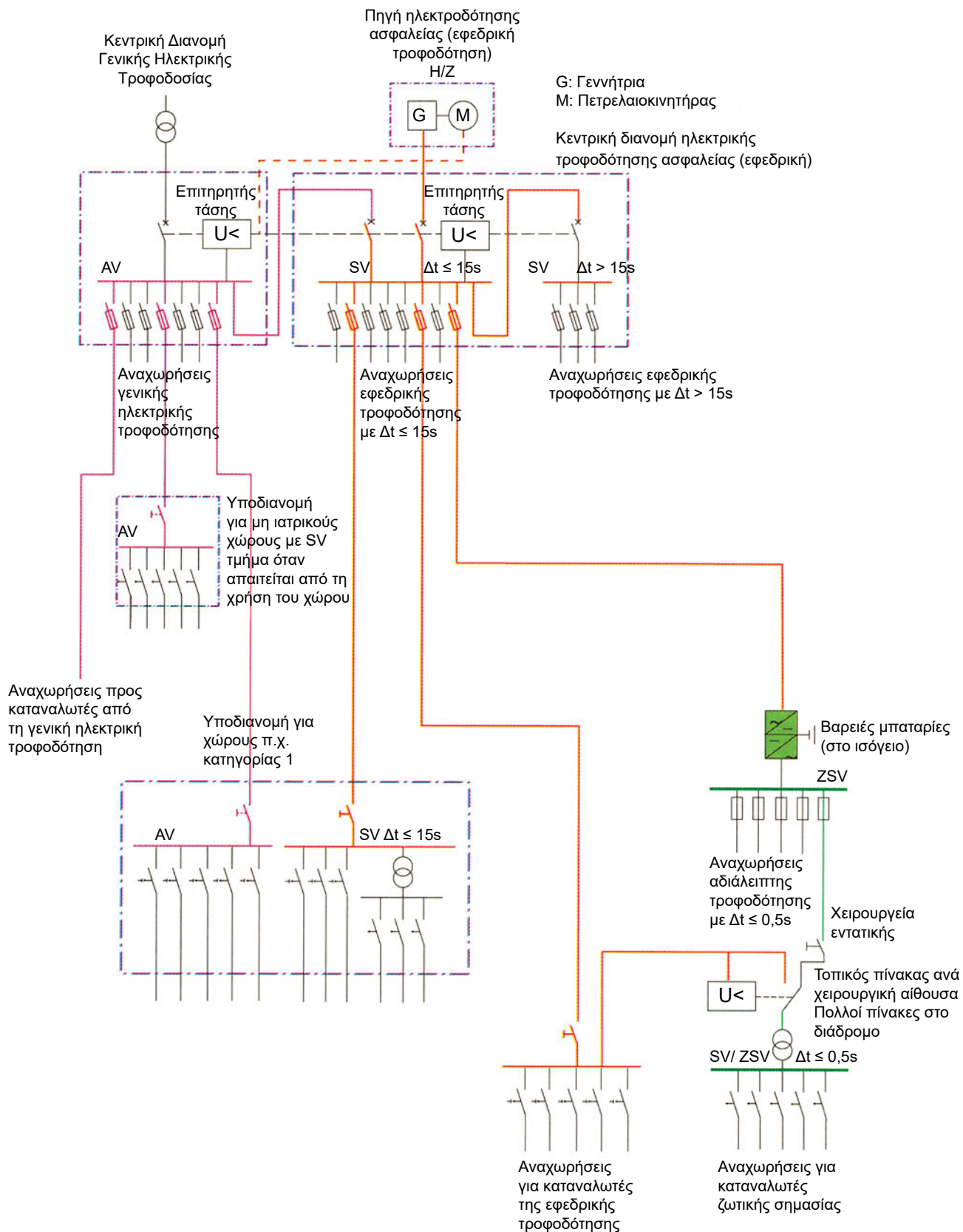
Σχήμα 1.2: Γενικό διάγραμμα διανομής ηλεκτρικής ενέργειας.
