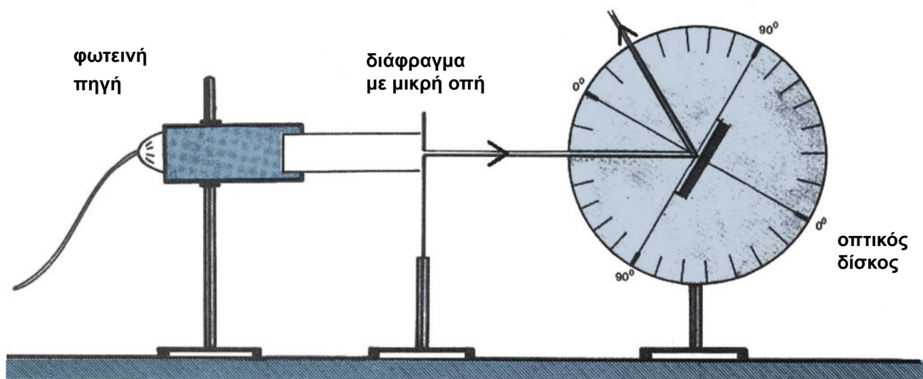
Σχήμα 1.5 Ανάκλαση φωτεινής ακτίνας σε πειραματική διάταξη.
