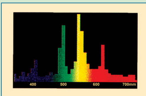
Σχήμα 3.35: Φασματική κατανομή λαμπτήρα ατμών υδραργύρου, βελτιωμένου φάσματος
