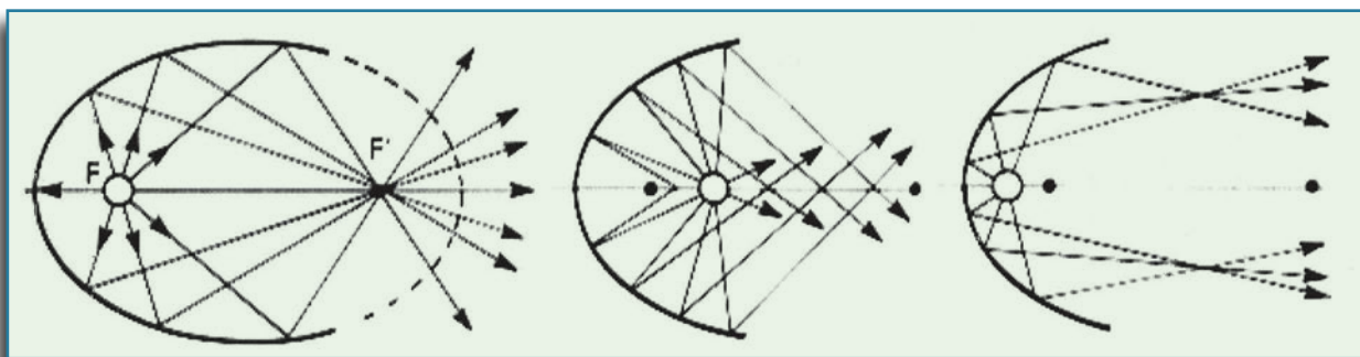
Σχήμα 1.3: Αποκλίνουσα, παράλληλη, συγκλίνουσα φωτεινή δέσμη
