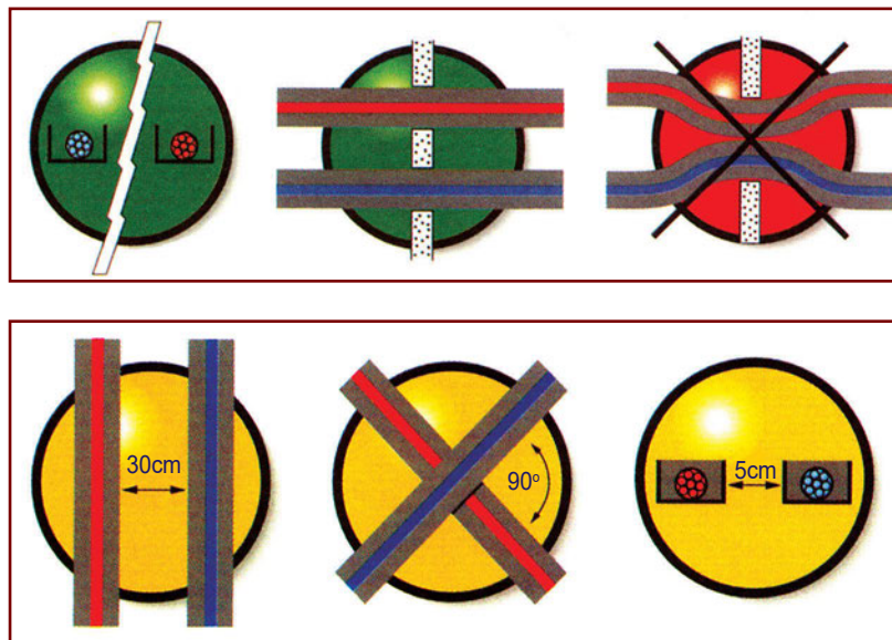
Σχήμα 6.5: Αποφυγή γειννίασης
