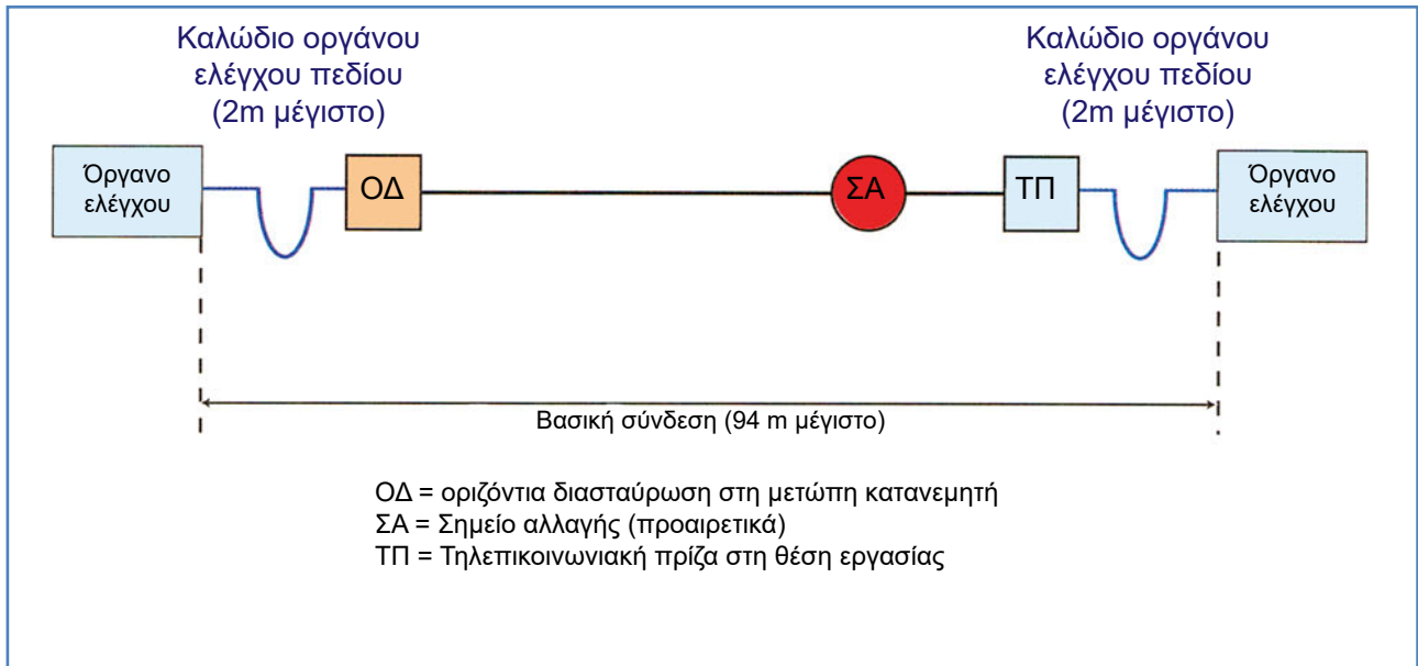
Σχήμα 5.1: Βασικός σύνδεσμος (TIA).
