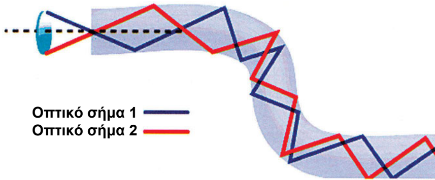
Σχήμα 3.8: Διάγραμμα ολικής εσωτερικής ανάκλασης σε οπτική ίνα.
