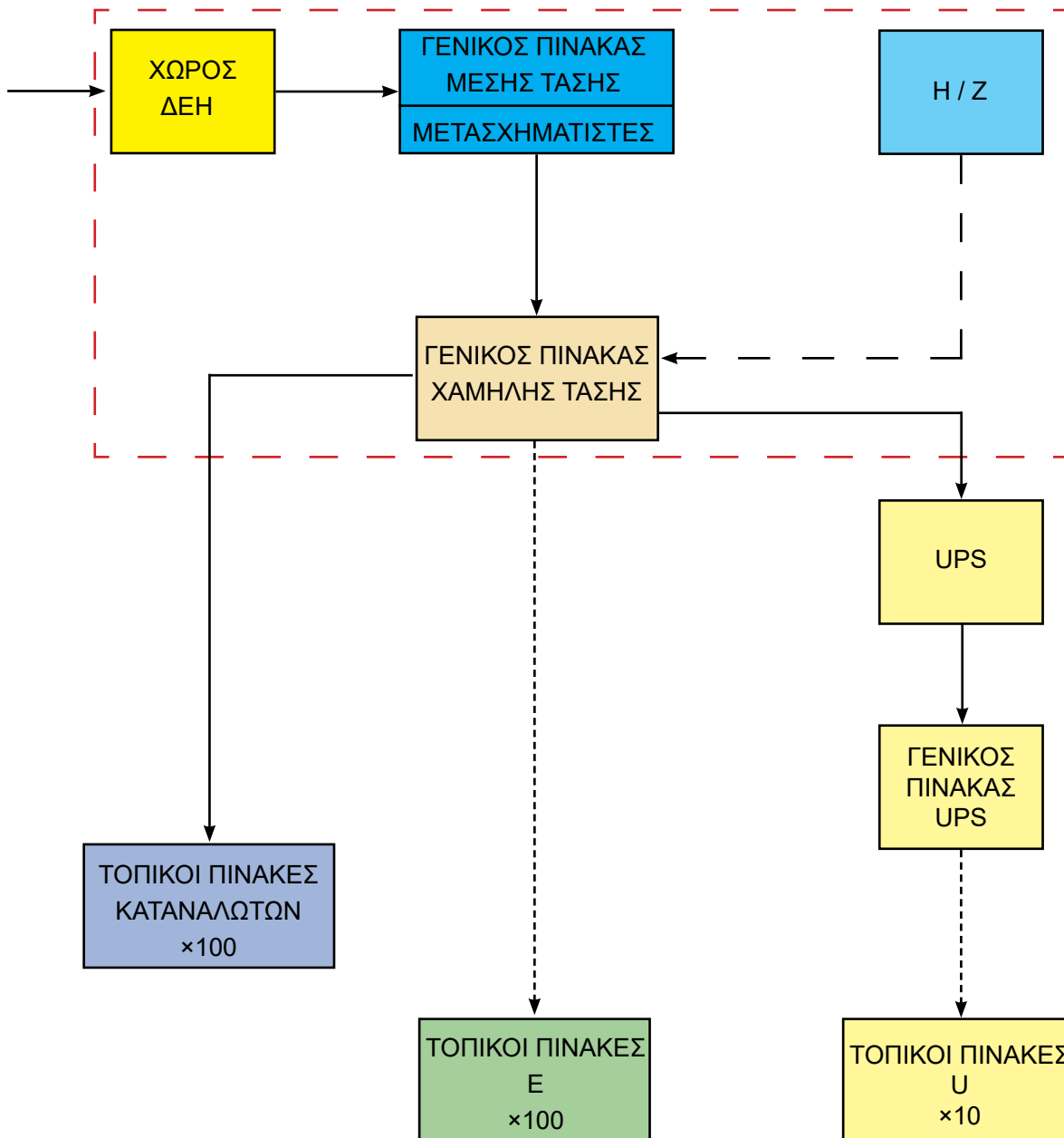
Σχήμα 1.1: Διάγραμμα ηλεκτρικής εγκατάστασης.
