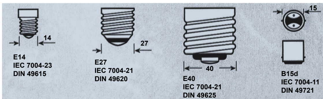
Σχήμα 3.3: Διάφοροι τύποι από κάλυκες
