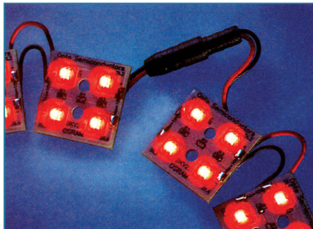
Σχήμα 4.9: Δίοδοι φωτοεκπομπής
