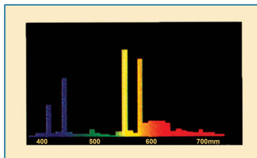
Σχήμα 3.34: Φασματική κατανομή λαμπτήρα ατμών υδραργύρου
