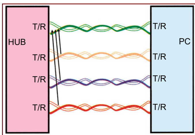
Σχήμα 4.7: Αθροιστική αλληλεπίδραση.
