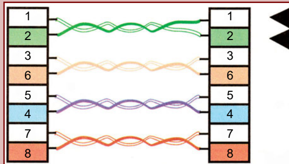
Το λάθος της αναστροφής ζευγαριού.
