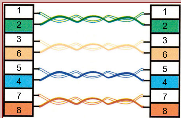
Σωστή συρμάτωση 4 ζευγαριών.
