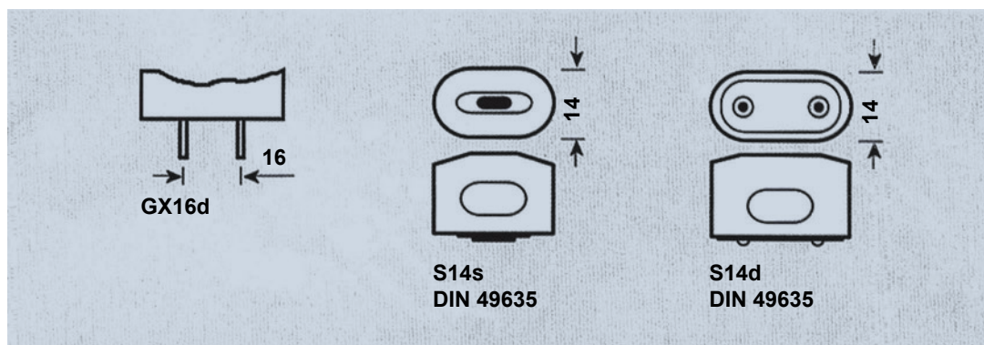
Σχήμα 3.3: Διάφοροι τύποι από κάλυκες
