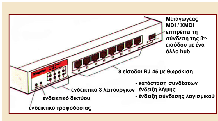
Σχήμα 1.12: Συγκεντρωτής (hub).
