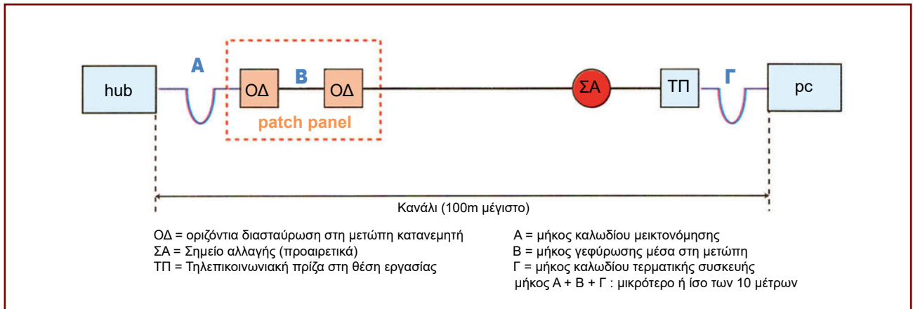
Σχήμα 5.3: Κανάλι (TIA, ISO).
