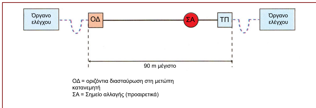
Σχήμα 5.2: Μόνιμος σύνδεσμος (ISO).
