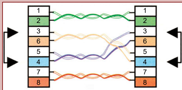
Το λάθος της διασταύρωσης ζευγαριού.
