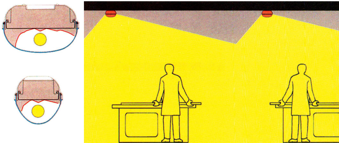
Σχήμα 4.13: Κατανομή φωτός με ανταυγαστήρα ασύμμετρης δέσμης
