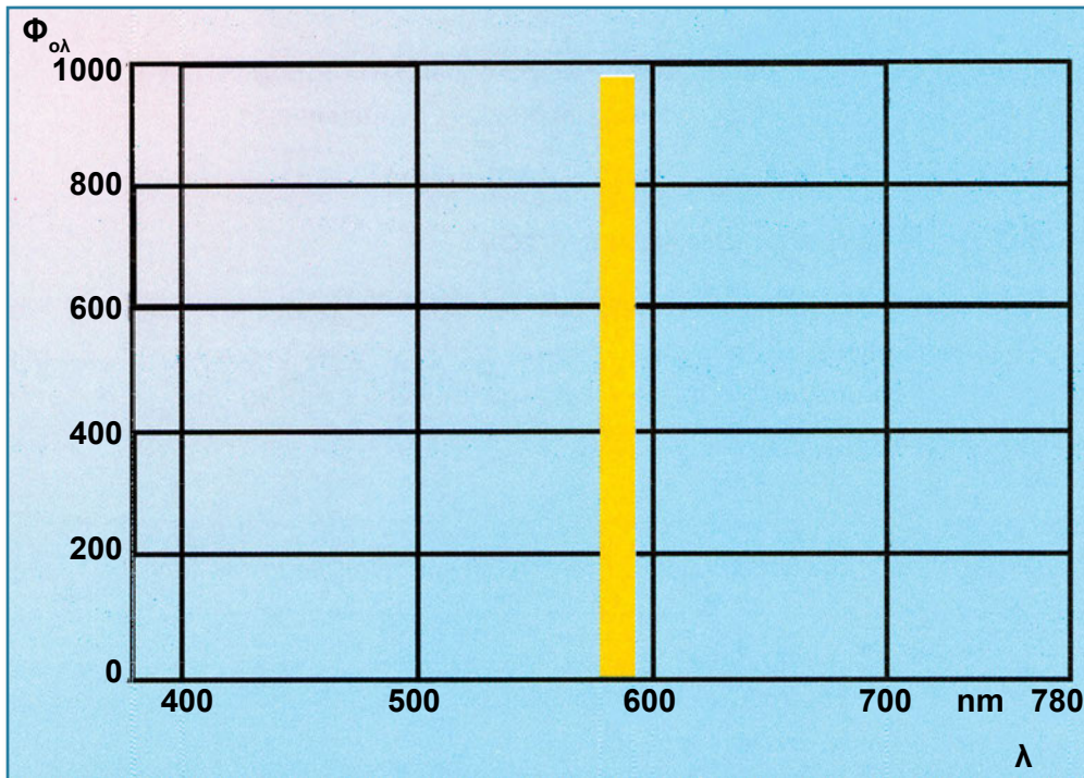
Σχήμα 3.39: Φασματική κατανομή λαμπτήρα νατρίου, χαμηλής πίεσης
