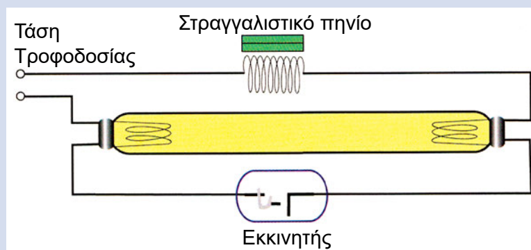
Σχήμα 3.20: Συνδεσμολογία λαμπτήρα φθορισμού
