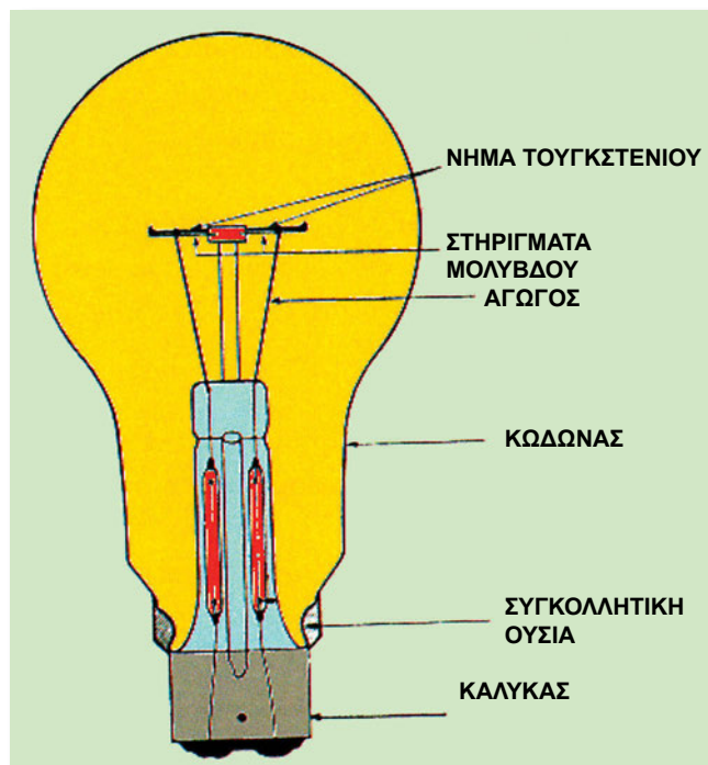
Σχήμα 3.1: Λαμπτήρας πυράκτωσης και τα μέρη που τον αποτελούν
