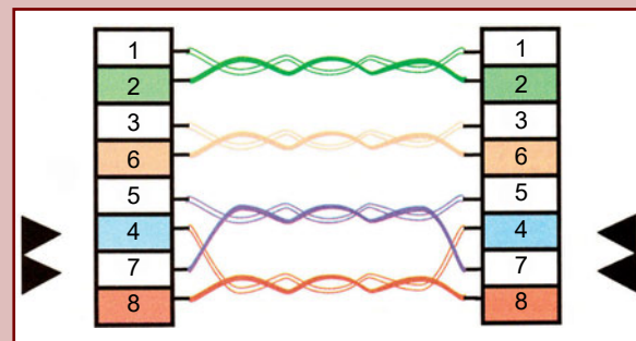
Το λάθος του διαχωρισμού ζευγαριού.
