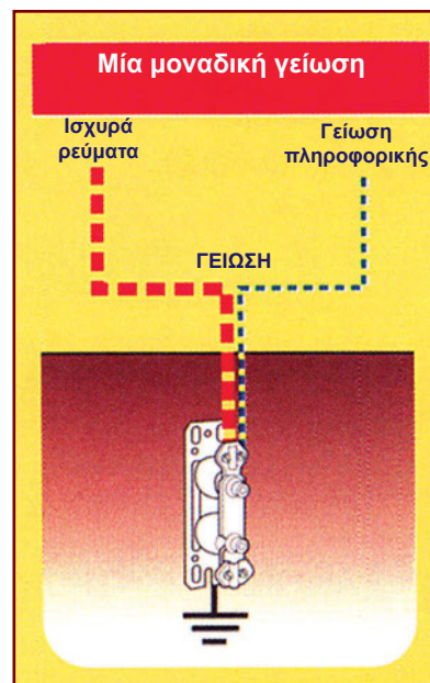
Σχήμα 6.3: Γειώσεις.
