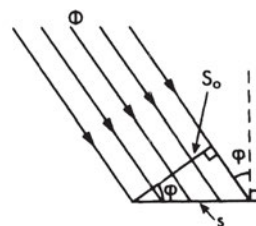
Σχήμα 2.7α: Φωτισμός επιφάνειας υπό γωνία
