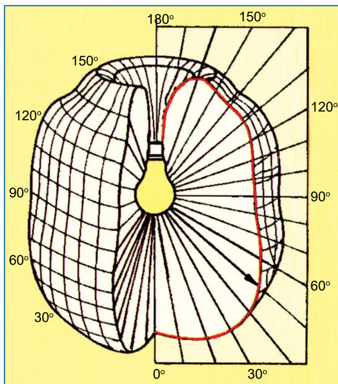
Σχήμα 2.4: Καμπύλη φωτεινής έντασης και φωτομετρικό στερεό
