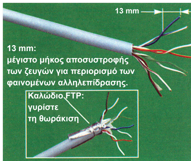
Σχήμα 6.1: Τερματισμός καλωδίων.
