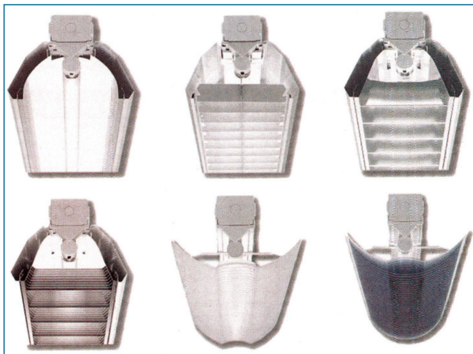
Σχήμα 4.14: Τύποι ανταυγαστήρων
