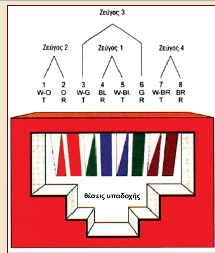
Πρότυπο T568B
