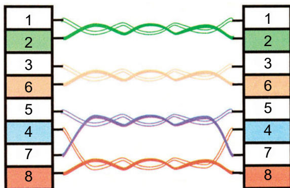
Σχήμα 4.3: Το λάθος της διασταύρωσης ζευγαριού.
