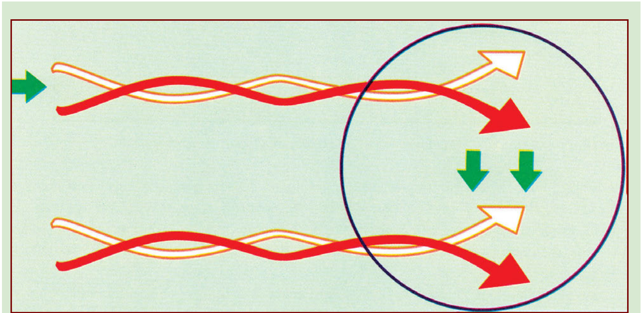
Σχήμα 4.8: Μακρινή αλληλεπίδραση.
