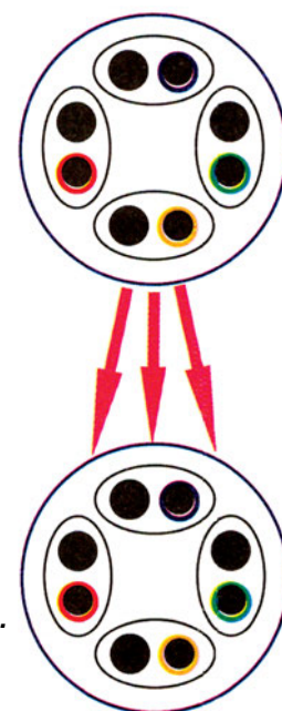
Σχήμα 4.9: Εξωτερική αλληλεπίδραση.
