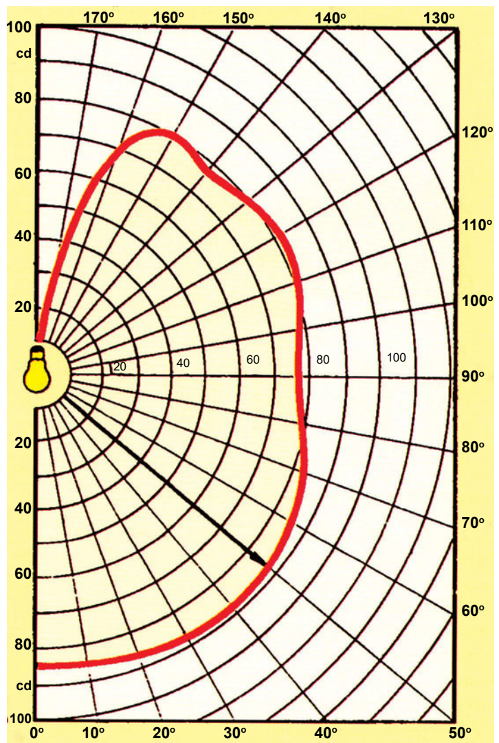
Σχήμα 2.5: Καμπύλη φωτεινής έντασης λαμπτήρα πυράκτωσης
