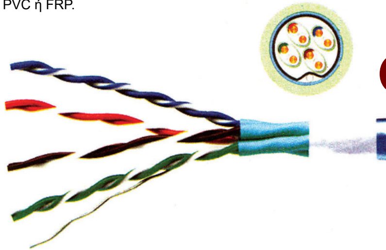
Σχήμα 3.4: Καλώδιο FTP.
