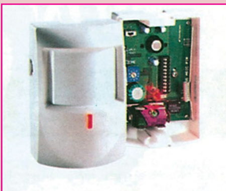
Σχήμα 6.7: Ανιχνευτής υπέρυθρης ακτινοβολίας
