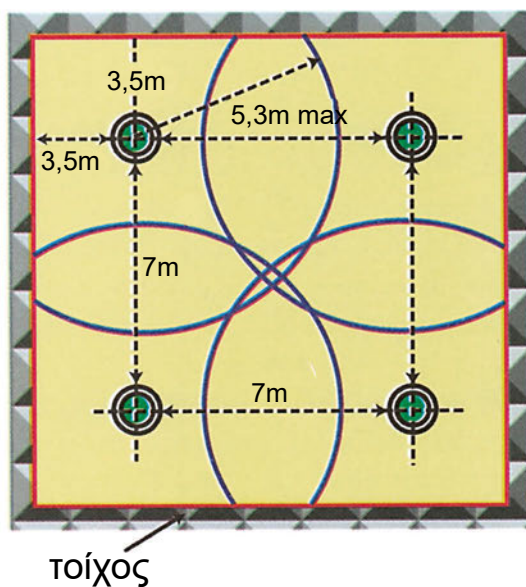
Σχήμα 1.1: Κατανομή ανιχνευτών σε κάτοψη χώρου
