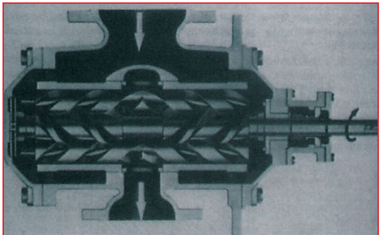
Εικόνα 8.3: Περιστροφική αντλία
