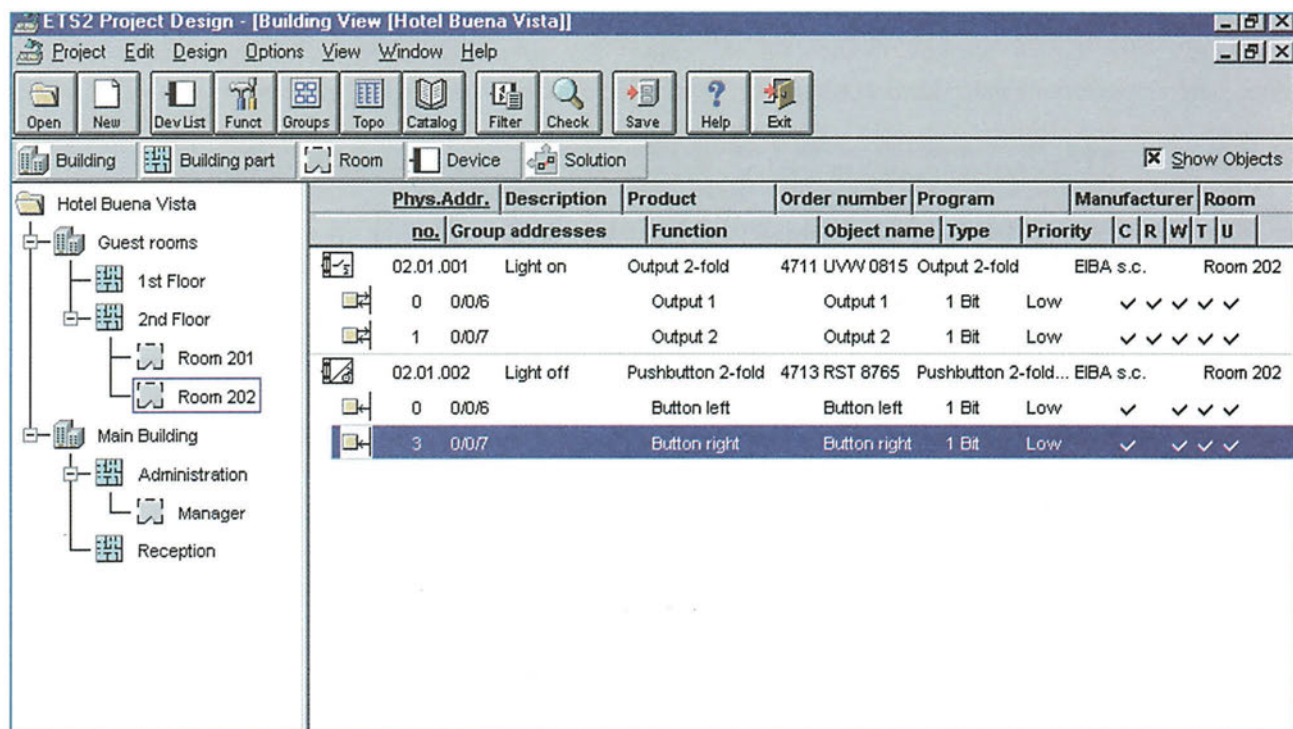
Σχήμα 4.6: Κτιριακή απεικόνιση με λειτουργικά υποσυστήματα
