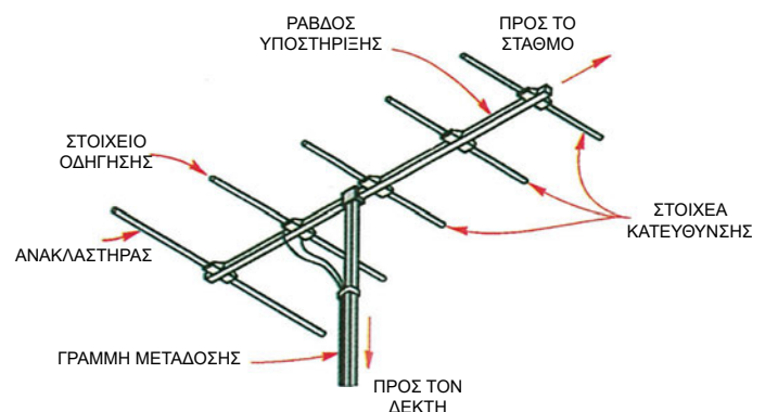
Σχήμα 3.3: Εξωτερική κεραία τηλεόρασης
