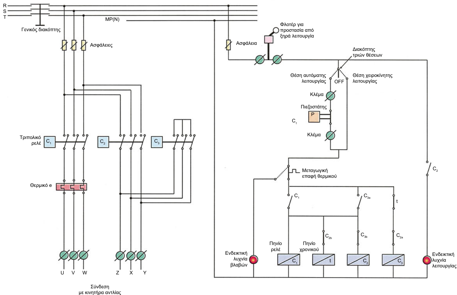
Σχήμα 8.6 Κύριο και βοηθητικό κύκλωμα κύριας αντλίας πυροσβεστικού συγκροτήματος
