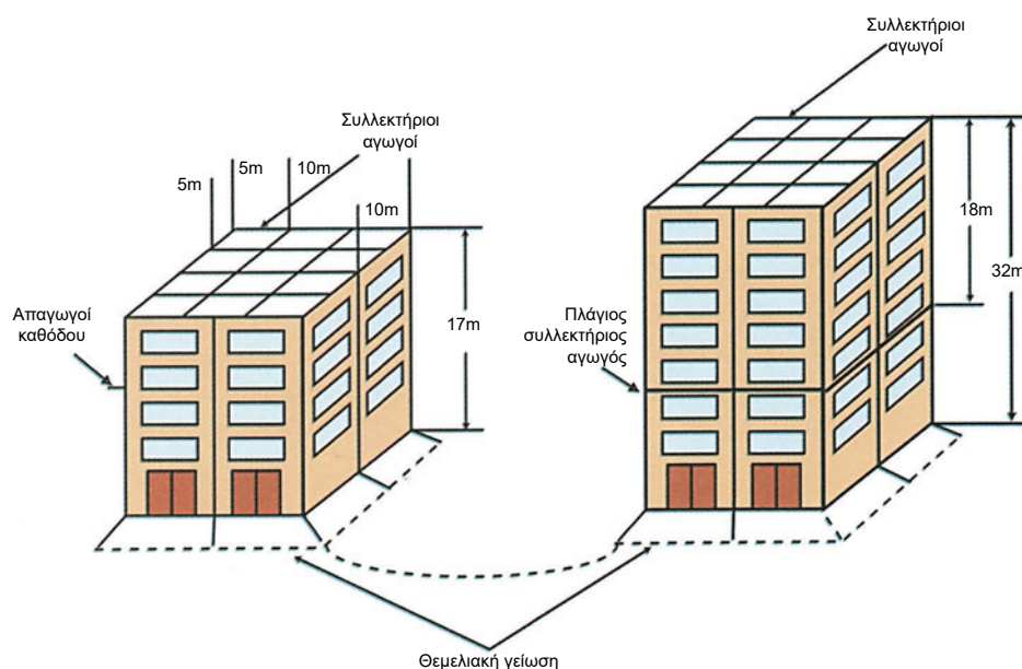
Σχήμα 4.6: Αλεξικέραυνο τύπου κλωβού Faraday
