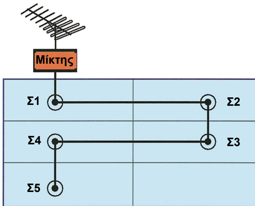
Σχήμα 3.7: Παράδειγμα εγκατάστασης
