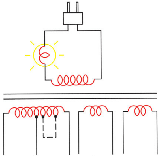
Κύκλωμα με σφάλμα βραχυκυκλωμένων σπειρών
