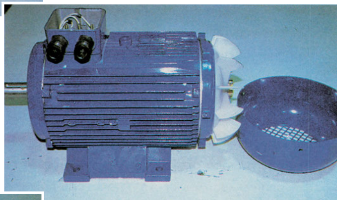
Κινητήρας μετά την αφαίρεση προστατευτικού καλύμματος
