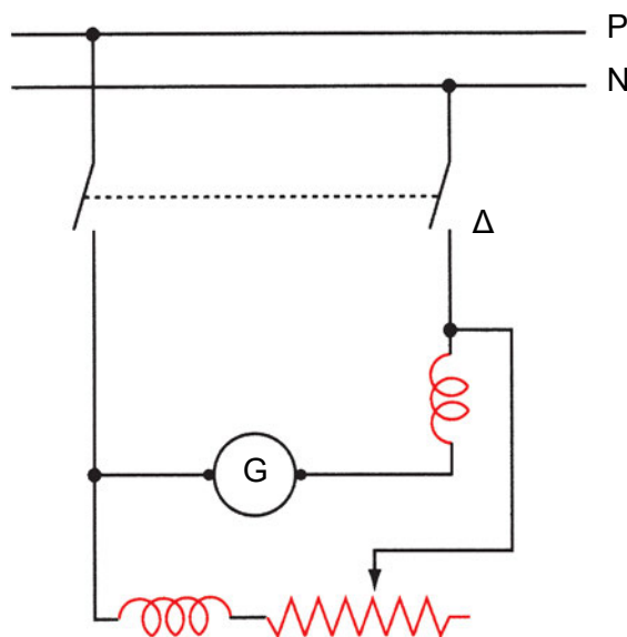
Κύκλωμα γεννήτριας σύνθετης διέγερσης
