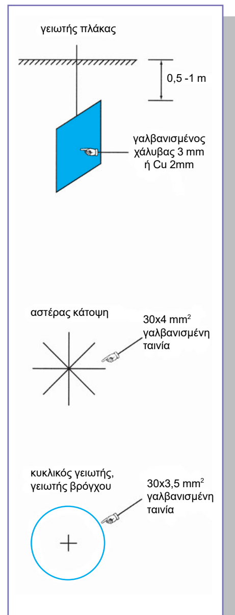
Σχηματικές διατάξεις γειωτών
