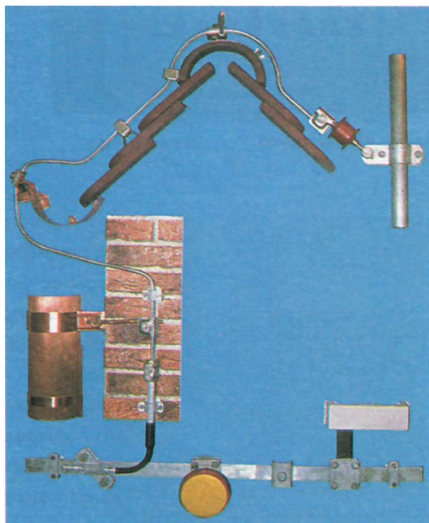
Διάταξη εξωτερικής αντικεραυνικής προστασίας
