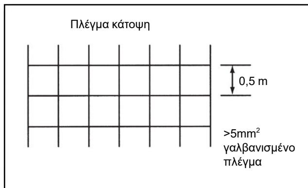
Πλέγμα γείωσης
