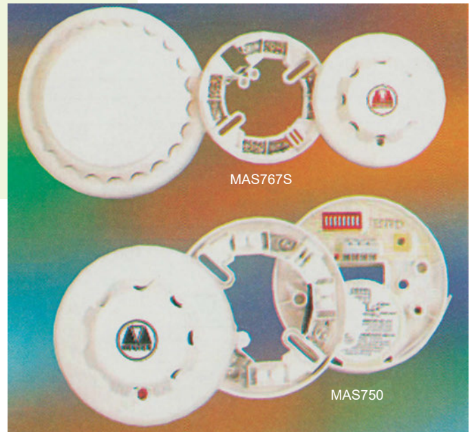
Ανιχνευτές αποσυναρμολογημένοι
