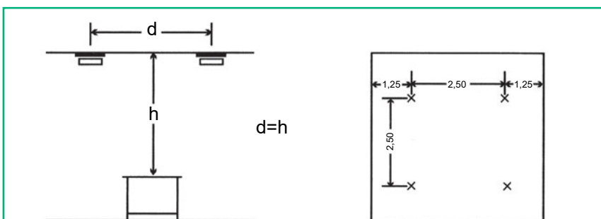
Σχηματική διάταξη της απόστασης μεταξύ των λαμπτήρων και του ύψους από το επίπεδο εργασίας
