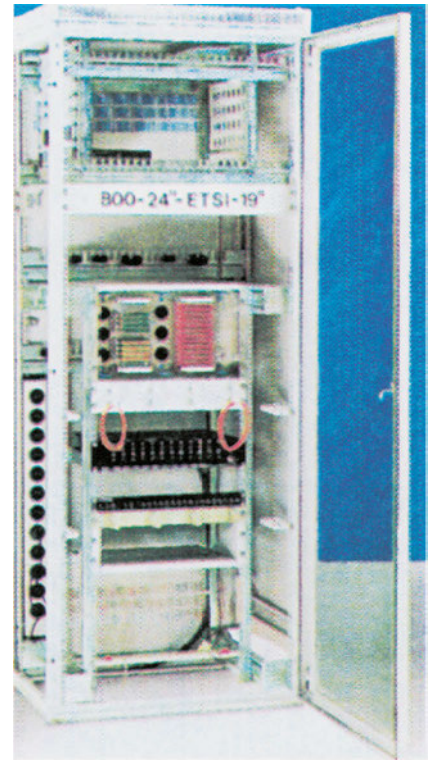
Επιδαπέδιος κατανεμητής (Rack)
