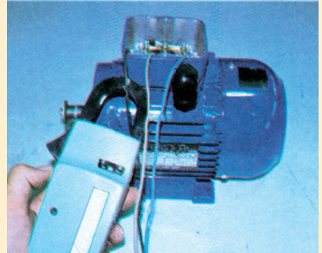
Μέτρηση της έντασης του ρεύματος με αμπεροτσιμπίδα
