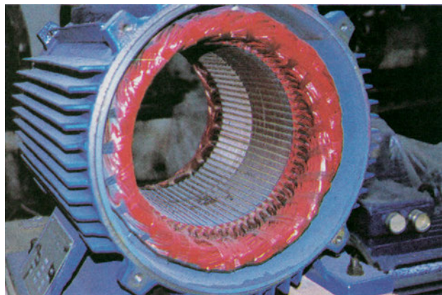
Τύλιγμα στάτη
