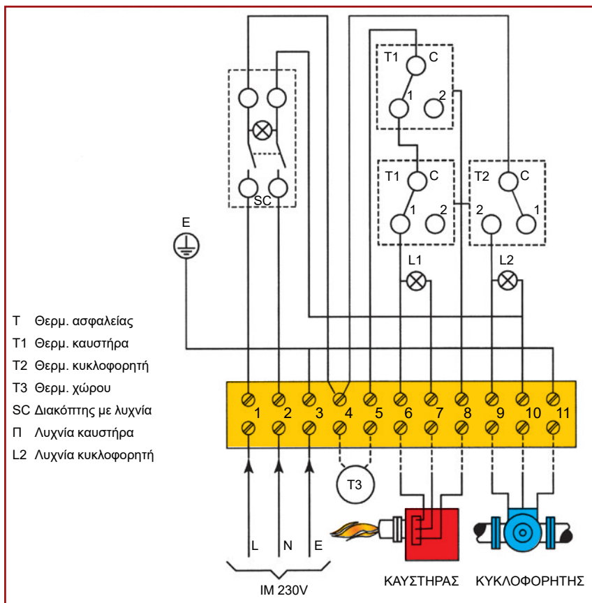
Ηλεκτρικό διάγραμμα σύνδεσης πίνακα λέβητα
