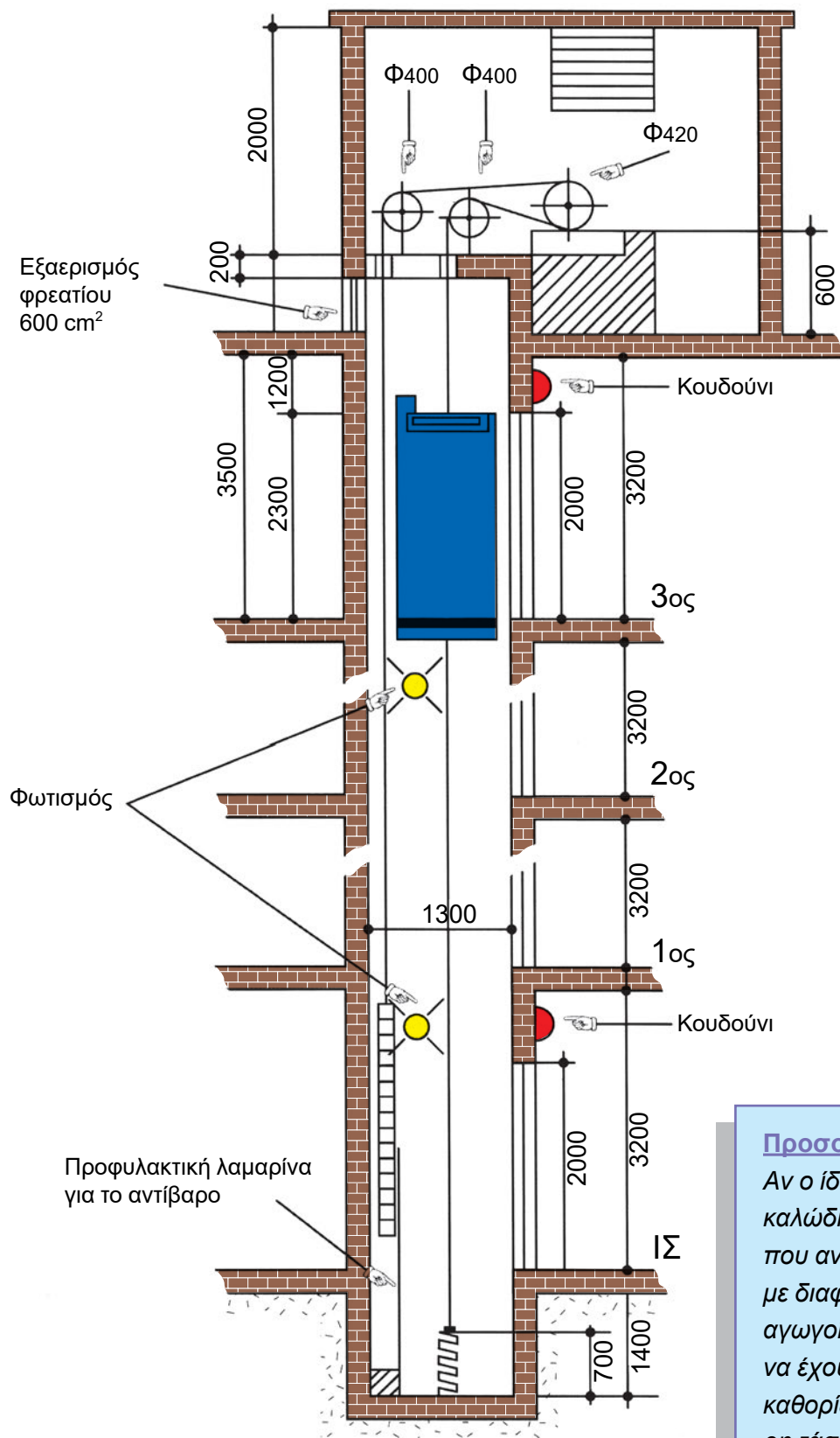
Τομή σε όλο το ύψος του φρεατίου
