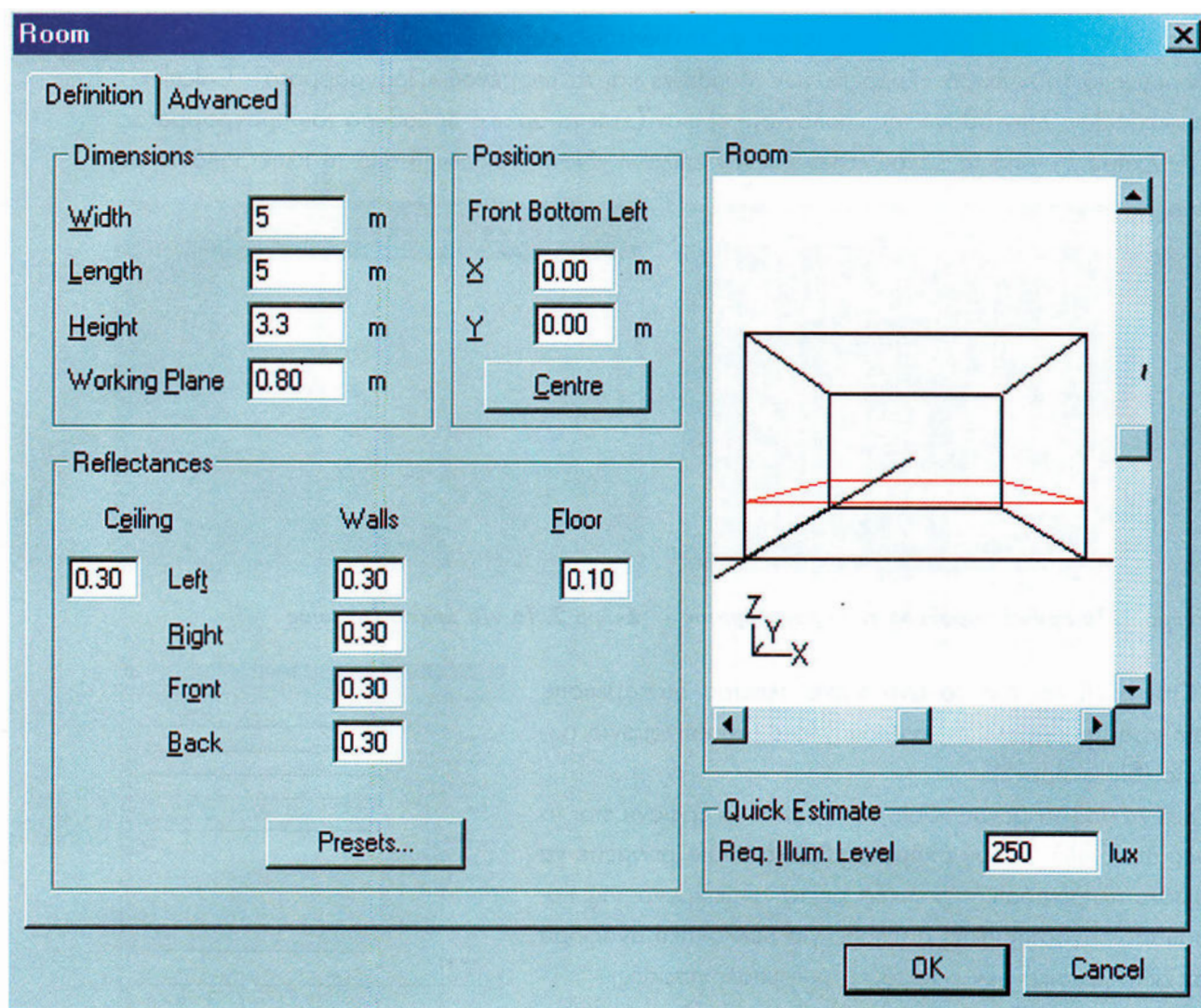
Σχήμα 5. Τα δεδομένα του χώρου, του επιπέδου εργασίας, οι συντελεστές ανάκλασης τοιχωμάτων και η επιθυμητή ένταση φωτισμού
