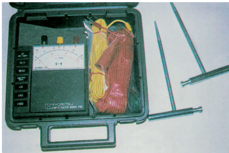
Όργανο μέτρησης της αντίστασης γείωσης
