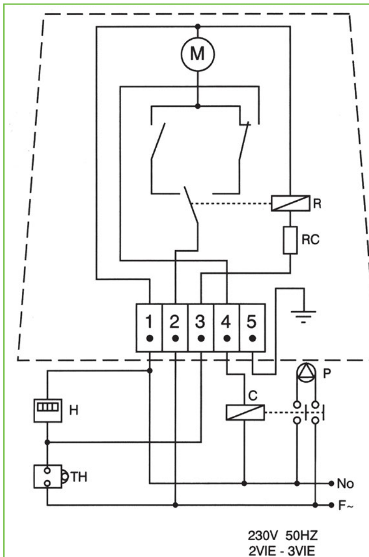
Συνδεσμολογία δίοδης ηλεκτροβάνας
