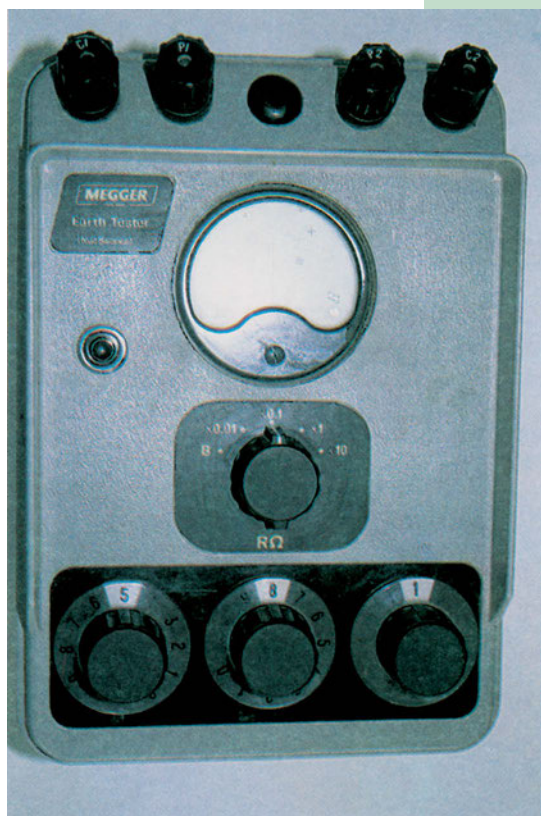
Εξωτερική όψη γειωσόμετρου
