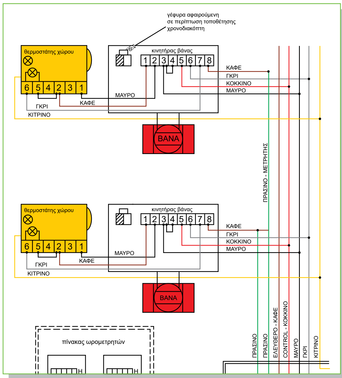
Κατασκευαστικό σχέδιο σύνδεσης βάνας και θερμοστάτη χώρου
