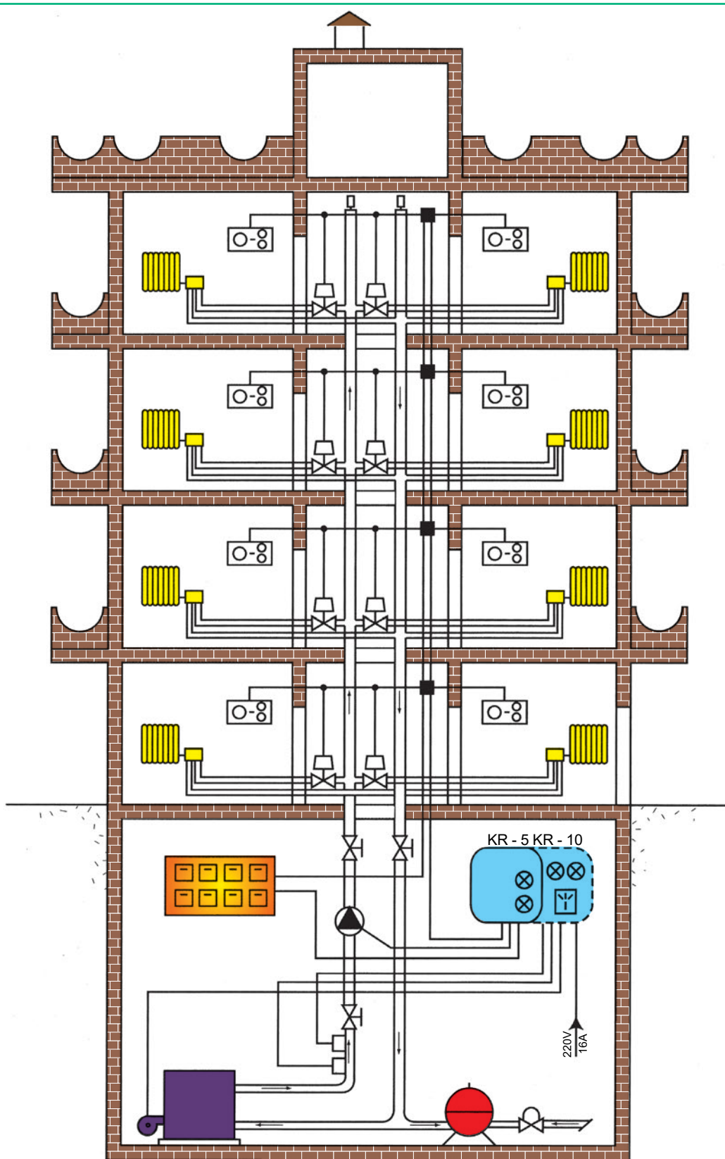
Κατακόρυφο διάγραμμα κεντρικής θέρμανσης και ηλεκτρικό διάγραμμα αυτόνομης λειτουργίας της
