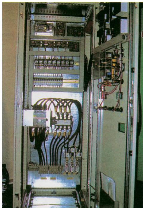
Βιομηχανικός πίνακας κίνησης
