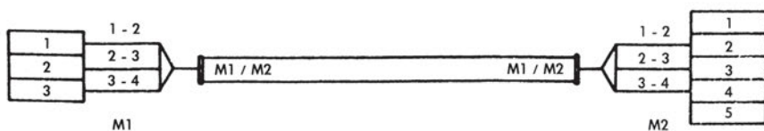
Κλεμοσειρά M1
