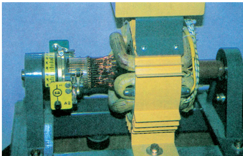
Γεννήτρια σύνθετης διέγερσης
