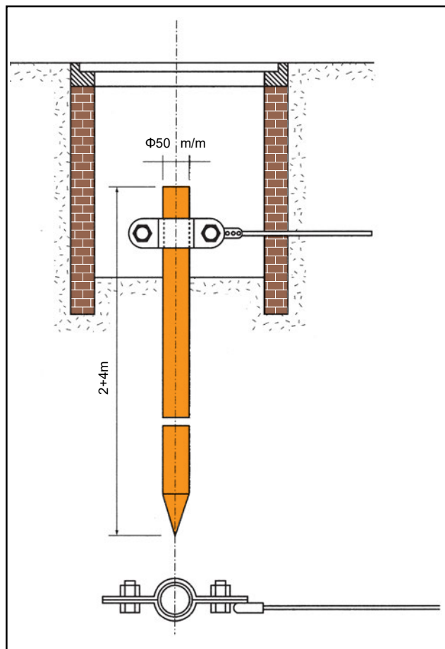
Ηλεκτρόδια γειώσεων
