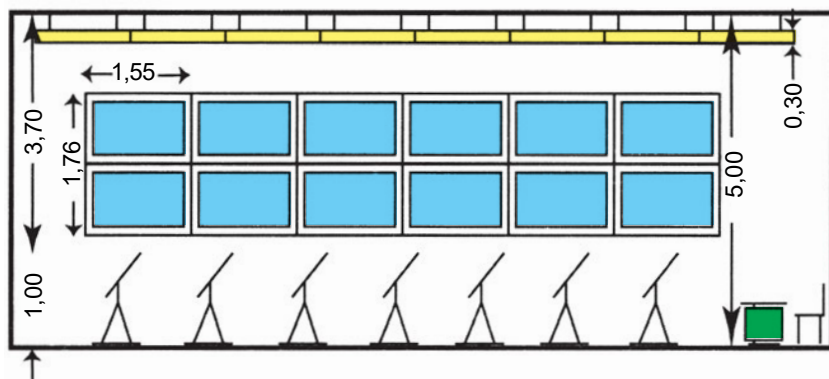
Τομή της αίθουσας σχεδίου
