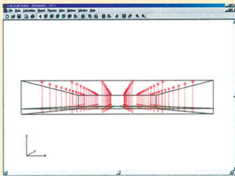
Σχήμα 2α. Τριδιάστατη απεικόνιση του χώρου με τη διάταξη των φωτιστικών σωμάτων και την επιφάνεια εργασίας
