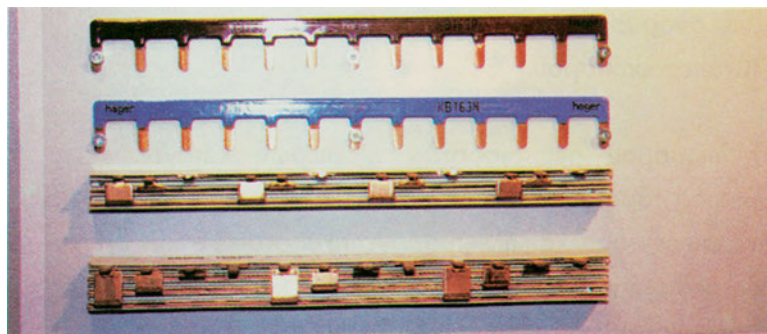
Περωνωτές μπάρες συνδέσεων
