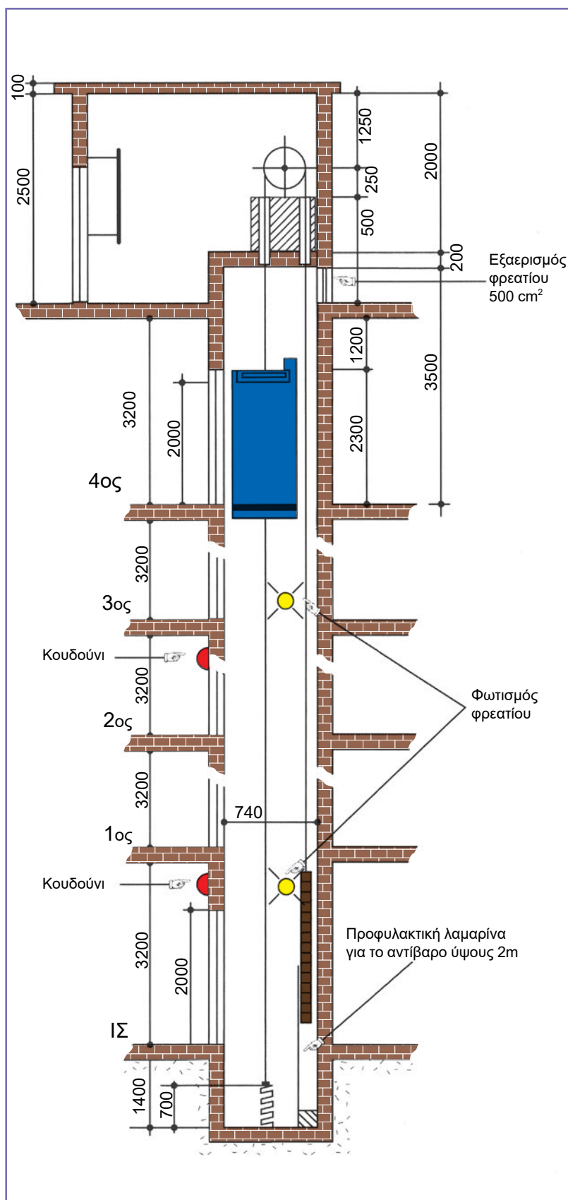
Τομή σε όλο το ύψος του φρεατίου
