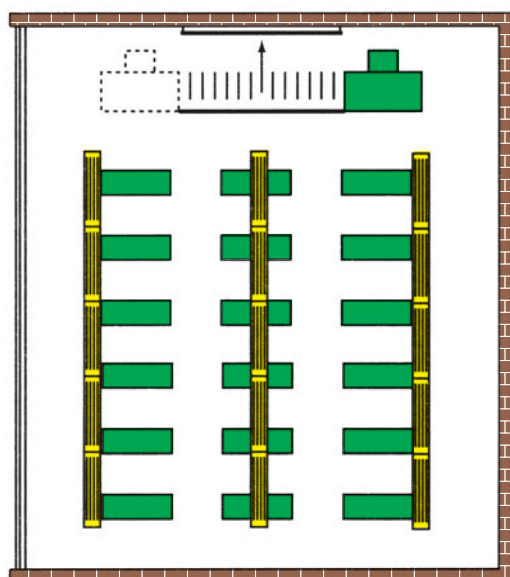
Παράδειγμα διάταξης των φωτιστικών σωμάτων για τον γενικό φωτισμό αίθουσας διδασκαλίας και τον τοπικό φωτισμό του μαυροπίνακα.
