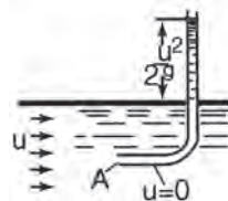
Σχήμα 16.8.δ Σωλήνας Pitot
