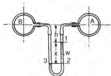
Σχήμα 15.8.5 Μέτρηση διαφοράς πίεσης μεταξύ δυο σωλήνων με διαφορικό μανόμετρο
