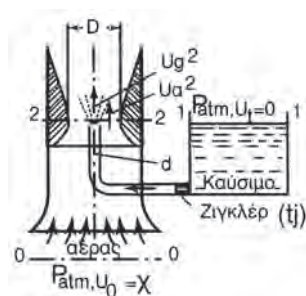
Σχήμα 16.8.β Εξαερωτής
