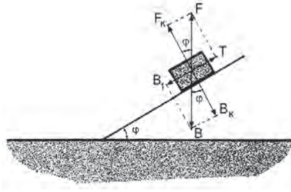
Σχήμα 14.4.β Σώμα ολισθαίνον σε κεκλιμένο επίπεδο
