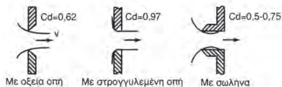
Σχήμα 16.6.β Οι τιμές του συντελεστή C_d , ανάλογα με το στόμιο εκροής.
