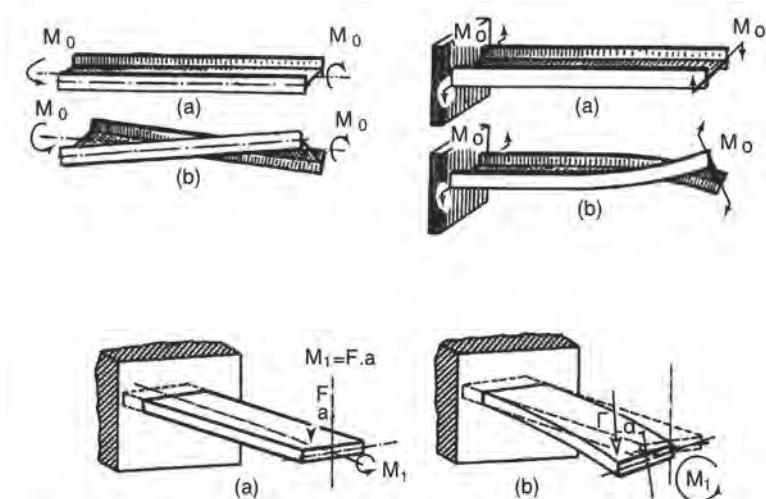
Σχήμα 11.4.β Παραμόρφωση φορέων υποκείμενων σε στρέψη, μη κυκλικής διατομής
