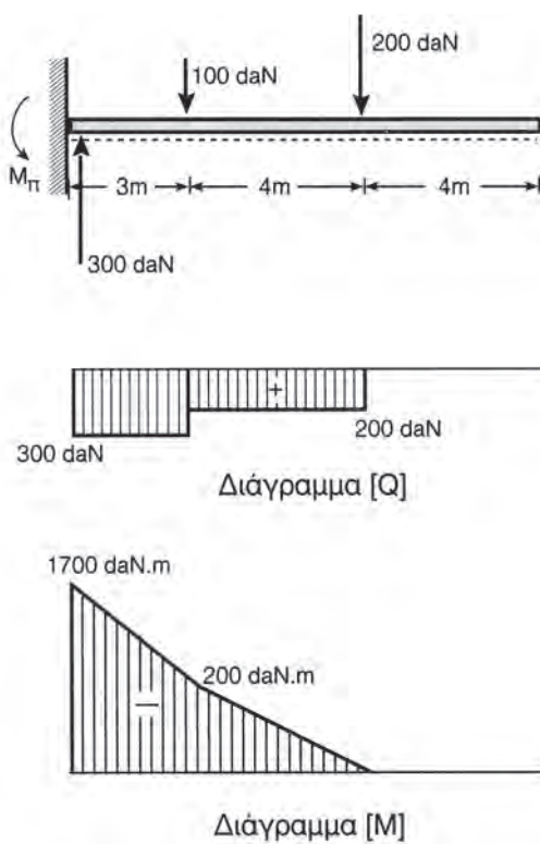
Σχήμα 8.6ξ
