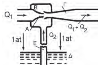
Σχήμα 16.8.γ Ψεκαστήρας
