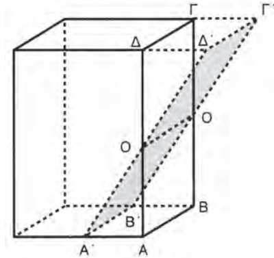
Σχήμα 10.1ζ Ο-Ο Ουδέτερος άξονας. Διατομή Α'Β'Γ'Δ' μιας καμπτόμενης δοκού
