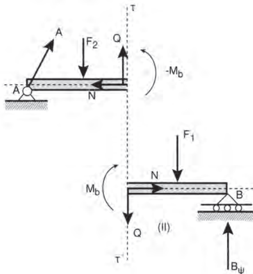
Σχήμα 8.5β Τομή τ - τ της δοκού
