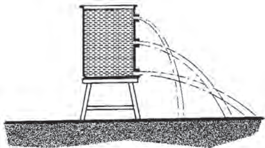
Σχήμα 15.4.β Πειραματική απόδειξη της αύξησης της υδροστατικής πίεσης μετά του βάθους
