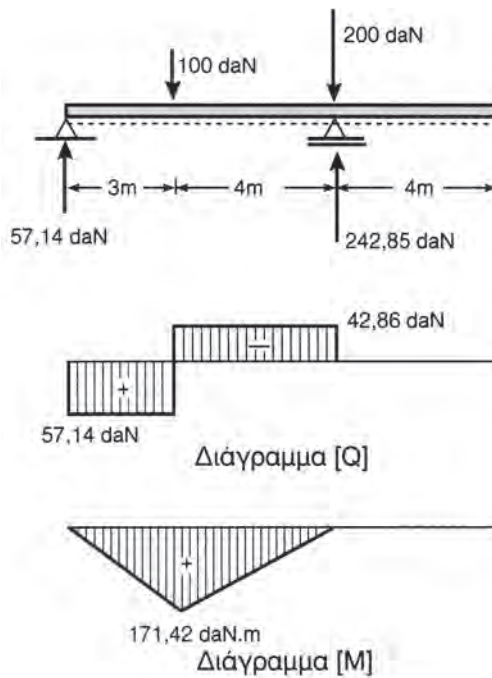
Σχήμα 8.6λ
