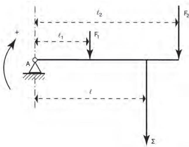
Σχήμα 2.2α Το θεώρημα των ροπών
