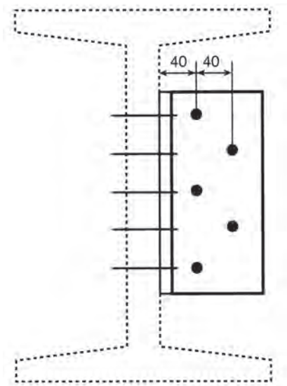
Καρφωτή σύνδεση
