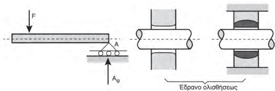
Σχήμα 8.2δ Κύλιση
