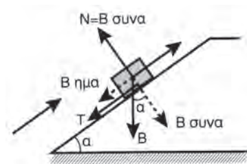
Σχήμα 13.5γ Φορτίο σε κεκλιμένο επίπεδο
