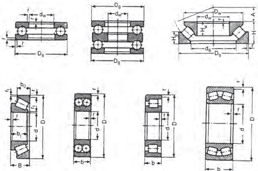
Σχήμα 14.6.4.α Διάφορα είδη ένσφαιρων τριβέων (τριβέας κύλισης)
