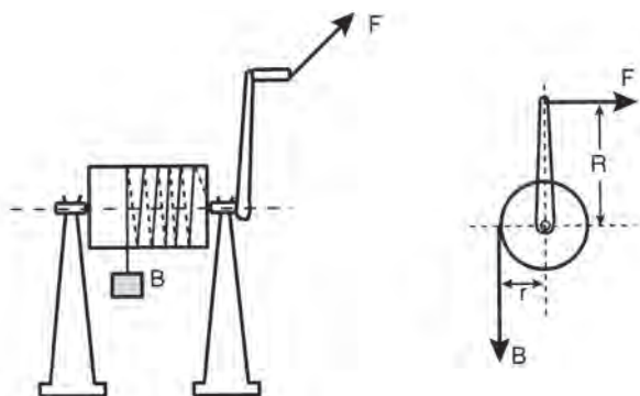
Σχήμα 13.4.3α Βαρούλκο
