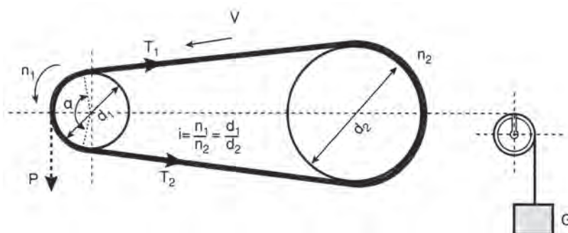
Σχήμα 13.7α Ιμαντοκίνηση
