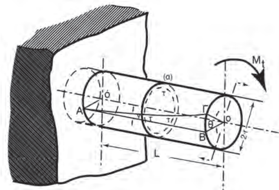
Σχήμα 11.2.α Η παραμόρφωση ράβδου κυκλικής διατομής καταπονούμενης σε στρέψη
