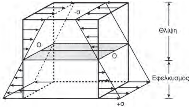
Σχήμα 8.5θ Κάμψη της διατομής της δοκού
