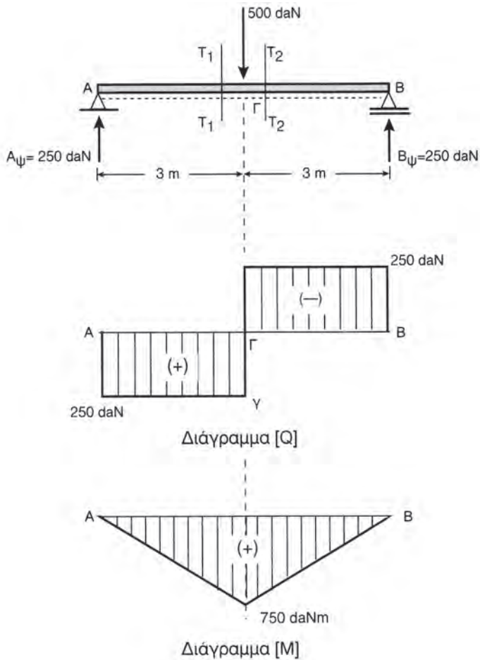
Σχήμα 8.6α Αμφιέρεστη δοκός
