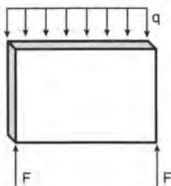
Σχήμα 8.1ε Δίσκος
