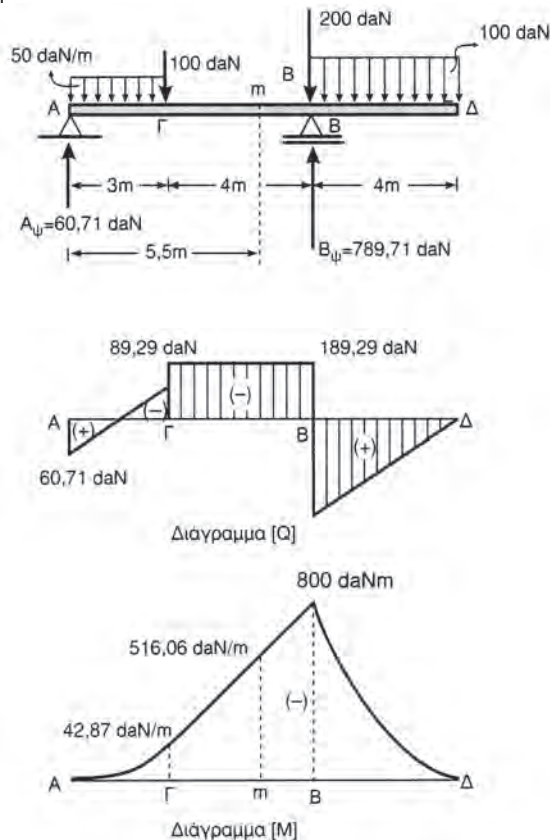
Σχήμα 8.6θ Μονοπροέχουσα δοκός
