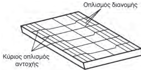
Σχήμα 10.4ε Τοποθέτηση χάλυβα σε πλάκα
