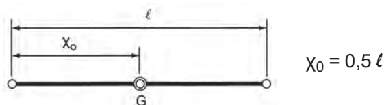
Σχήμα 4.2α Κεντροειδές γραμμής
