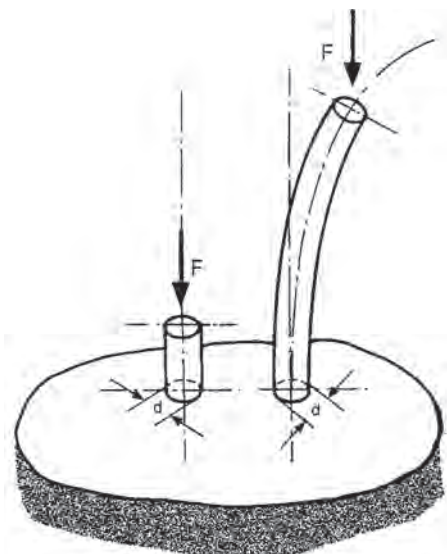
Σχήμα 12.3.1α Η διαφορά συμπεριφοράς στην καταπόνηση της θλίψης, εξαιτίας της διαφοράς ύψους του στοιχείου.
