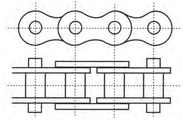
Σχήμα 13.7ζ Αλυσοκίνηση
