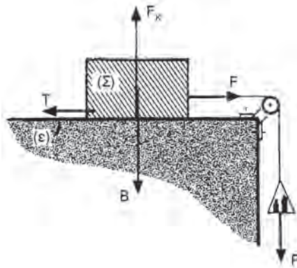
Σχήμα 14.4.α Σώμα ολισθαίνον σε οριζόντιο επίπεδο
