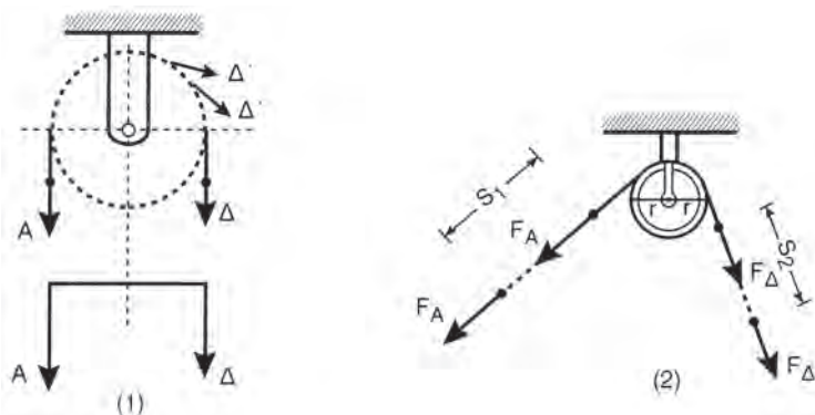
Σχήμα 13.4.2γ Τροχαλία
