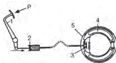
Σχήμα 15.9.2.α Υδραυλικό φρένο αυτοκινήτου
