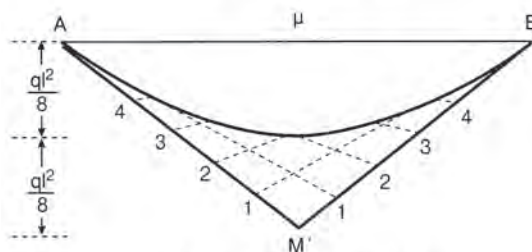
Σχήμα 8.60 Αμφιέριστη δοκός
