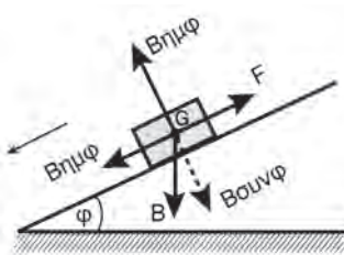
Σχήμα 13.2δ Το φορτίο κατέρχεται
