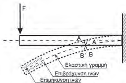
Σχήμα 10.1θ Ελαστική γραμμή – Βέλος κάμψης
