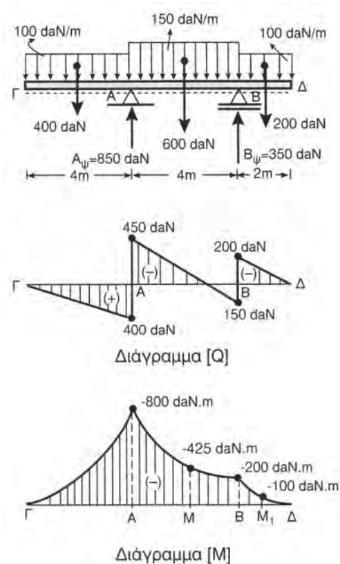
Σχήμα 8.6i Αμφιπρόεχουσα δοκός
