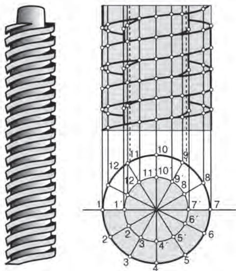
Σχήμα 13.6δ Τετραγωνικό σπείρωμα
