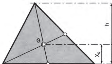
Σχήμα 4.3δ Κεντροειδές επιφάνειας τριγώνου
