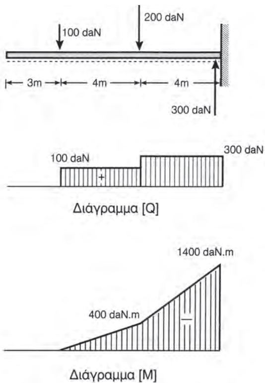
Σχήμα 8.6ο
