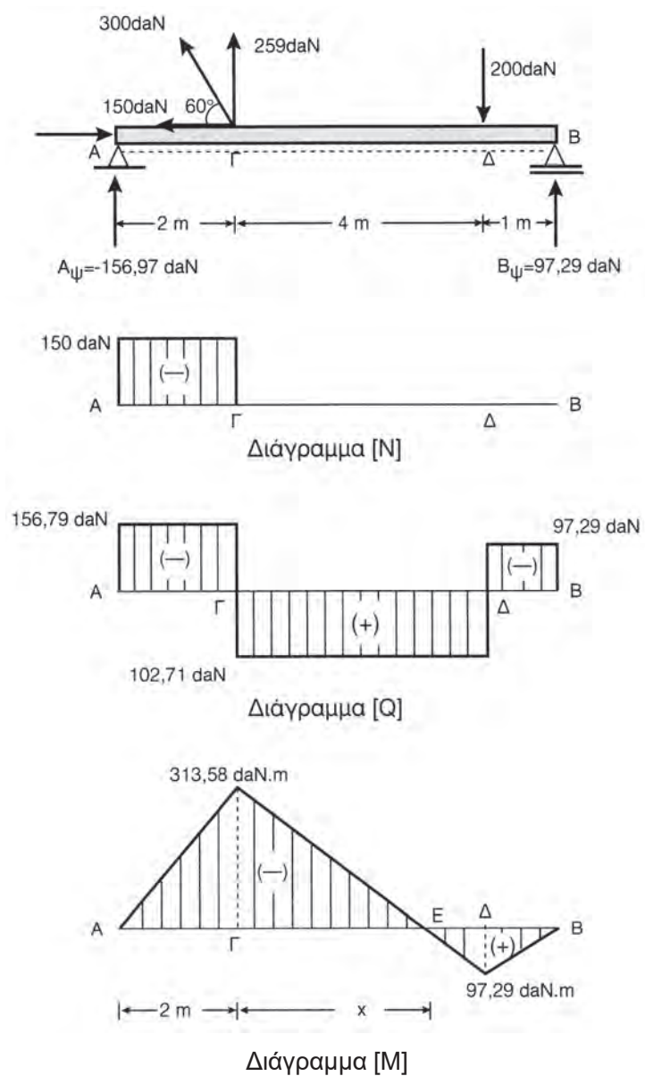
Σχήμα 8.6ε Αμφιέρειστη δοκός
