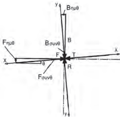
Σχήμα 14.6.3.γ Η ανάλυση των δυνάμεων που ενεργούν στο σπείρωμα κοχλία, σε ορθογώνιο σύστημα x, x' - y, y' .
