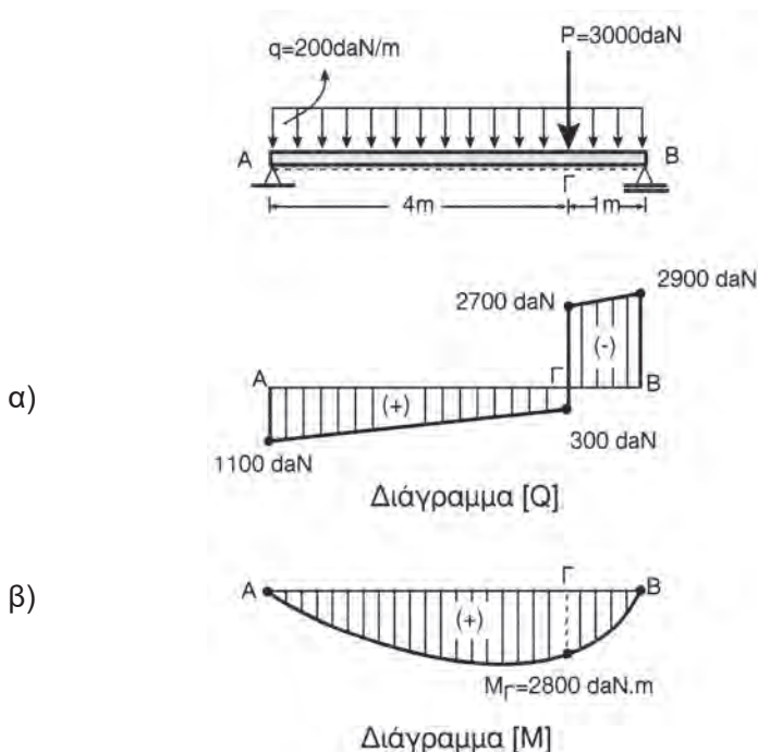
Σχήμα 10.4η Αμφιέρειστη δοκός καταπονούμενη σε κάμψη
