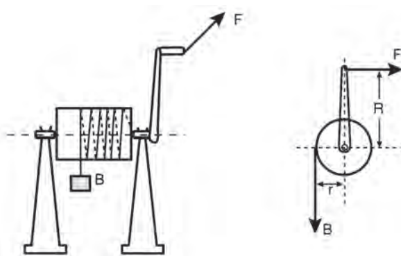
Σχήμα 13.2στ Το έργο στην περιστροφική κίνηση
