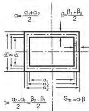
Σχήμα 11.5.γ Ορθογωνική σωληνωτή διατομή (στραντζαριστό)
