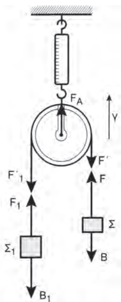
Σχήμα 13.4.2α Τροχαλία
