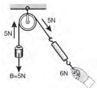
Σχήμα 13.4.2β Τροχαλία
