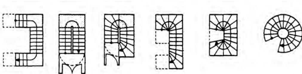
Εικ. 172 Διάφορες μορφές σκάλας.
