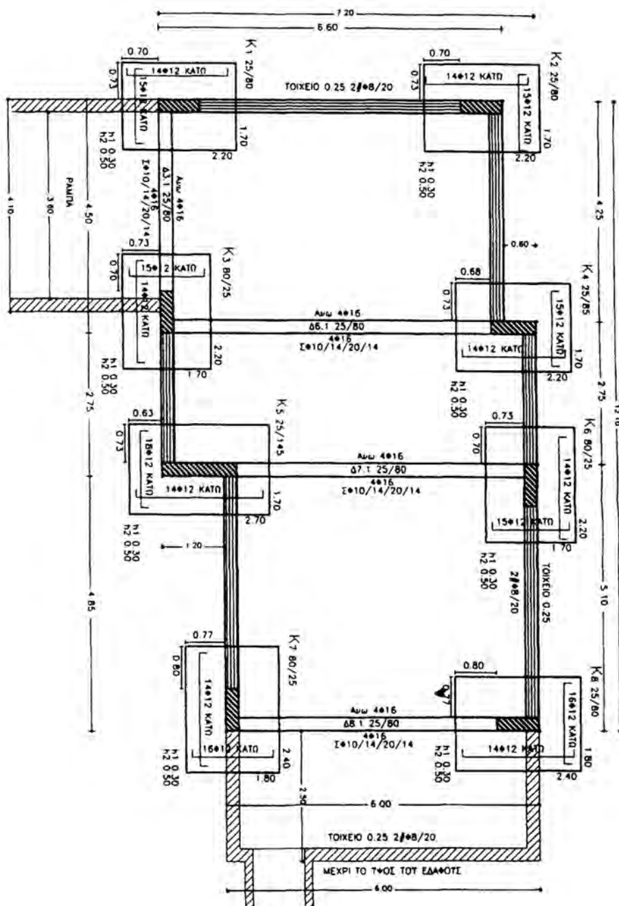
Εικ. 159 Ξυλότυπος θεμελίων.
