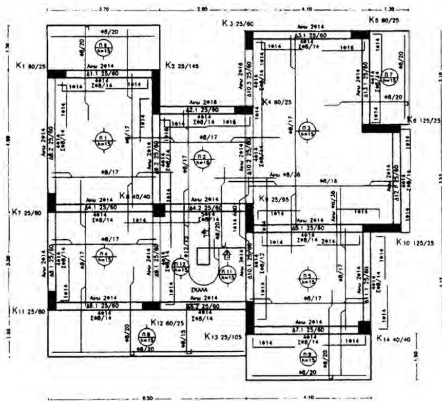
ΞΥΛΟΤΥΠΟΣ ΙΣΟΓΕΙΟΥ
