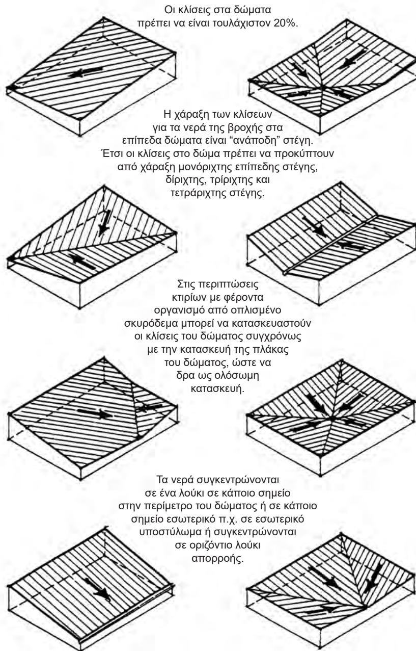
Εικ. 218 Κλίσεις απορροής των ομβρίων.
