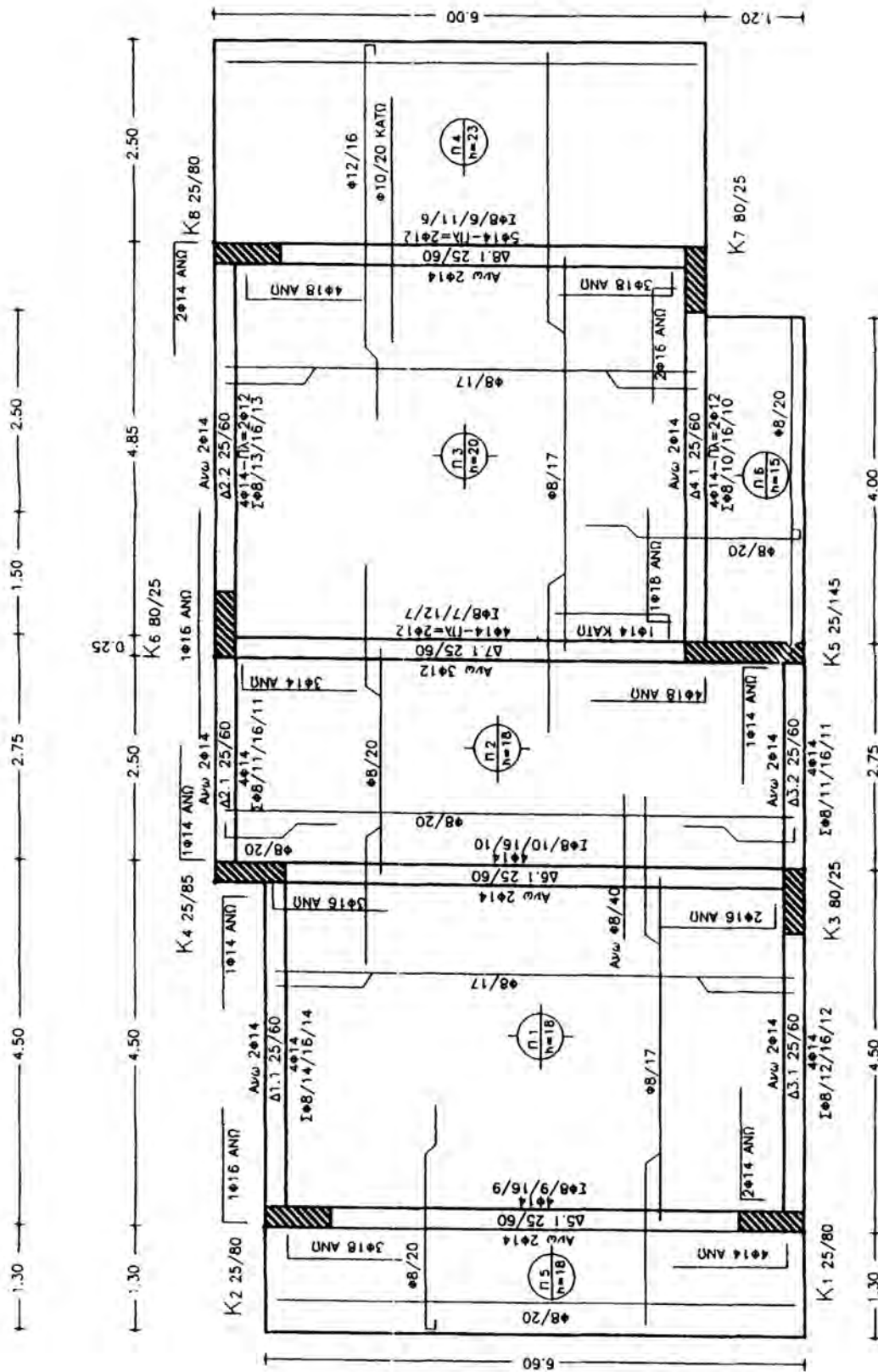
Εικ. 142 Ευλόγυτος πλάκας.
