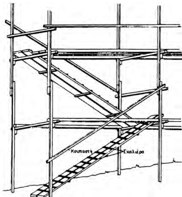
Εικ. 123 Διαμόρφωση κεκλιμένου επιπέδου (ξυλίνης ράμπας) για την κίνηση των εργαζομένων στην οικοδομή.
