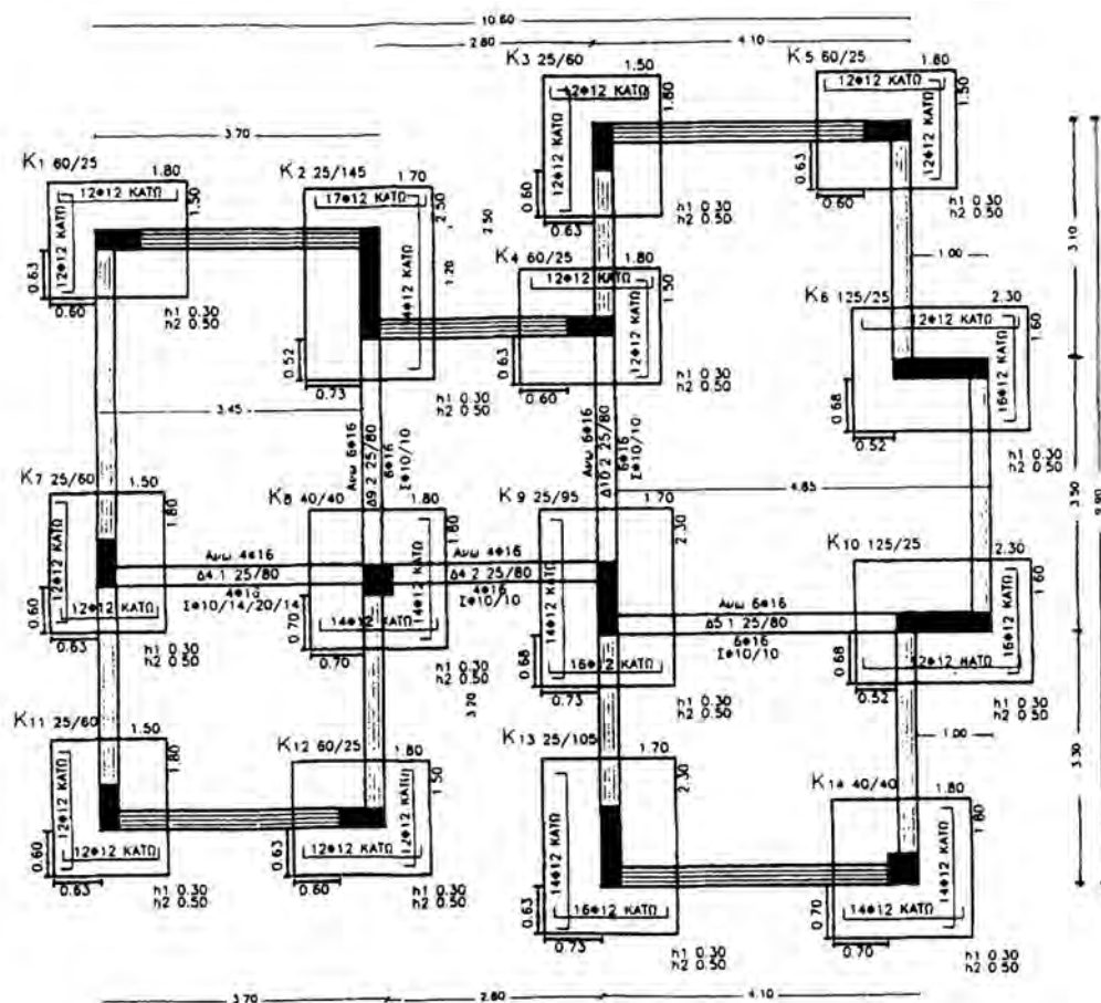
Εικ. 161 Θεμελίωση.
