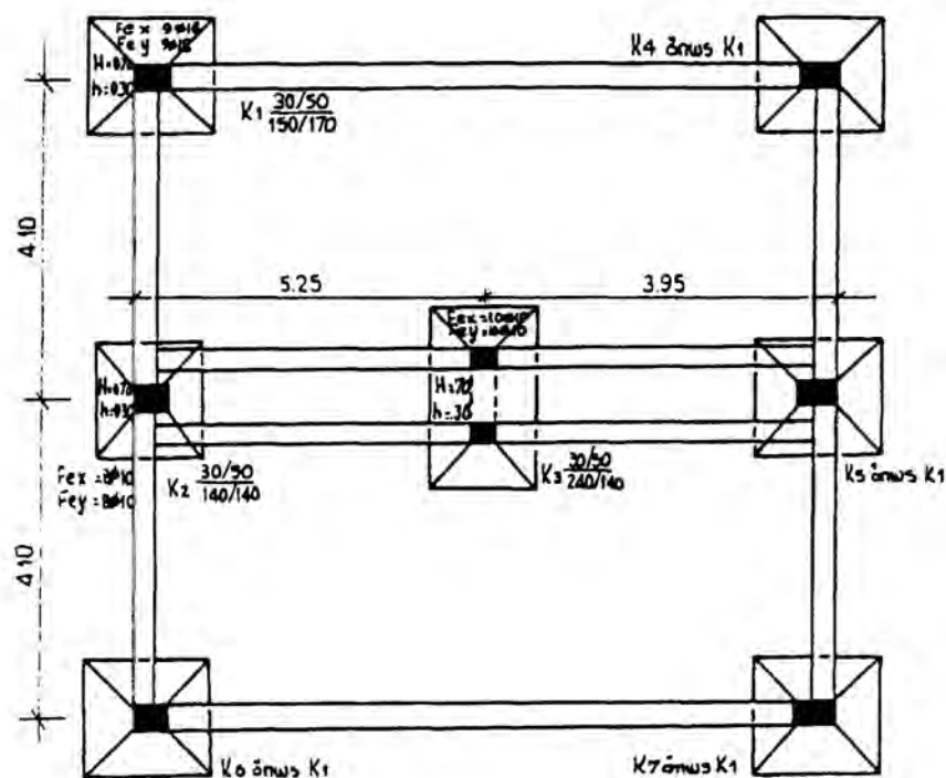
Εικ. 157 Θεμελίωση.
