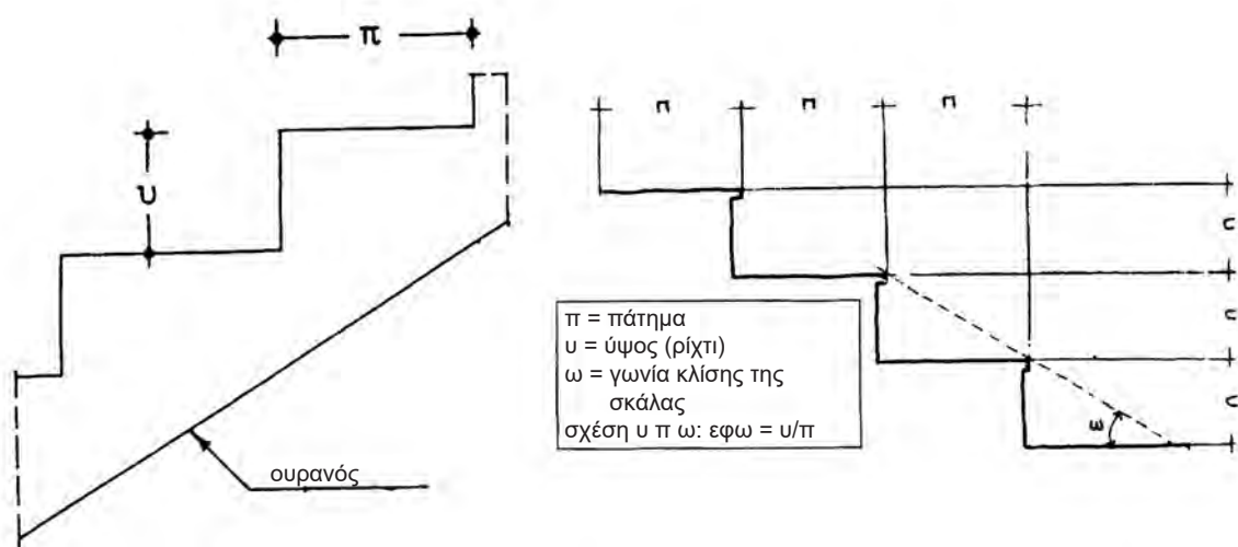
Εικ. 165 Τα βασικά στοιχεία μιας σκάλας.
