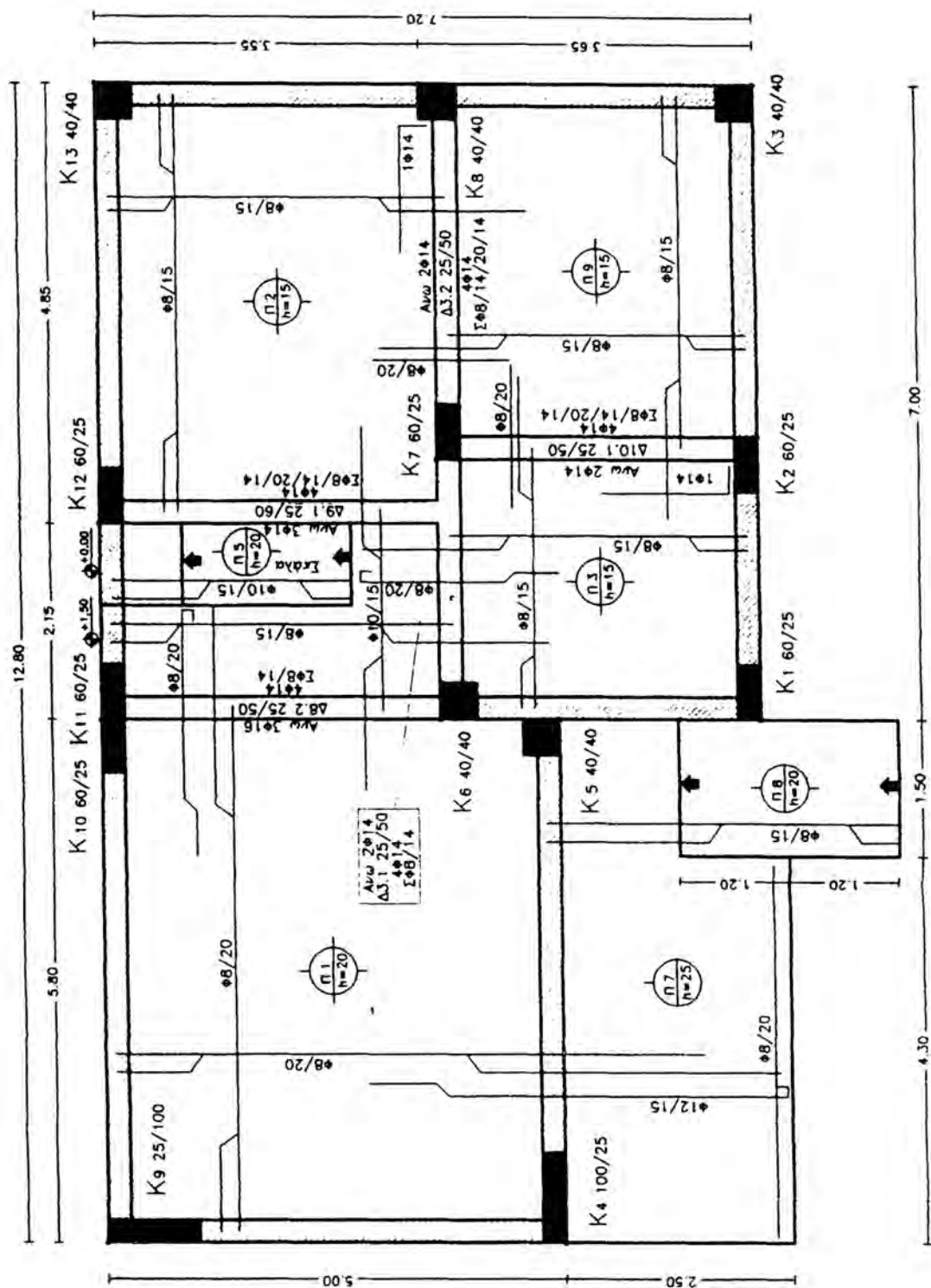
Εικ. 141 Ευλότυπος πλάκας.
