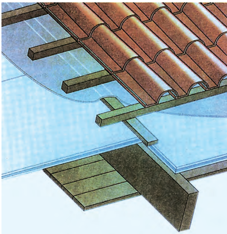
Εικ. 233 Μόνωση ξύλινης στέγης (α).
