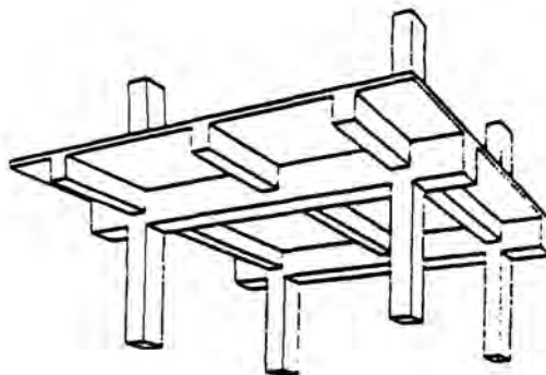
Εικ. 128 Τετραέρευση πλάκα.
