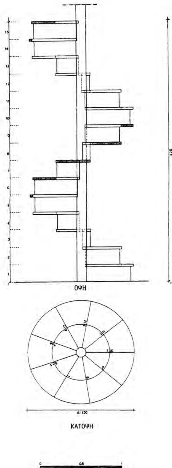
Εικ. 192 Κάτοψη και τομή κυκλικής σκάλας.
