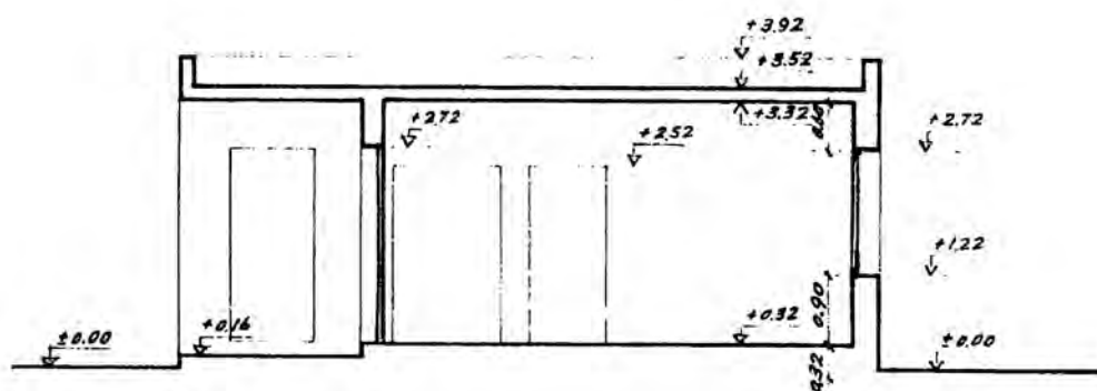
ΤΟΜΗ Γ-Γ
