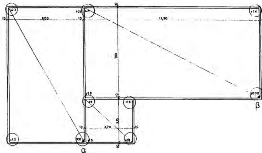
Εικ.215 Αποχέτευση δωματίων - συμβολισμός υψομέτρων.
