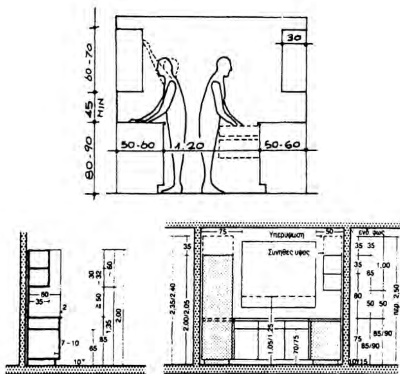
Εικ. 52 Κατακόρυφη τομή στην κουζίνα - εξοπλισμός.
