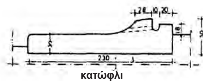
κατώφλι
