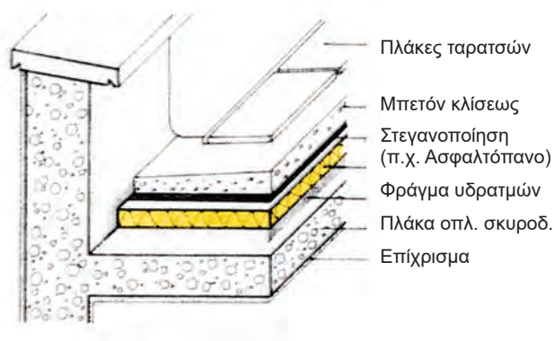
Εικ. 225 Στηθαία δωμάτων.
