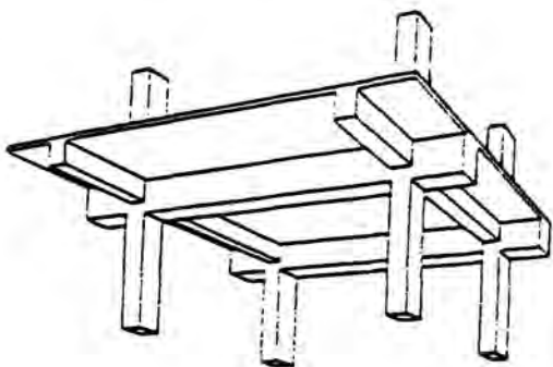
Εικ. 127 Διέρευση πλάκα με εγκάρσια δοκίδια, ανάμεσα στα υποστυλώματα.
