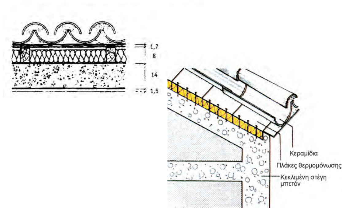
Εικ. 237 Μόνωση στέγης από οπλισμένο σκυρόδεμα.
