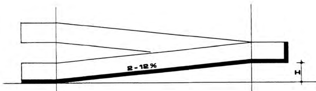
Εικ. 173 Ράμπα.
