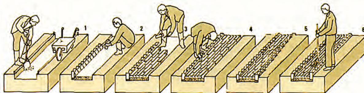
Φωτ. 5-30: Διάστρωση διαδρόμου από τούβλο
