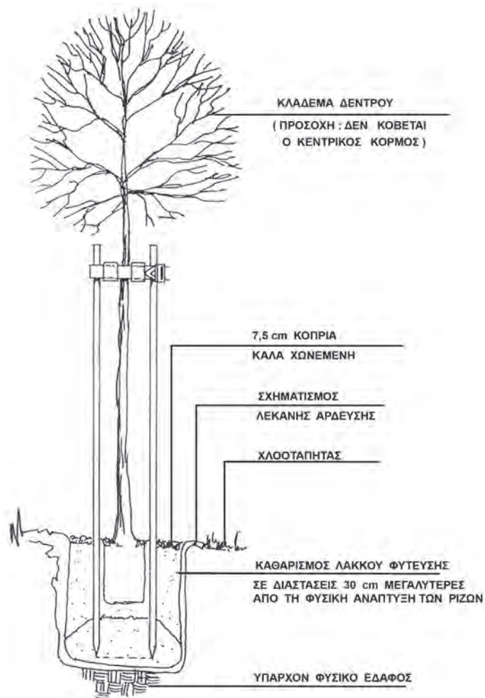
Φωτ. 5-19 και 5-20: Τρόπος δεσίματος δέντρου στο υποστήλωμα (λεπτομέρεια από Γραφείο Χ. Ροΐδη)
