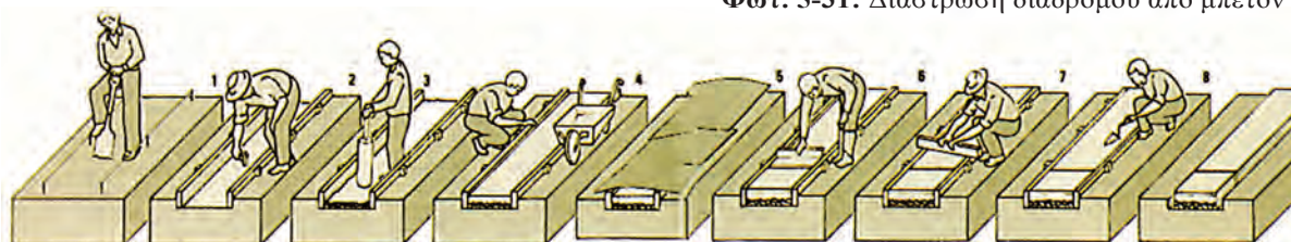
Φωτ. 5-31: Διάστρωση διαδρόμου από μπετόν
