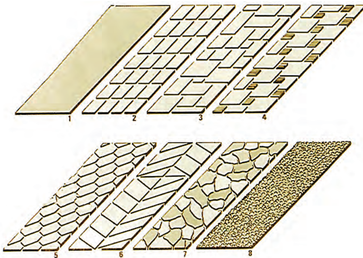
Φωτ. 5-36: Διάφορα μοτίβα (pattern) πλακόστρωσης. Σημασία έχει να διακρίνει κανείς τον τρόπο που συνδυάζονται τα υλικά μεταξύ τους
