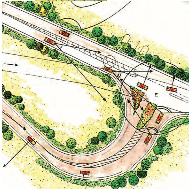
Σχήμα 7-2 και 7-3: Σχεδιασμός φύτευσης συγκοινωνιακών κόμβων. Θέες κατά την κίνηση των οχημάτων είναι ελεύθερες χωρίς φύτευση για τον πλήρη έλεγχο του πεδίου οδήγησης (Πηγή: Αρχείο Σ. Σεκλιζιώτη).
