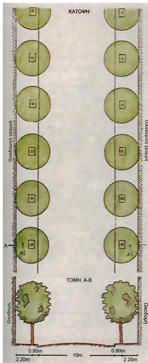
Σχέδιο 6-9: Τυπικό σχέδιο απεικόνισης δενδροστοιχίας
