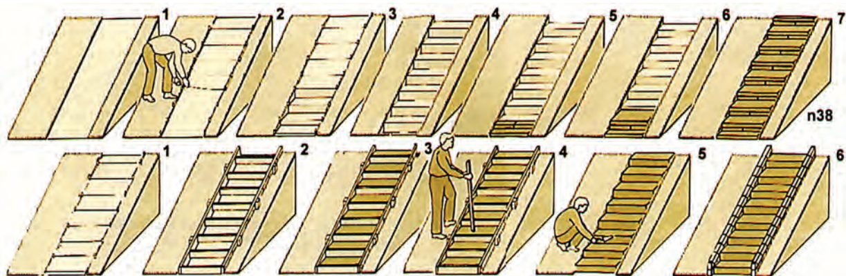
Φωτ. 5-41: Τεχνική κατασκευής σκάλας επί κεκλιμένου εδάφους. Η πορεία της εργασίας των σχημάτων περιγράφεται πάνω και κάτω από την φωτογραφία
