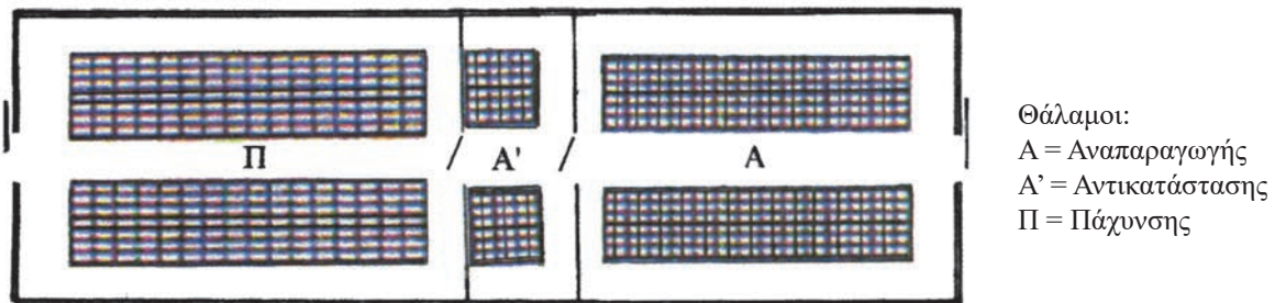
Εικ. 14.18 Κάτοψη κονικλοτροφείου με τρεις θαλάμους
