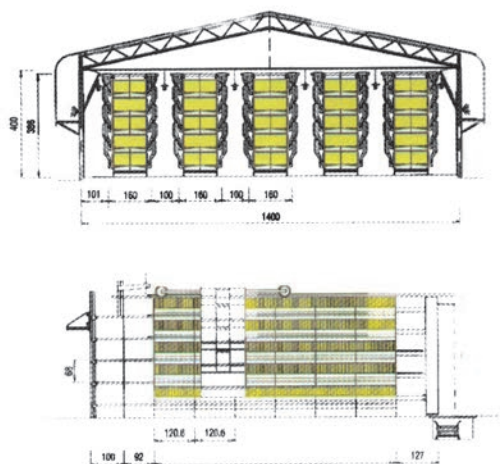
Εικ. 10.15 Τομή (επάνω) και κάτοψη (κάτω) θαλάμου εκτροφής ορνίθων αβγοπαραγωγής με πέντε σειρές κλωβών. Διακρίνονται οι διαστάσεις.
