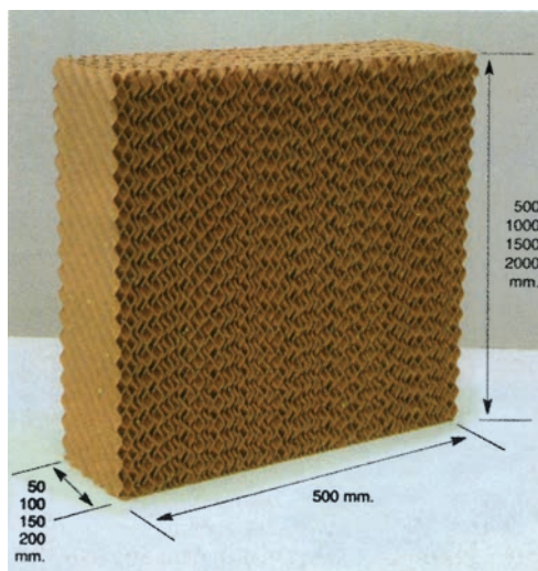
Εικ 4.13 Χάρτινο διαβρεχόμενο πάνελ δροσισμού
